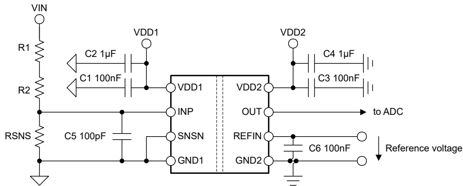
图 9-1. AMC0x11S-Q1 去耦
