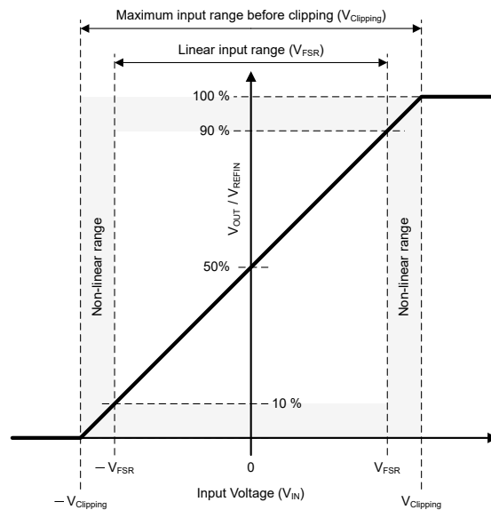
图 7-2. AMC0x30R-Q1 的输入到输出传递曲线
