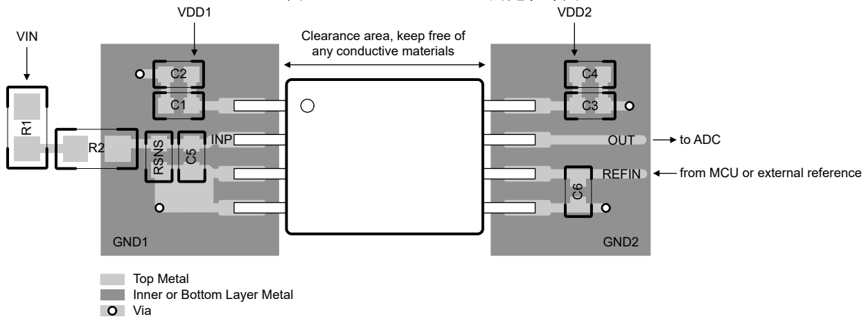
图 10-1. AMC0x30R-Q1 的建议布局
