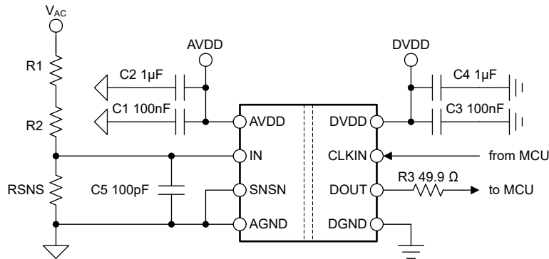
图 8-4. AMC0x36-Q1 去耦
