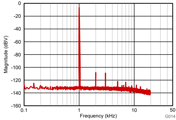
图 6-42. 1kHz 输入信号时的频谱
