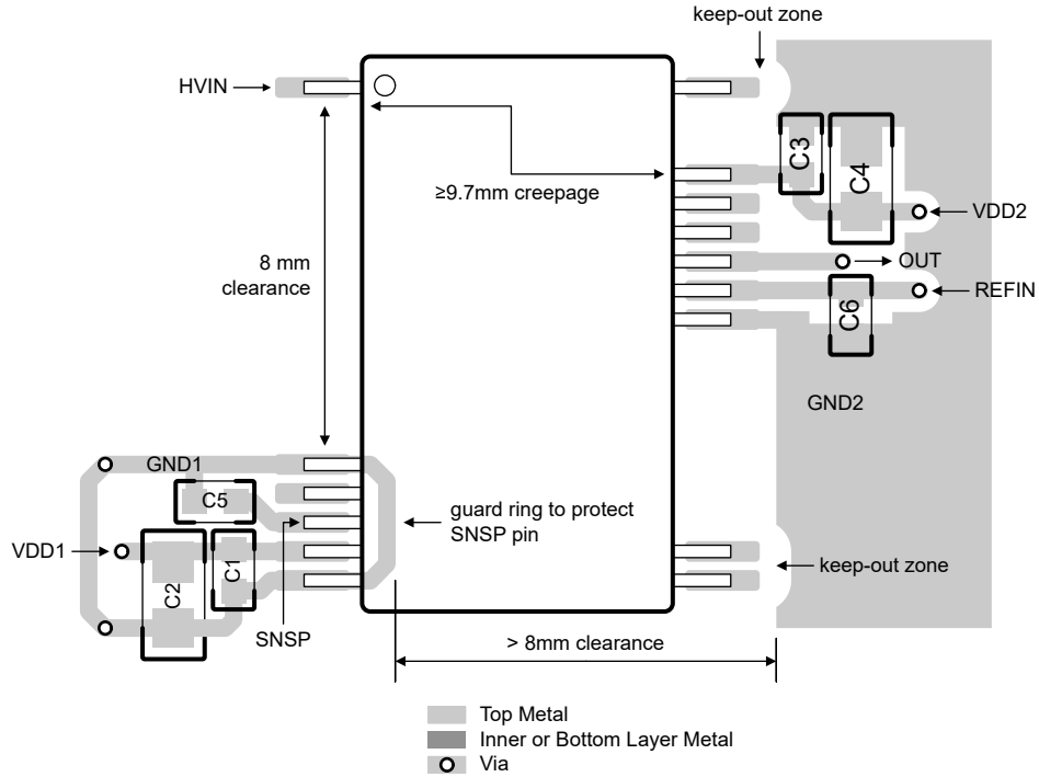
图 8-6. AMC0380R 的建议布局
