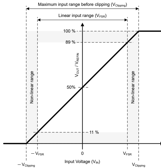
图 7-2. AMC0380R 的输入到输出传送曲线
