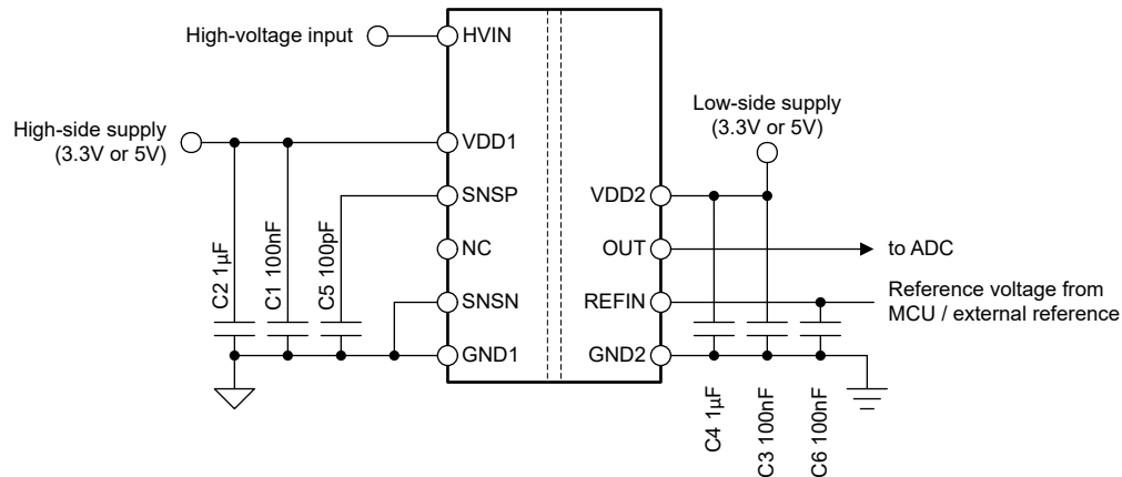
图 8-5. AMC0380R 去耦
