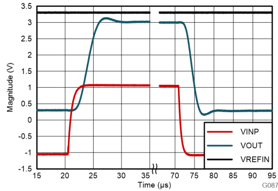
图 8-4. AMC0380R 的阶跃响应
