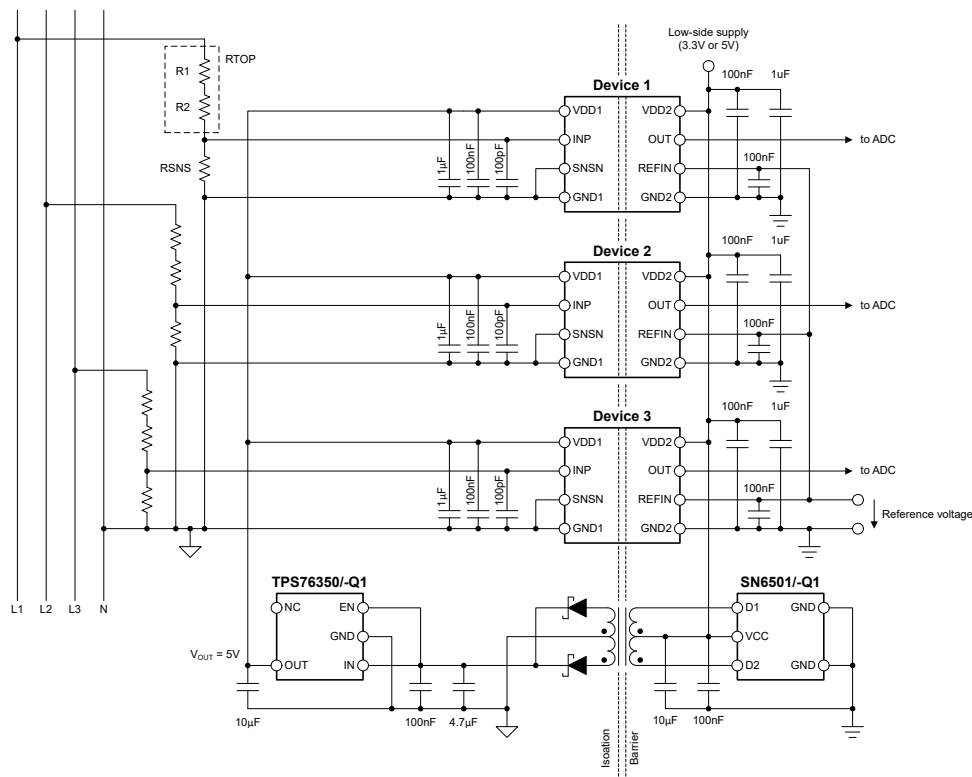
图 8-1. 在典型应用中使用 AMC0380R
