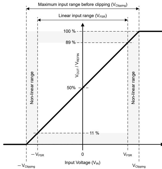
图 7-2. AMC0380R-Q1 的输入到输出传送曲线
