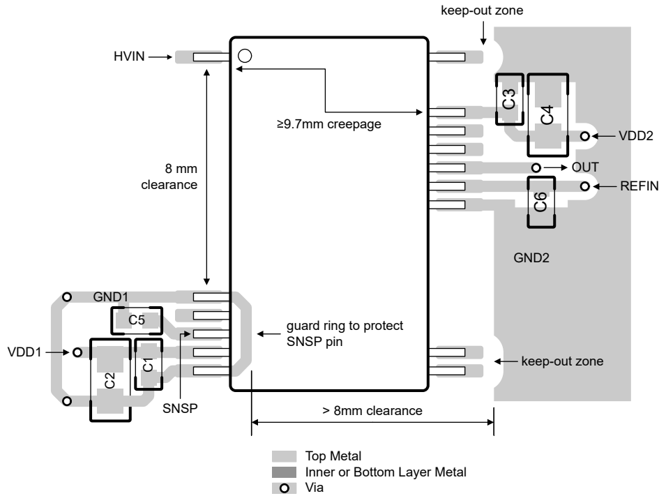
图 8-6. AMC0380R-Q1 的建议布局
