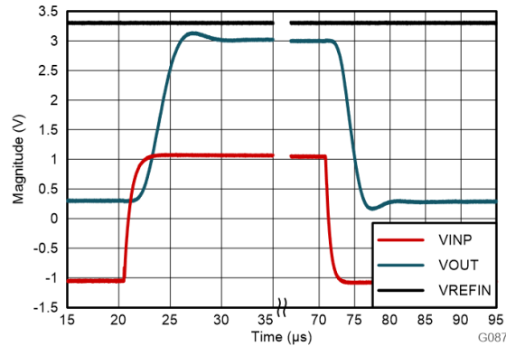
图 8-4. AMC0380R-Q1 的阶跃响应
