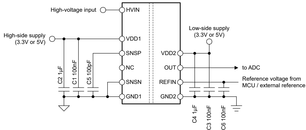
图 8-5. AMC0380R-Q1 去耦
