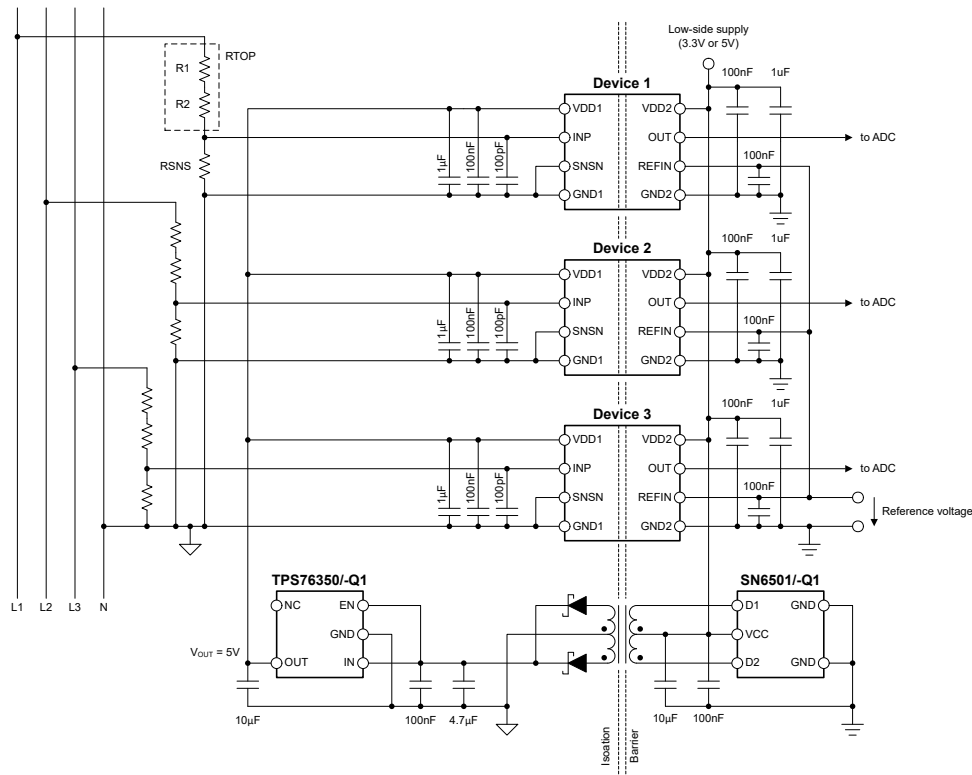
图 8-1. 在典型应用中使用 AMC0380R-Q1
