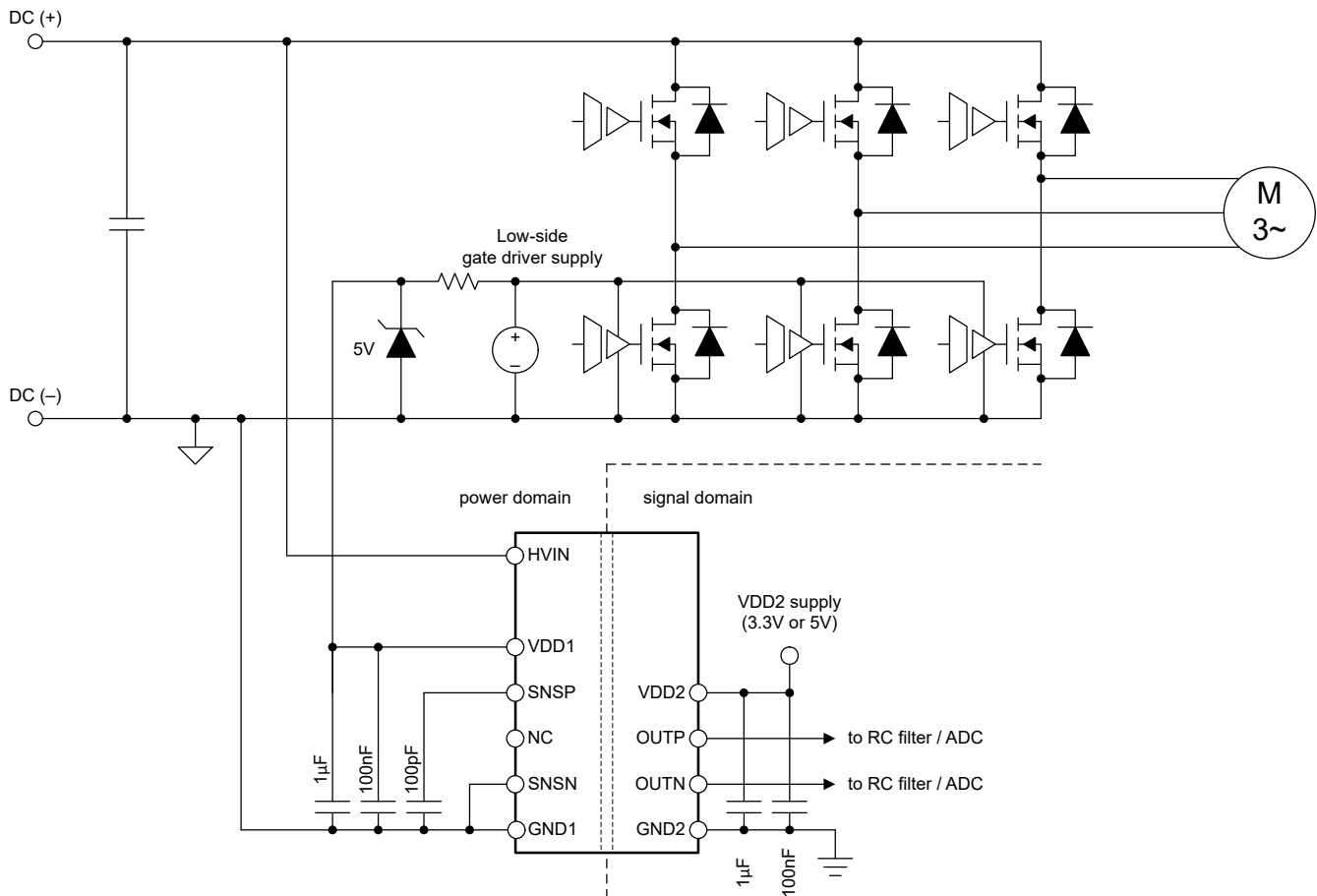
图 8-1. 在典型应用中使用 AMC0381D
