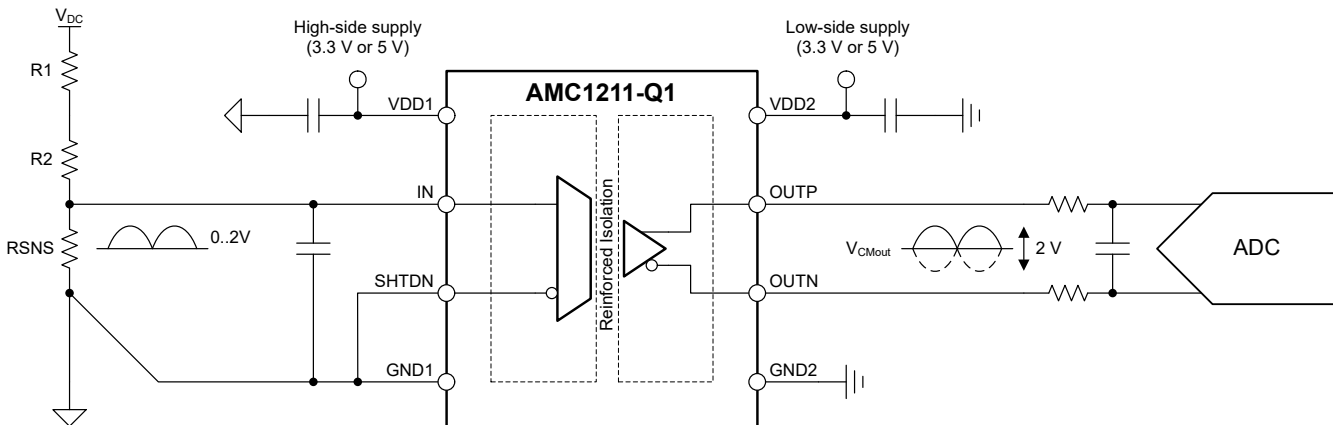
简化原理图
