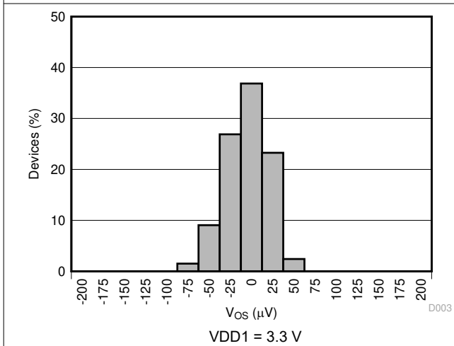
图 6-7. Input Offset Voltage Histogram
