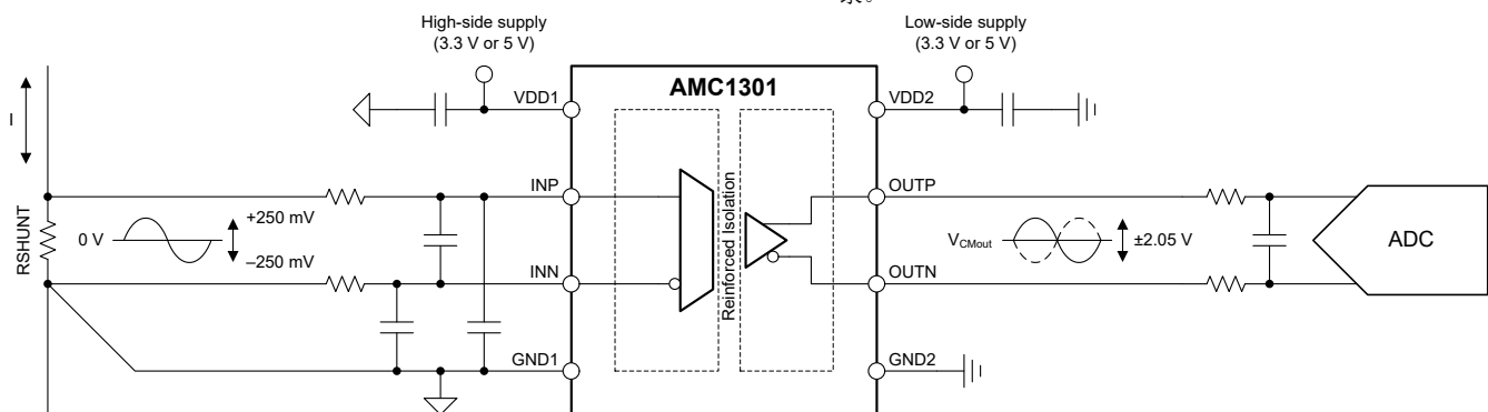
简化原理图
