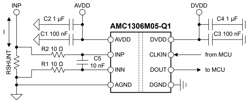
图 9-1. Decoupling of the AMC1306M05-Q1
