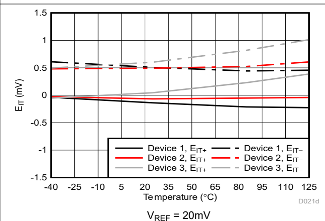
图 5-9. 跳变阈值误差与温度间的关系
