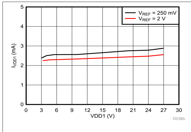
图 5-30. 高侧电源电流与电源电压间的关系
