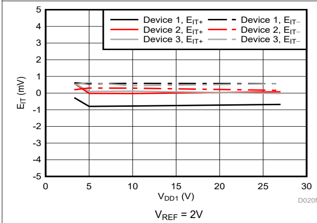
图 5-20. 跳变阈值误差与电源电压间的关系
