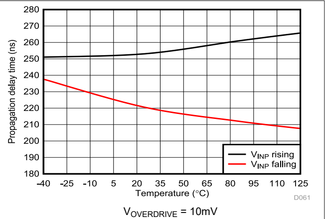
图 5-25. 传播延迟与温度间的关系
