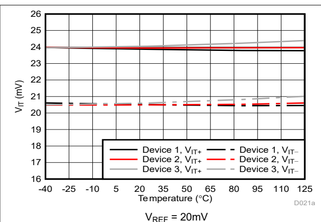
图 5-7. 跳变阈值与温度间的关系
