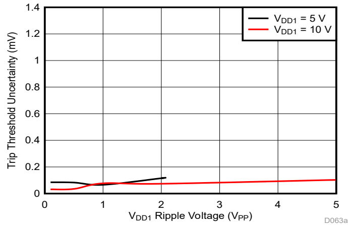
图 7-3. 跳变阈值对 VDD1 纹波电压的灵敏度 ( f_{RIPPLE} = 10\text{kHz} )
