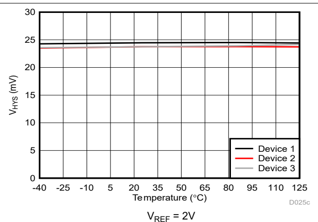
图 5-23. 跳变阈值迟滞与温度间的关系
