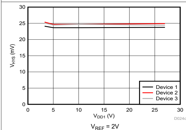
图 5-22. 跳变阈值迟滞与电源电压间的关系
