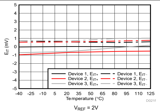
图 5-21. 跳变阈值误差与温度间的关系
