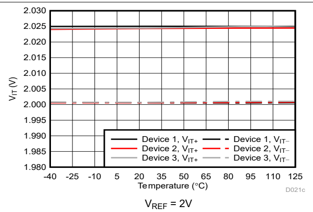
图 5-19. 跳变阈值与温度间的关系
