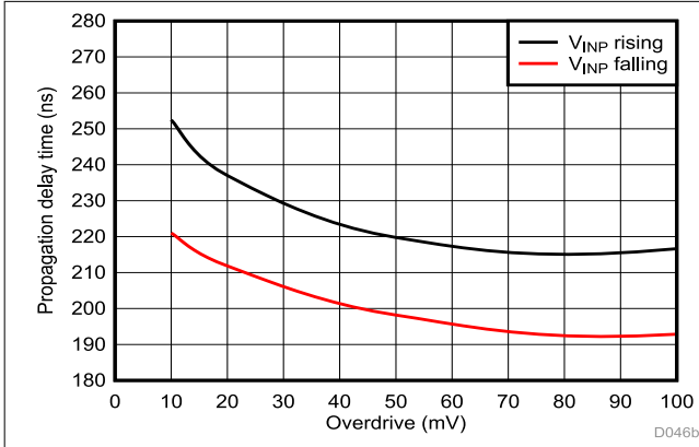
图 5-24. 传播延迟与过驱间的关系
