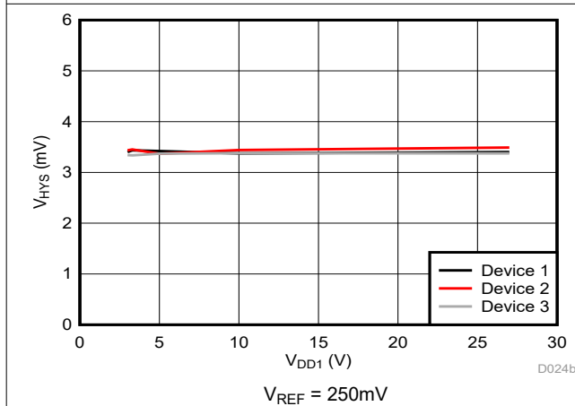
图 5-16. 跳变阈值迟滞与电源电压间的关系
