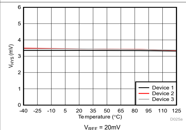
图 5-11. 跳变阈值迟滞与温度间的关系
