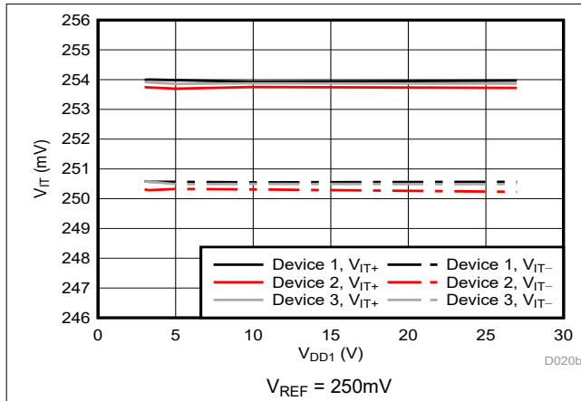
图 5-12. 跳变阈值与电源电压间的关系
