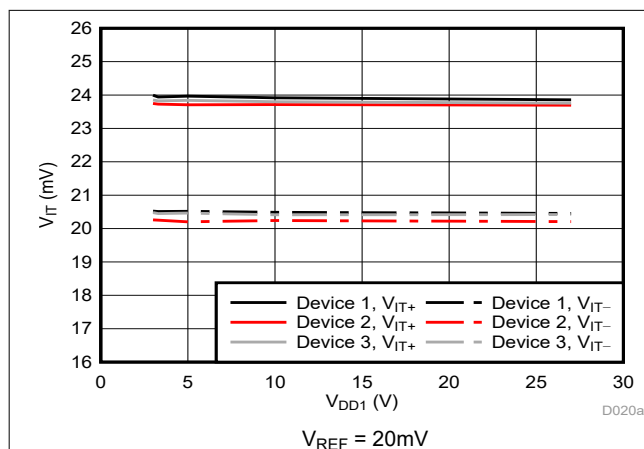
图 5-6. 跳变阈值与电源电压间的关系
