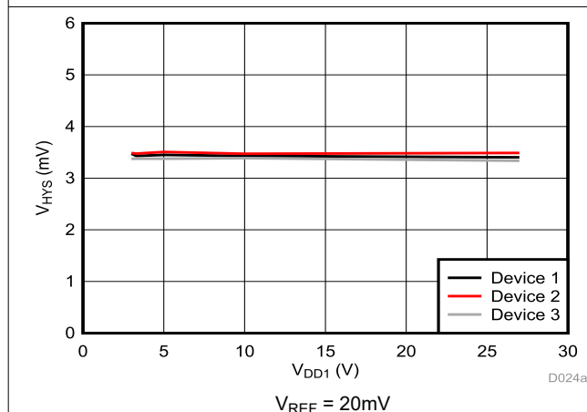
图 5-10. 跳变阈值迟滞与电源电压间的关系
