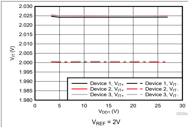
图 5-18. 跳变阈值与电源电压间的关系
