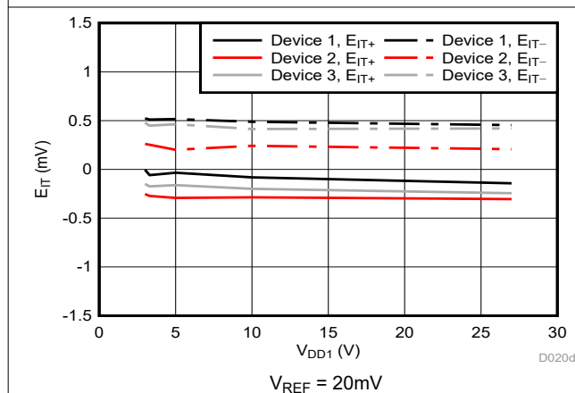
图 5-8. 跳变阈值误差与电源电压间的关系
