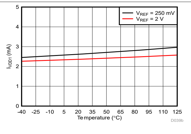
图 5-31. 高侧电源电流与温度间的关系
