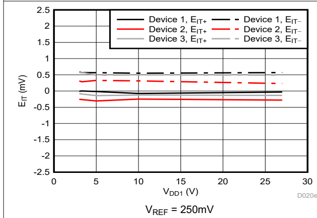
图 5-14. 跳变阈值误差与电源电压间的关系
