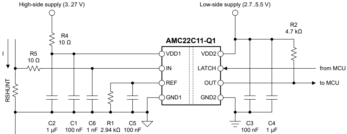
图 7-4. AMC22C11-Q1 去耦
