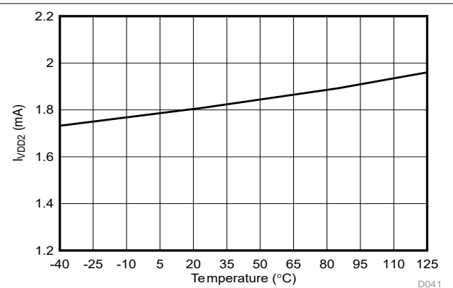
图 5-31. 高侧电源电流与温度间的关系
