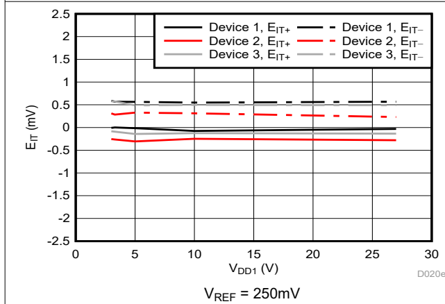
图 5-14. 跳变阈值误差与电源电压间的关系
