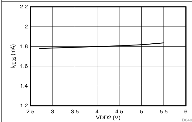
图 5-30. 高侧电源电流与电源电压间的关系
