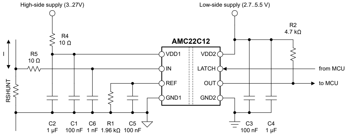
图 7-6. AMC22C12 去耦
