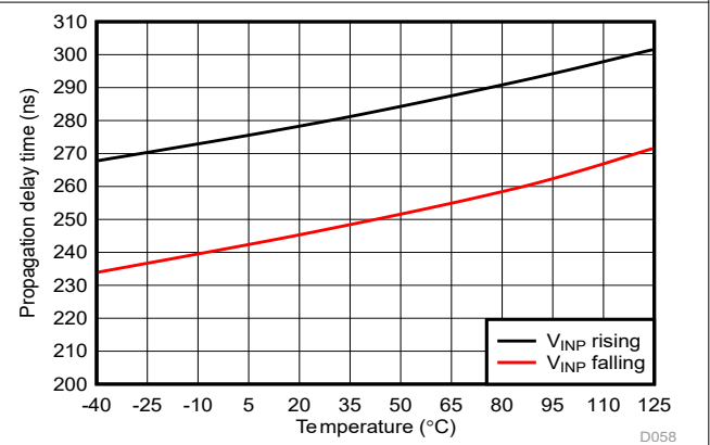
图 5-37. Cmp0 传播延迟与温度间的关系
