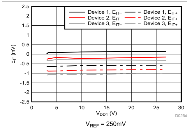
图 5-32. Cmp1 跳变阈值误差与电源电压间的关系
