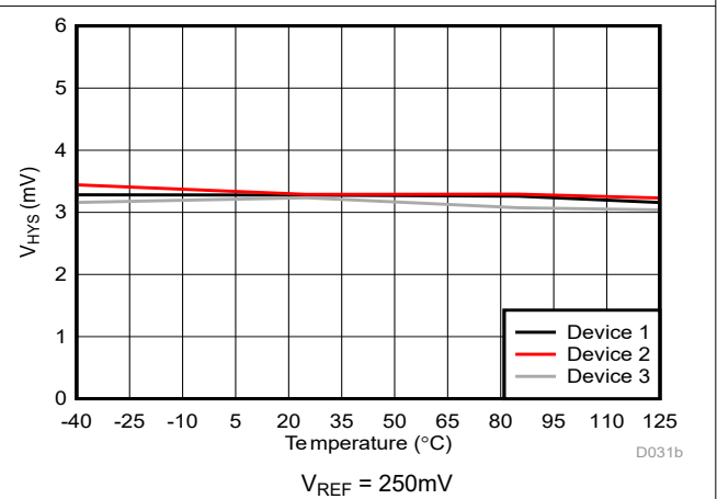
图 5-35. Cmp1 跳变阈值迟滞与温度间的关系
