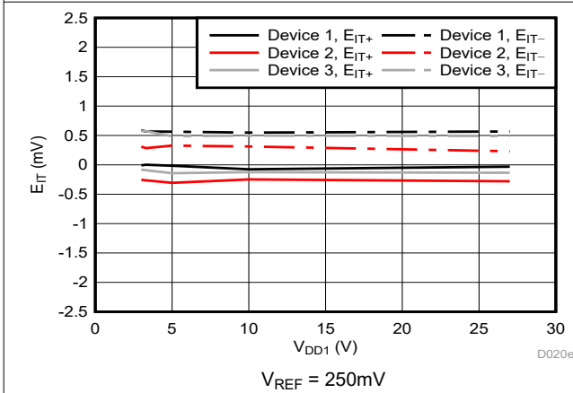
图 5-14. Cmp0 跳变阈值误差与电源电压间的关系
