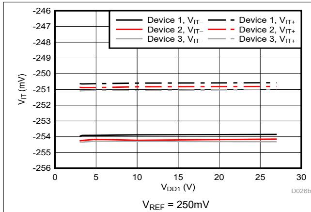
图 5-30. Cmp1 跳变阈值与电源电压间的关系
