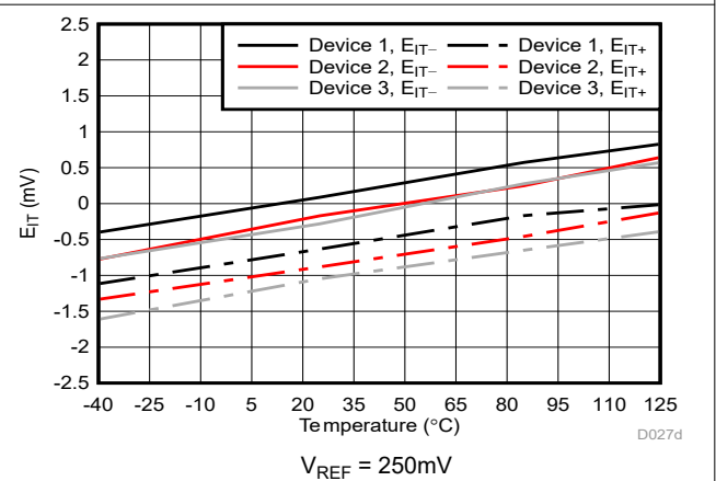
图 5-33. Cmp1 跳变阈值误差与温度间的关系
