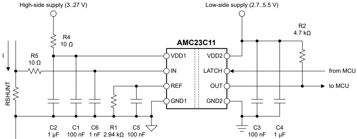
图 7-4. AMC23C11 去耦
