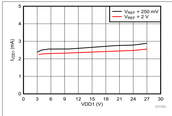
图 5-30. 高侧电源电流与电源电压间的关系
