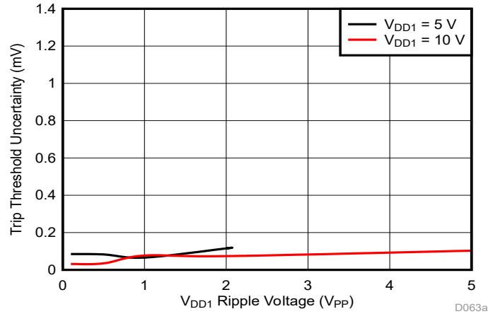
图 7-3. 跳变阈值对 VDD1 纹波电压的灵敏度 ( f_{\text{RIPPLE}} = 10\text{KHz} )
