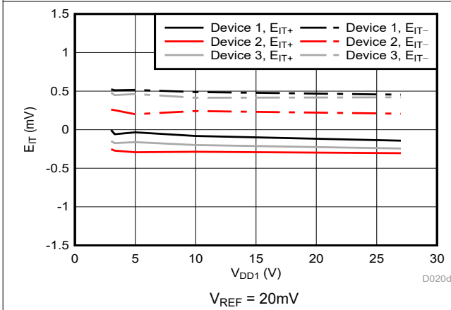
图 5-8. 跳变阈值误差与电源电压间的关系
