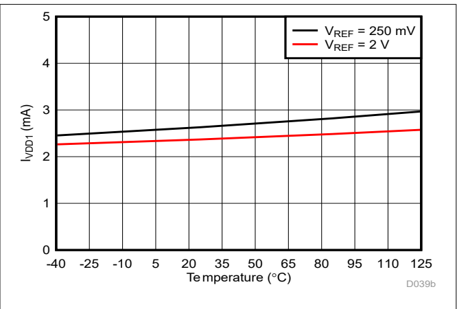
图 5-31. 高侧电源电流与温度间的关系
