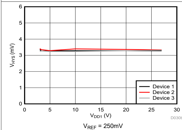
图 5-34. Cmp1 跳变阈值迟滞与电源电压间的关系
