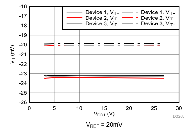
图 5-24. Cmp1 跳变阈值与电源电压间的关系
