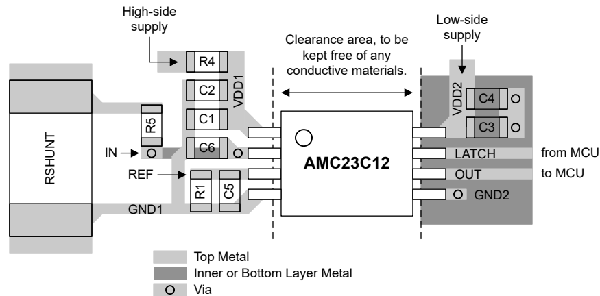
图 8-7. 建议布局 AMC23C12
