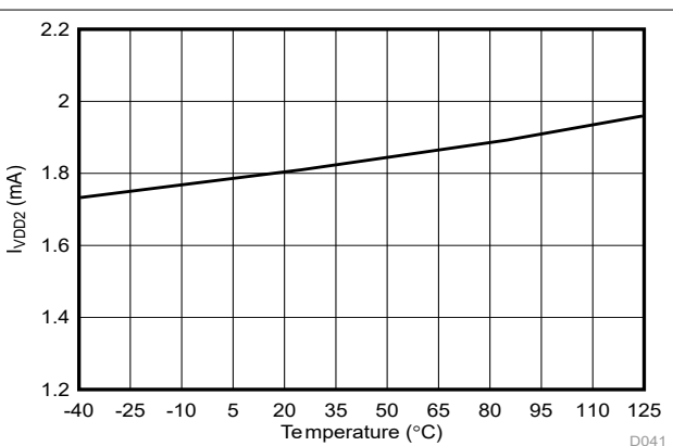
图 5-45. 高侧电源电流与温度间的关系
