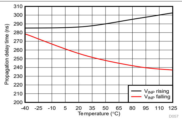
图 5-37. Cmp0 传播延迟与温度间的关系
