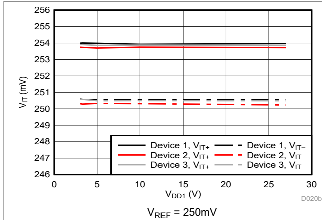
图 6-11. Cmp0 跳变阈值与电源电压间的关系
