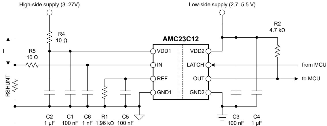
图 8-6. 去耦 AMC23C12
