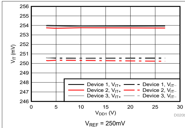
图 5-12. Cmp0 跳变阈值与电源电压间的关系
