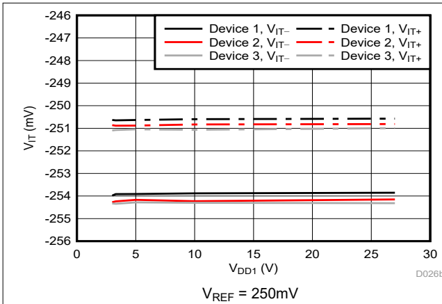
图 5-30. Cmp1 跳变阈值与电源电压间的关系
