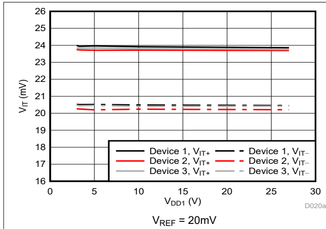
图 5-6. Cmp0 跳变阈值与电源电压间的关系
