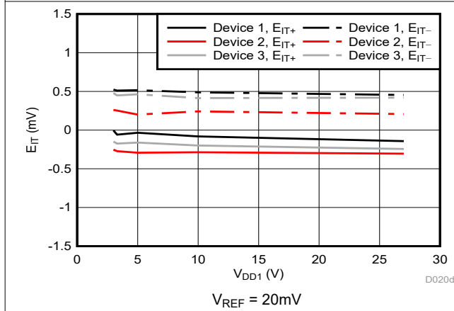
图 5-8. Cmp0 跳变阈值误差与电源电压间的关系
