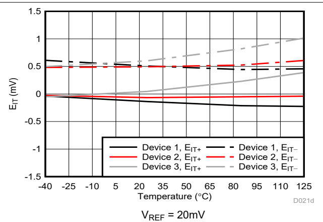
图 6-8. Cmp0 跳变阈值误差与温度间的关系
