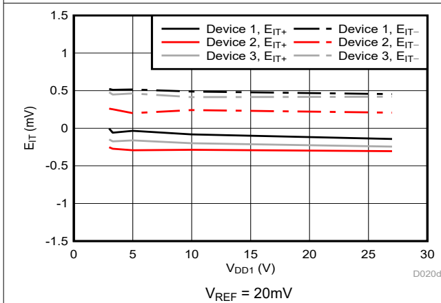
图 6-7. Cmp0 跳变阈值误差与电源电压间的关系
