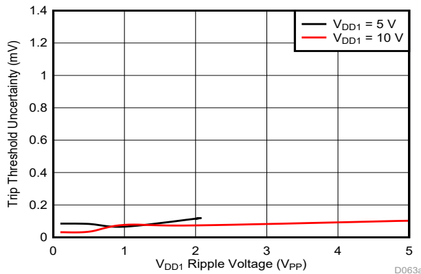
图 8-4. 跳变阈值对 V_{DD1} 纹波电压的灵敏度 ( Cmp0 , f_{RIPPLE} = 10\text{kHz} )
