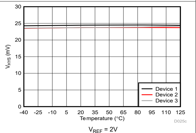
图 5-23. Cmp0 跳变阈值迟滞与温度间的关系
