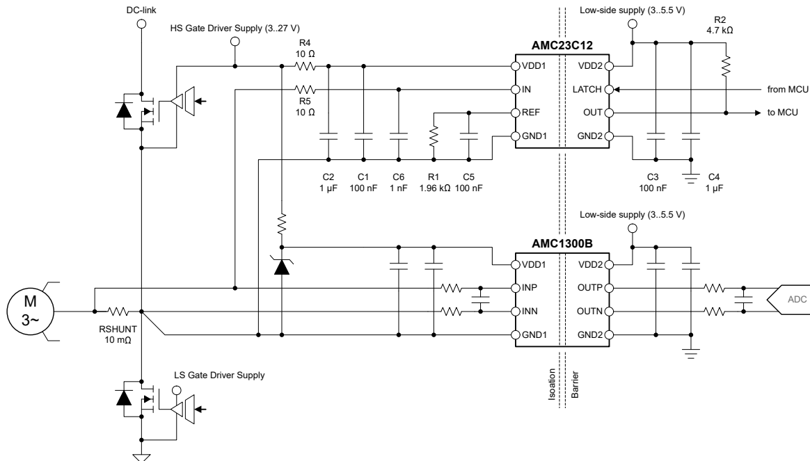
图 8-1. 使用 AMC23C12 进行过流检测
