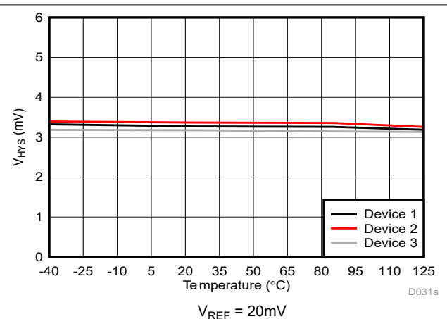
图 5-29. Cmp1 跳变阈值迟滞与温度间的关系
