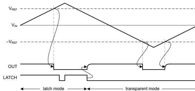
图 6-2. 功能时序图
