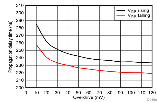
图 5-36. Cmp0 传播延迟与过驱间的关系
