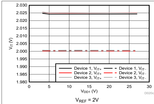
图 5-18. Cmp0 跳变阈值与电源电压间的关系
