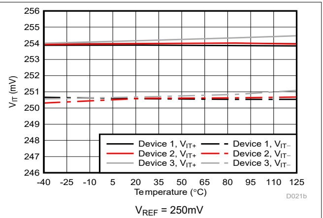
图 5-13. Cmp0 跳变阈值与温度间的关系
