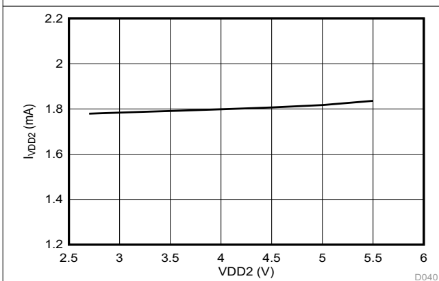
图 5-44. 高侧电源电流与电源电压间的关系
