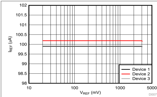
图 5-42. 基准电流与基准电压间的关系
