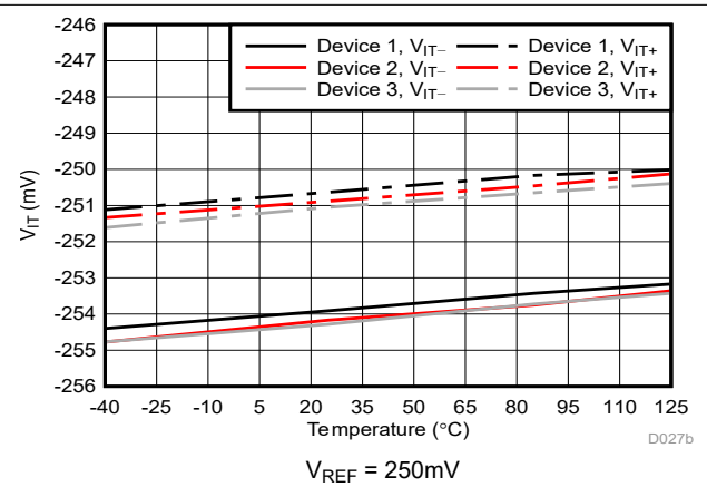
图 5-31. Cmp1 跳变阈值与温度间的关系
