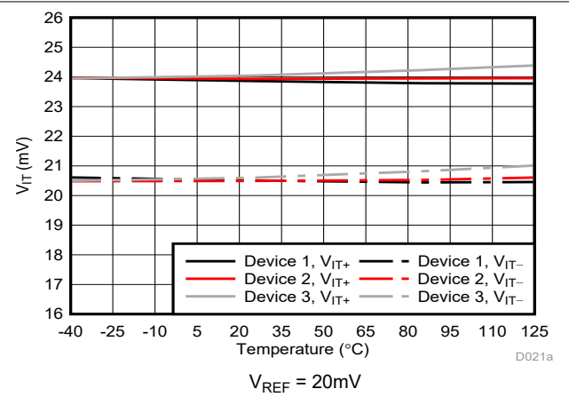
图 6-6. Cmp0 跳变阈值与温度间的关系
