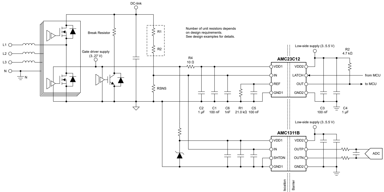
图 8-2. 使用 AMC23C12 进行过压检测
