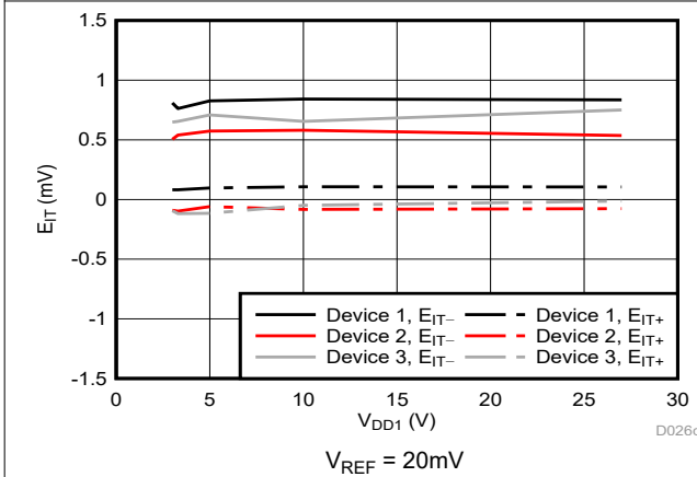
图 5-26. Cmp1 跳变阈值误差与电源电压间的关系
