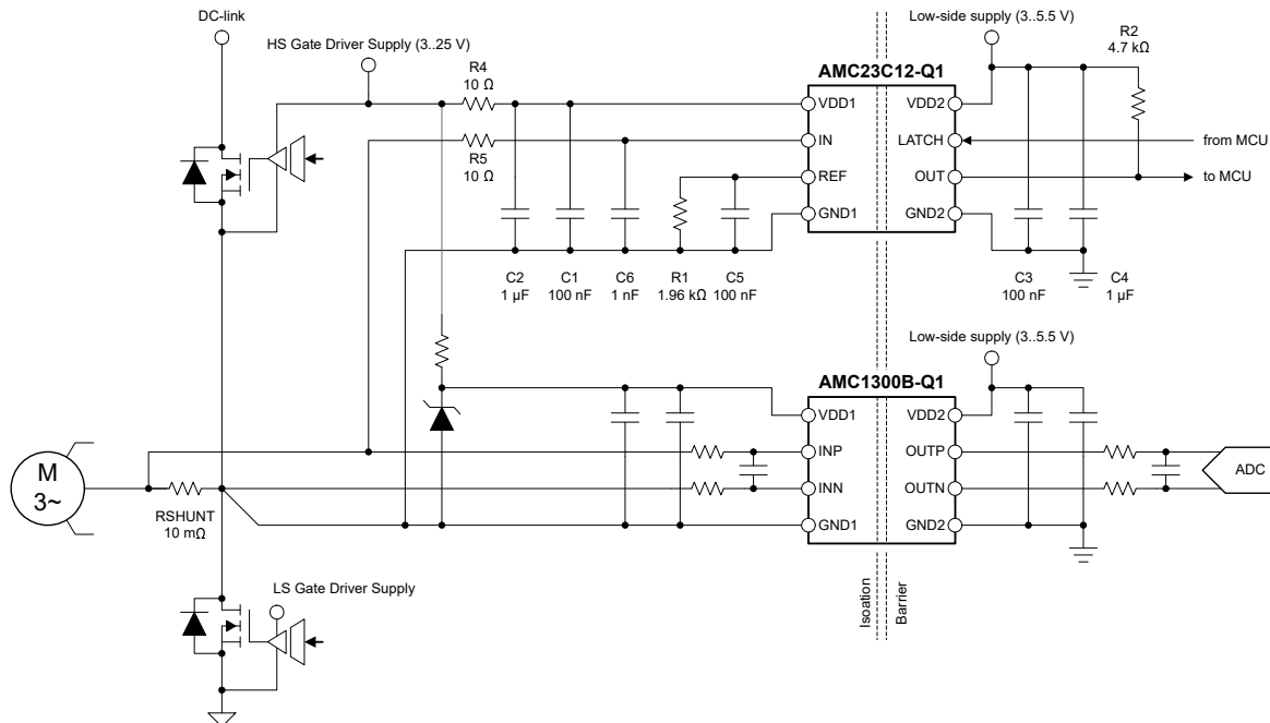
图 8-1. 使用 AMC23C12-Q1 进行过流检测
