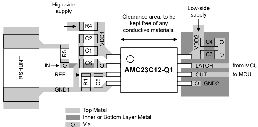
图 8-7. 建议布局 AMC23C12-Q1
