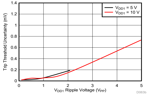
图 8-5. 跳变阈值对 V_{\text{DD1}} 纹波电压的灵敏度 (Cmp1, f_{\text{RIPPLE}} = 10\text{kHz} )
