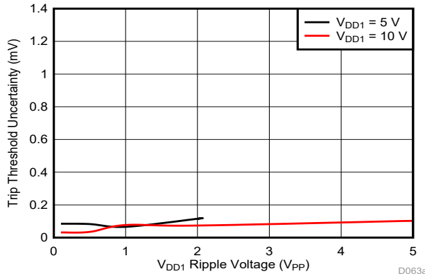
图 8-4. 跳变阈值对 V_{\text{DD1}} 纹波电压的灵敏度 (Cmp0, f_{\text{RIPPLE}} = 10\text{kHz} )
