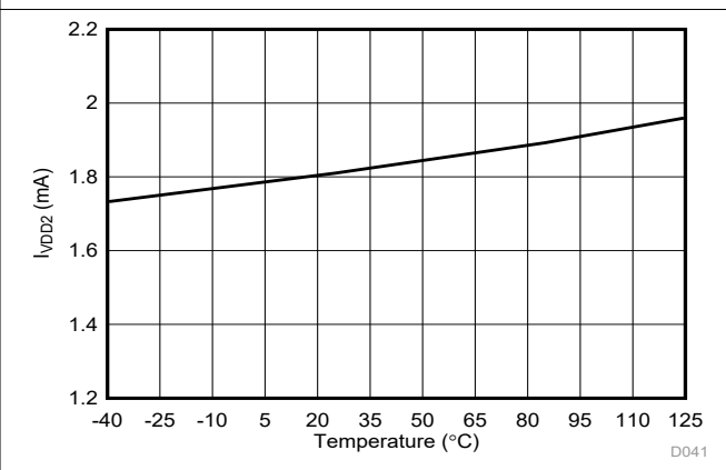
图 6-46. 低侧电源电流与温度间的关系
