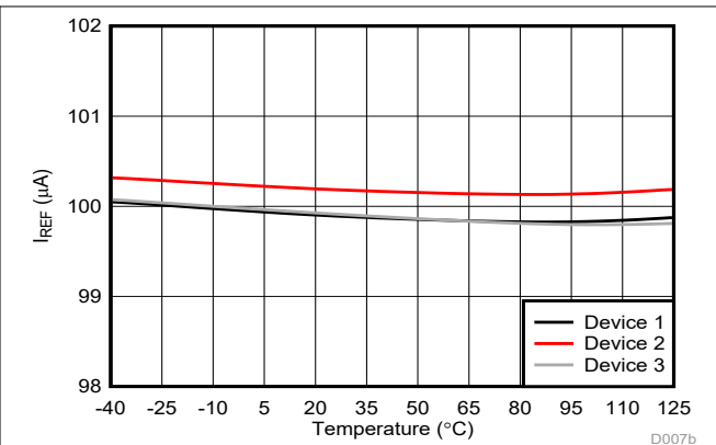
图 6-42. 基准电流与温度间的关系
