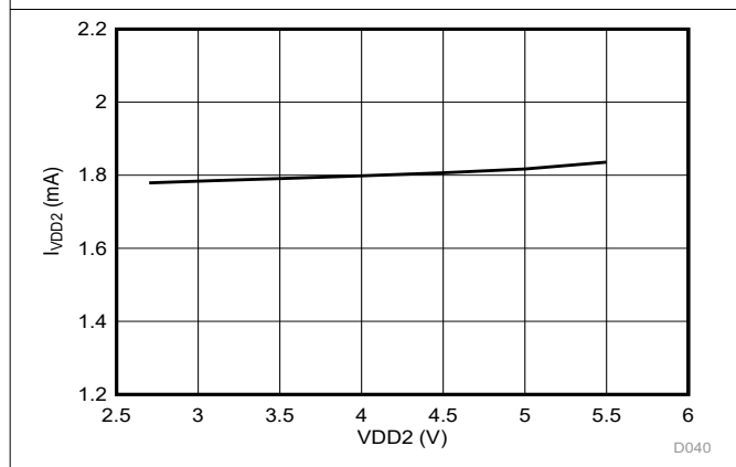
图 6-45. 低侧电源电流与电源电压间的关系
