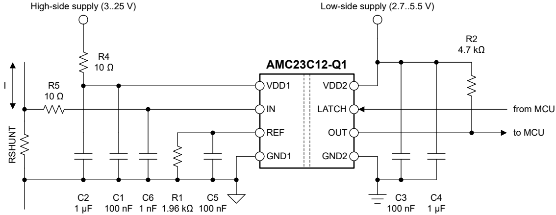
图 8-6. 去耦 AMC23C12-Q1
