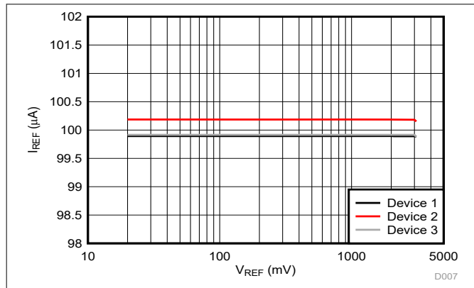
图 6-41. 基准电流与基准电压间的关系
