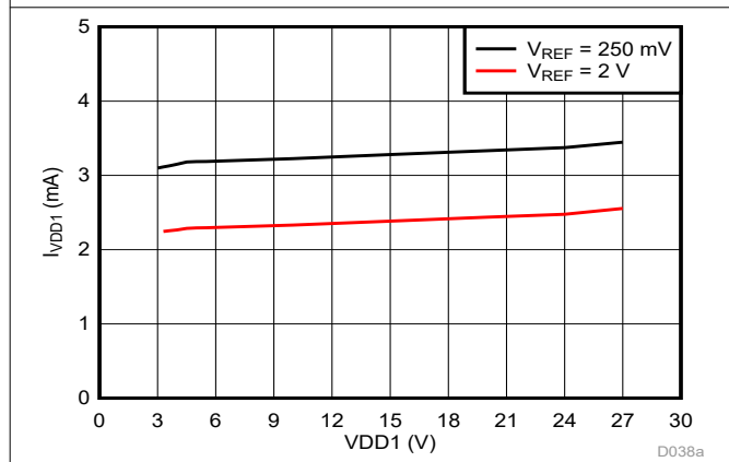
图 6-43. 高侧电源电流与电源电压间的关系
