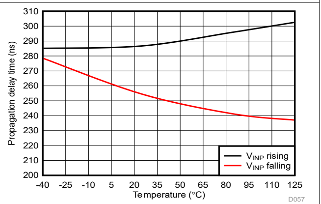
图 5-51. Cmp3 传播延迟与温度间的关系
