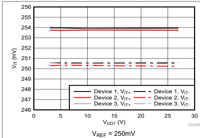
图 5-24. Cmp0 跳变阈值与电源电压间的关系
