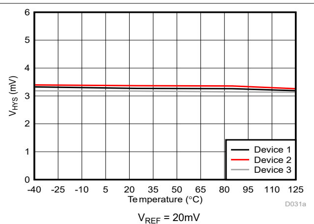
图 5-41. Cmp1 跳变阈值迟滞与温度间的关系
