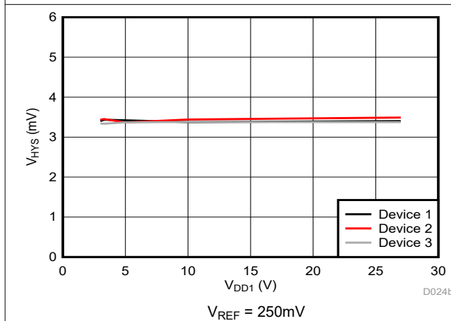
图 5-28. Cmp0 跳变阈值迟滞与电源电压间的关系
