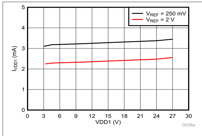
图 5-60. 高侧电源电流与电源电压间的关系
