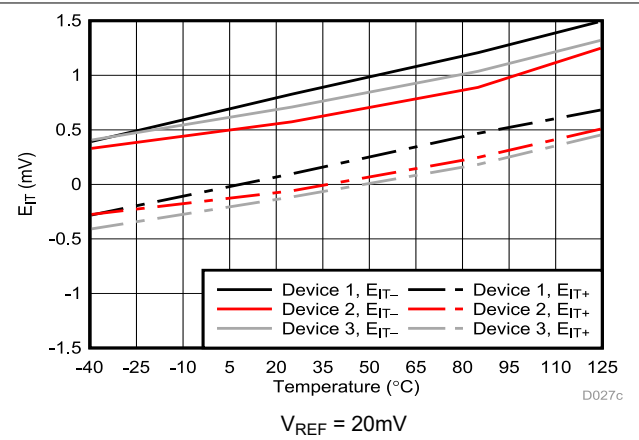
图 5-39. Cmp1 跳变阈值误差与温度间的关系
