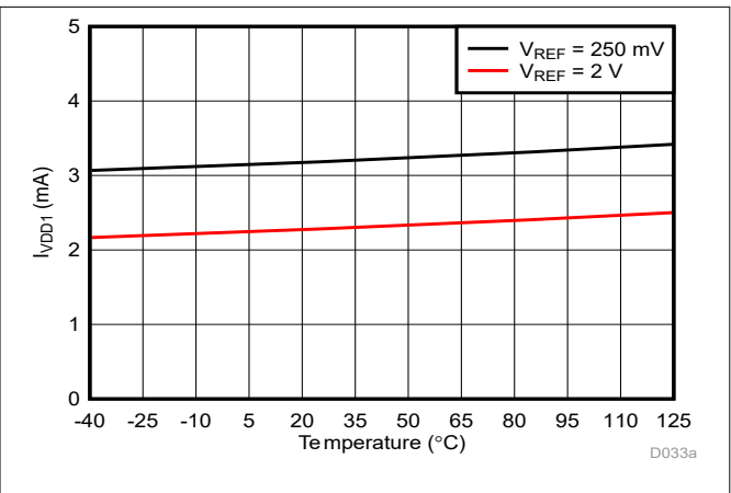
图 5-61. 高侧电源电流与温度间的关系
