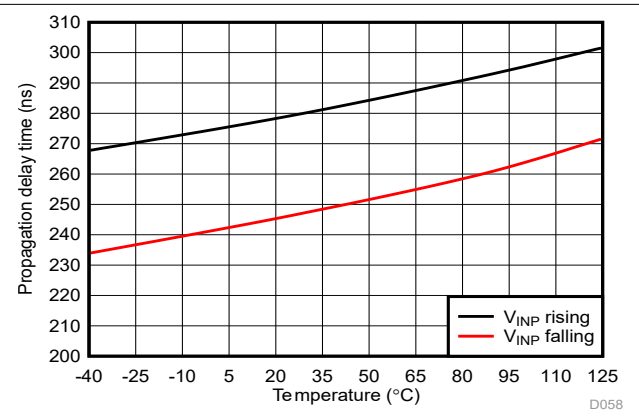
图 5-55. Cmp1 传播延迟与温度间的关系
