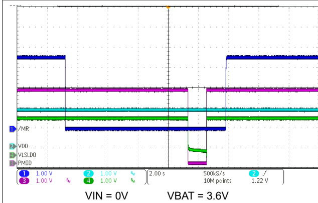
图 8-6. HW Reset on \overline{MR} Long Button Press
