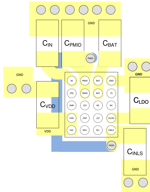
图 10-1. Layout Example
