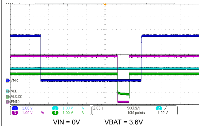
图 8-6. HW Reset on MR Long Button Press
