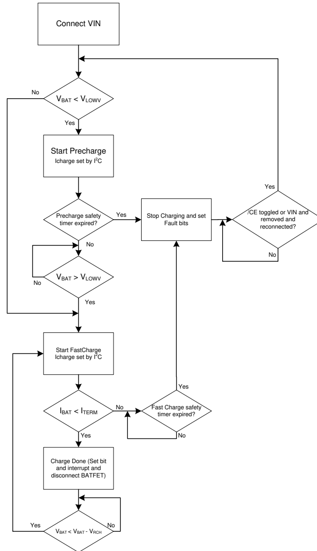
图 7-1. BQ21061 Charger Flow Diagram
