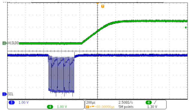
VBAT = 3.6V
