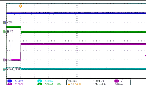
图 8-4. Power Down
