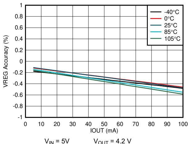
图 6-3. 负载调整率 (4.2V OUT 时为 1s)
