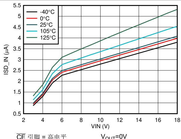
图 6-8. 输入关断电流与输入电压间的关系
