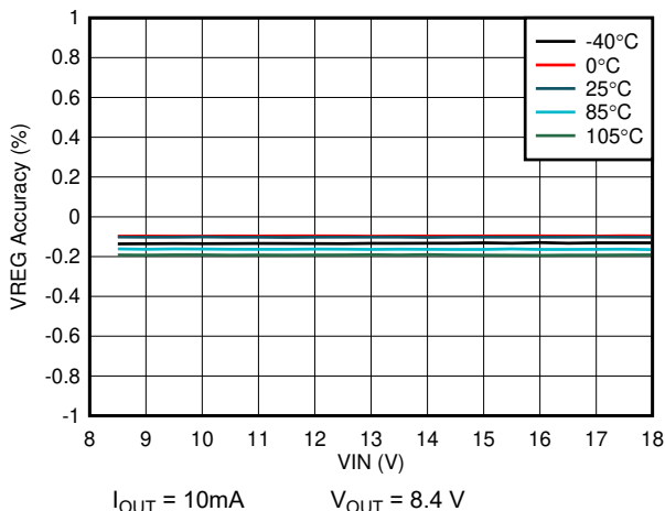
图 6-2. 线性调整率 (8.4V OUT 时为 2s)
