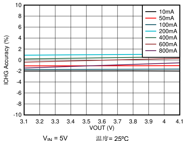
图 6-4. ICHG 精度与 V OUT 间的关系
