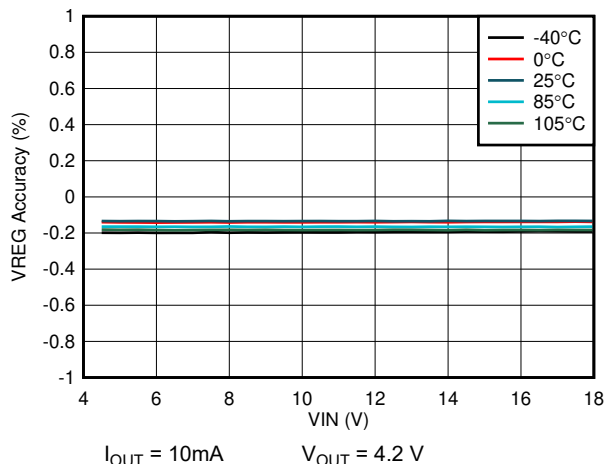
图 6-1. 线性调整率 (4.2V OUT 时为 1s)
