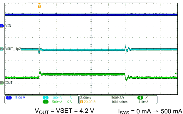
图 8-9. OUT Transient Response
