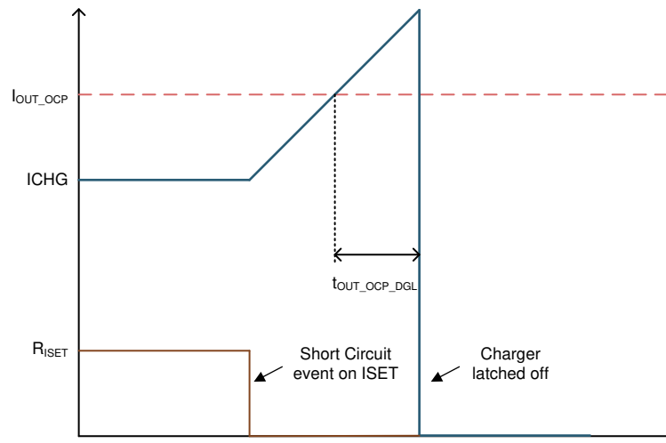
图 7-7. Overcurrent Protection
