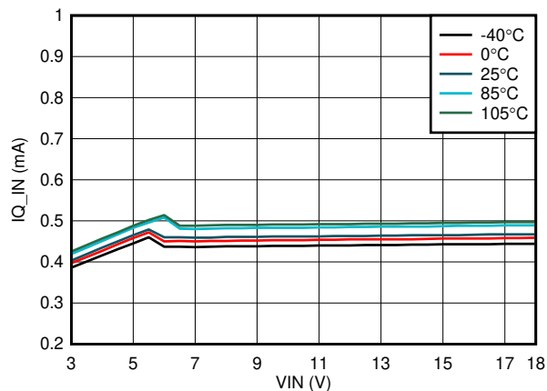
图 6-9. 输入静态电流与输入电压间的关系
