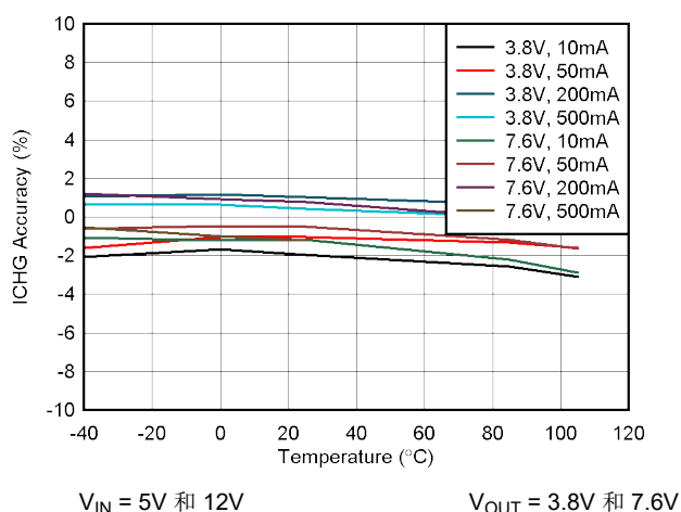
图 6-5. ISET 精度与温度间的关系
