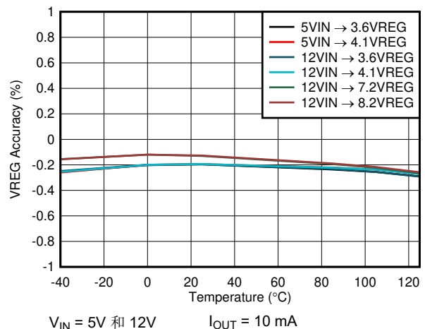
图 6-6. VSET 精度与温度间的关系
