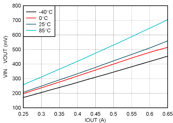
图 6-7. 压降电压与输出电流间的关系
