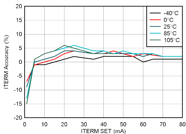
图 6-11. 终止电流精度与终止电流设置间的关系
