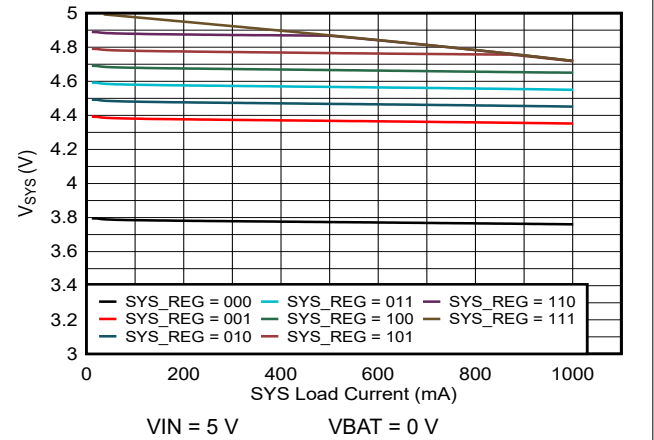
图 7-4. SYS Load Regulation
