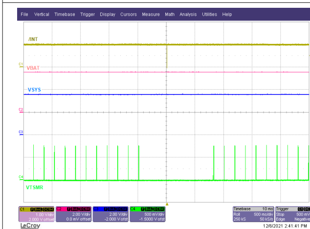
图 9-18. Wake1 Interrupt without VIN
