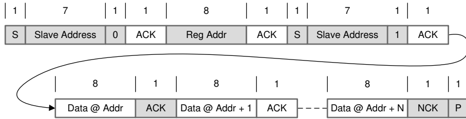
图 9-19. Multi-Read
