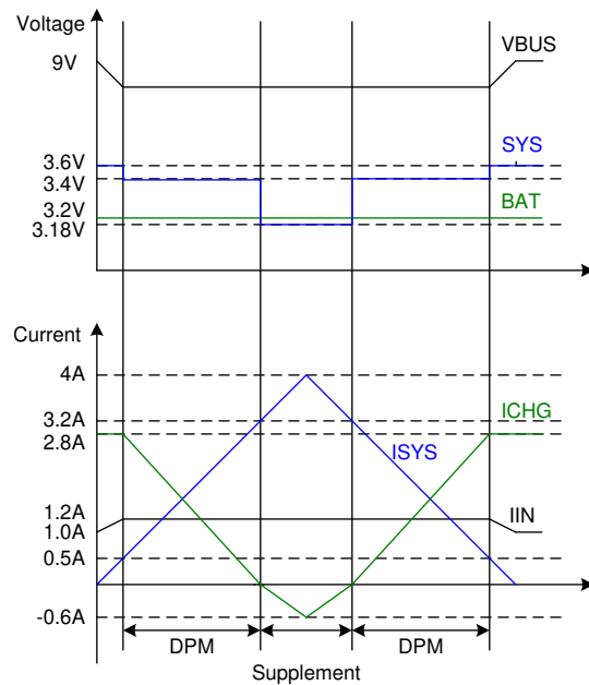
图 9-8. DPM Response
