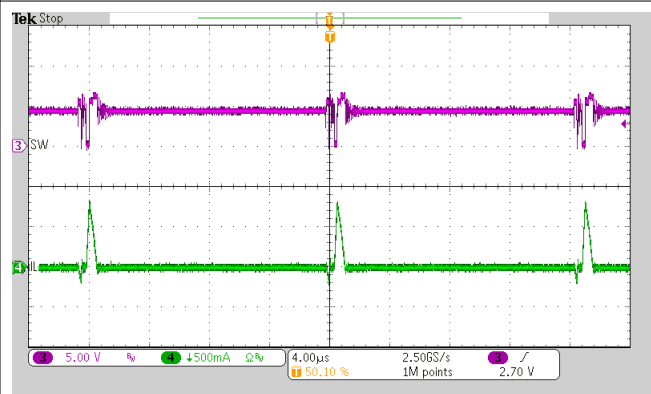
图 10-9. Charge Enable
