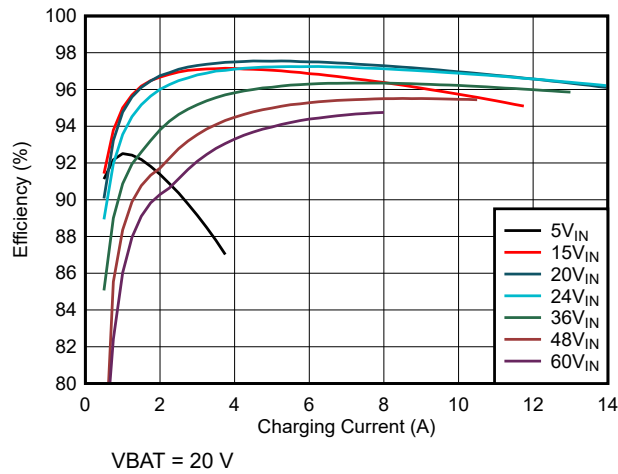
图 7-1. 充电效率与充电电流间的关系 (5 节串联电池配置)
