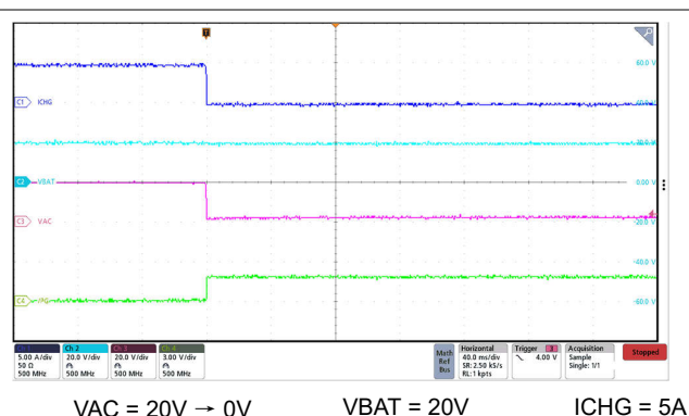
图 9-4. 5A ICHG 下的 VAC 拔下断电
