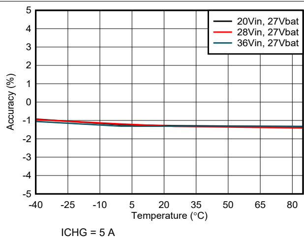
图 7-5. 充电电流精度与温度间的关系
