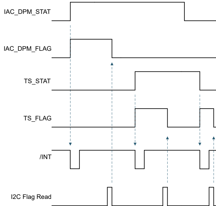
图 8-7. INT 生成行为示例
