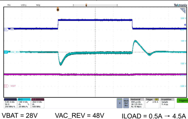
图 9-17. 反向模式升压瞬态响应
