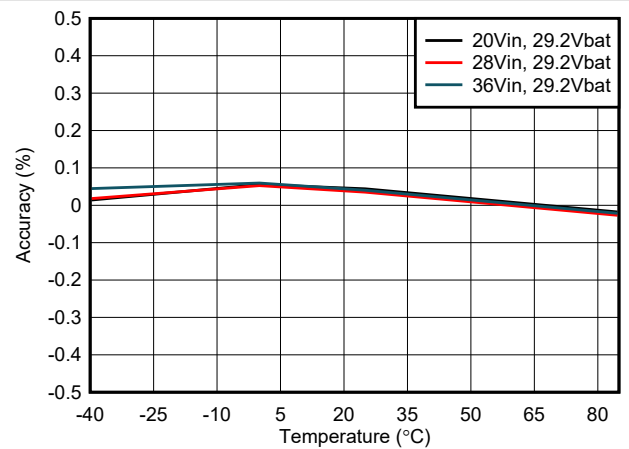
图 7-4. 充电电压精度与温度间的关系
