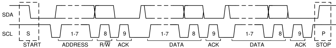
图 8-11. I 2 C 总线上的完整数据传输
