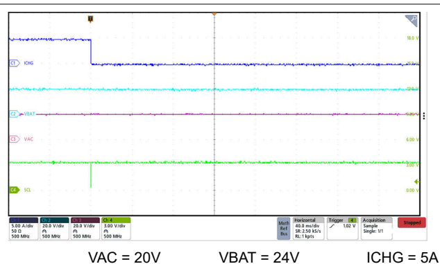
图 9-6. 5A ICHG 下通过 I 2 C 实现的充电禁用
