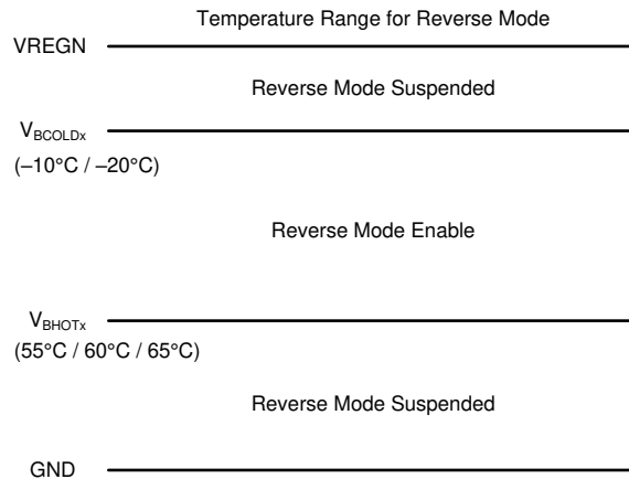
图 8-5. 反向模式下的 TS 引脚热敏电阻检测阈值
