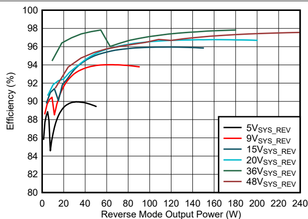
图 7-9. 反向模式效率 (5 节串联电池配置)
