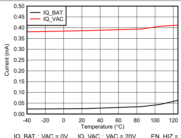
图 7-6. VBAT = 28V 时电池和输入静态电流与温度间的关系
