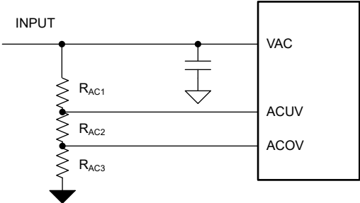
图 9-2. ACUV 和 ACOV 电阻分压器
