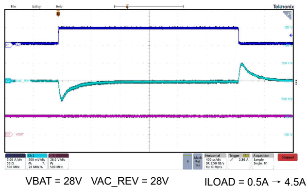
图 9-16. 反向模式降压/升压瞬态响应
