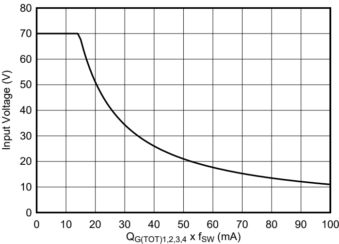
图 8-2. REGN LDO 安全工作区 (SOA)
