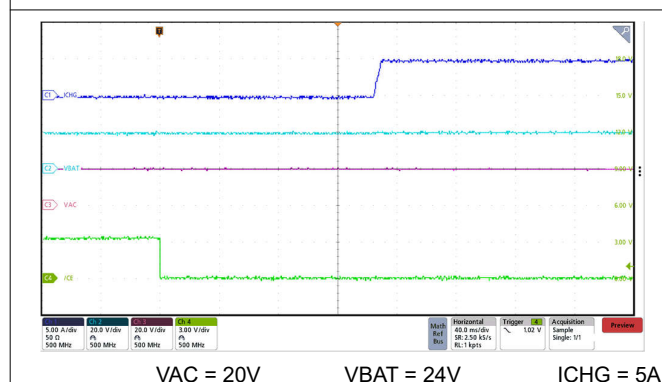
图 9-7. 5A ICHG 下通过 \overline{CE} 引脚实现的充电启用
