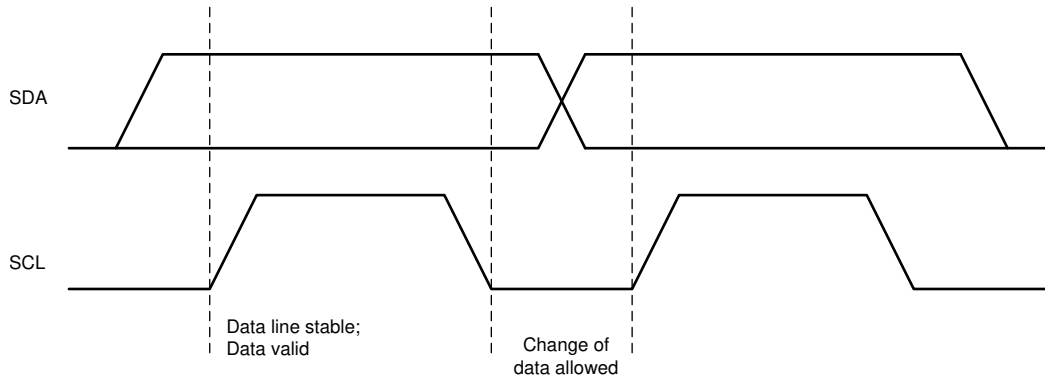
图 8-8. I 2 C 总线上的位传输
