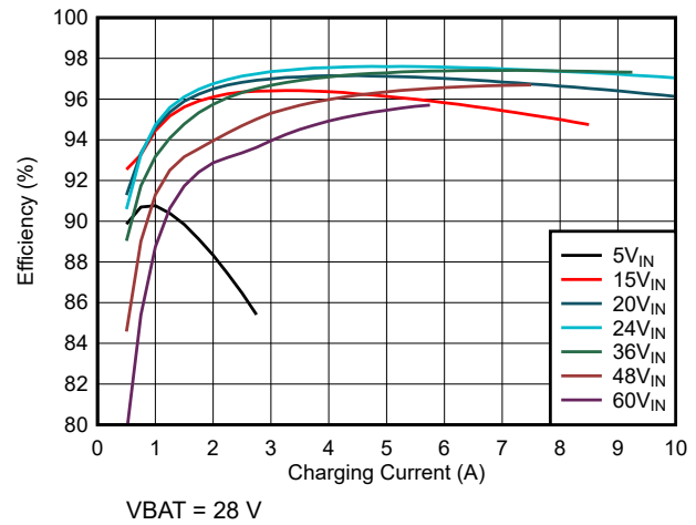
图 7-2. 充电效率与充电电流间的关系 (7 节串联电池配置)
