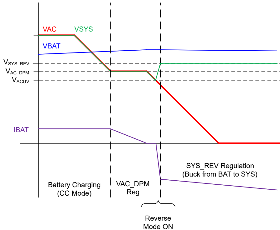
图 8-6. 移除 VAC 后, 如果 BAT > VSYS_REV, 则进入自动反向模式
