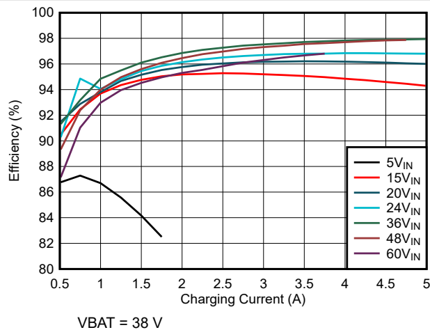
图 7-3. 充电效率与充电电流间的关系 (10 节串联电池配置)
