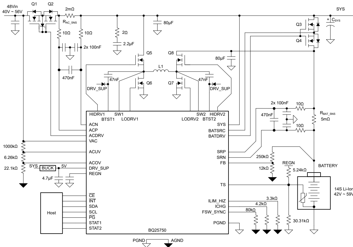
图 9-1. BQ25750 : I 2 C 控制，48VAC，采用 14 节锂离子电池，10A 充电电流和 350kHz 开关频率
