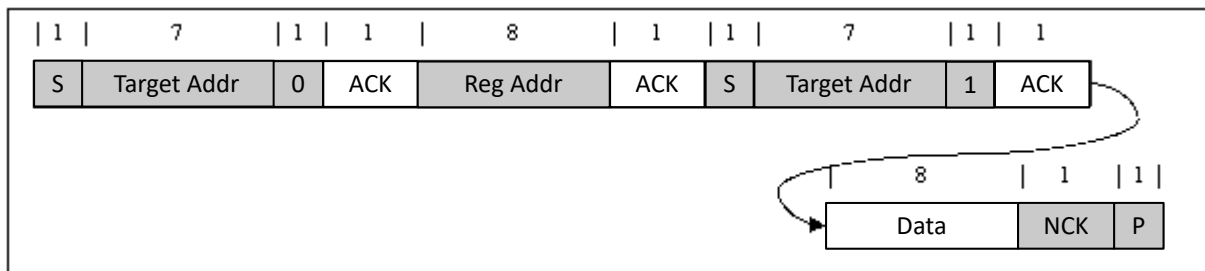
图 8-13. 单次读取
