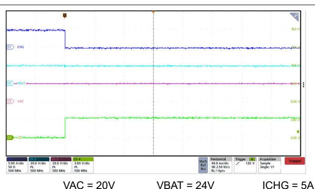
图 9-8. 5A ICHG 下通过 \overline{CE} 引脚实现的充电禁用
