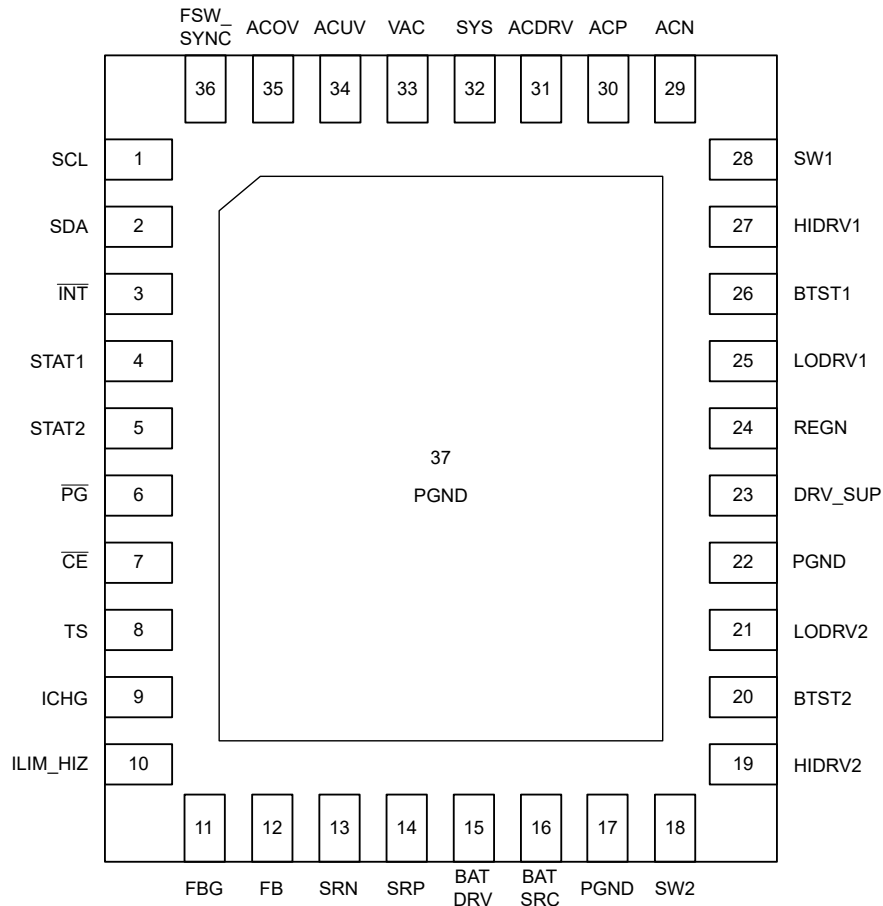
图 6-1. BQ25750 RRV 封装 36 引脚 VQFN 顶视图
