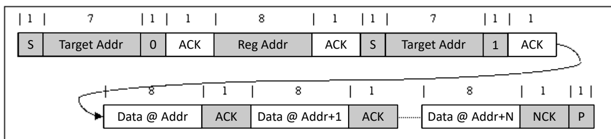
图 8-15. 多重读取
