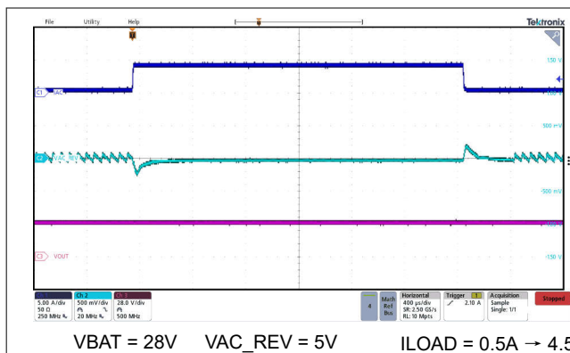
图 9-15. 反向模式降压瞬态响应
