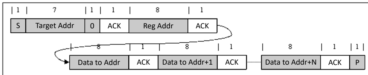
图 8-14. 多重写入
