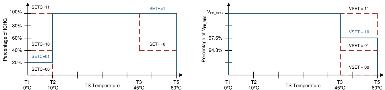
图 8-4. TS 充电值
