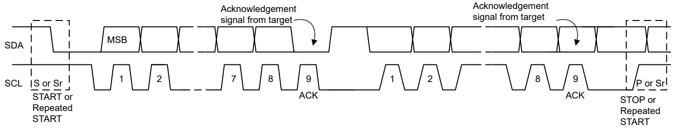
图 8-10. I 2 C 总线上的数据传输
