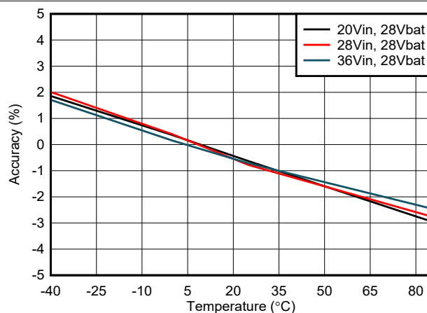
图 7-8. 输入电流 (IAC_DPM) 调节精度与温度间的关系
