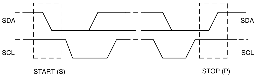
图 8-9. I 2 C 总线上的 START 和 STOP 条件
