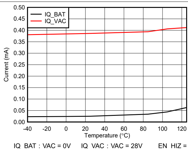
图 6-6. VBAT = 20V 时电池和输入静态电流与温度间的关系
