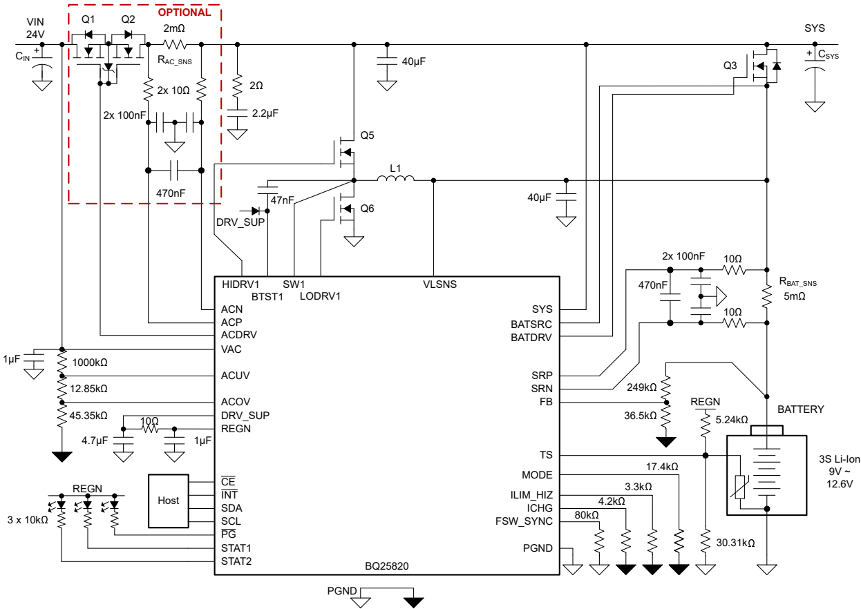
图 8-1. BQ25820 : I 2 C 控制型，24VAC，采用 3 节串联锂离子电池，10A 充电电流和 350kHz 开关频率
