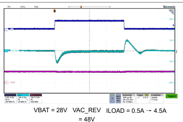
图 8-8. 反向模式升压瞬态响应
