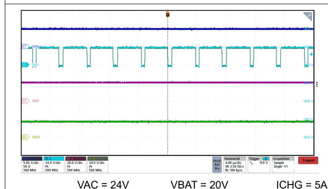
图 8-7. 降压开关波形
