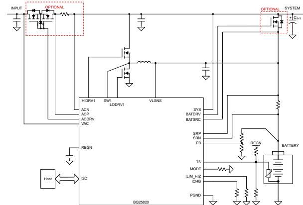
BQ25820 简化原理图
