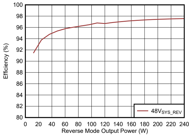
VBAT = 38V 图 6-11. 反向模式效率 (10 节串联电池配置)
