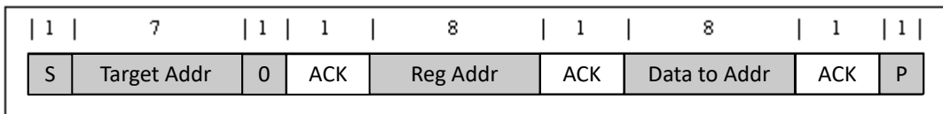
图 7-11. 单独写入
