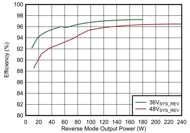
VBAT = 28V 图 6-10. 反向模式效率 (7 节串联电池配置)
