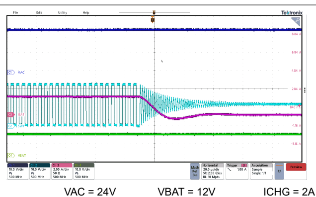
图 8-6. 2A ICHG 下通过 I 2 C 禁用充电
