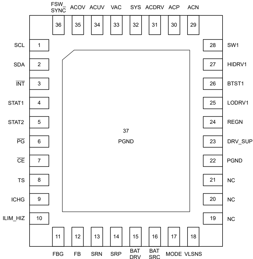
图 5-1. BQ25820 , RRV 封装 36 引脚 VQFN 顶视图
