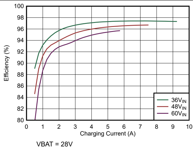
图 6-2. 充电效率与充电电流间的关系 (7 节串联电池配置)
