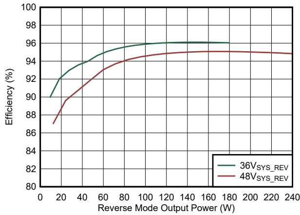
VBAT = 20V 图 6-9. 反向模式效率 (5 节串联电池配置)
