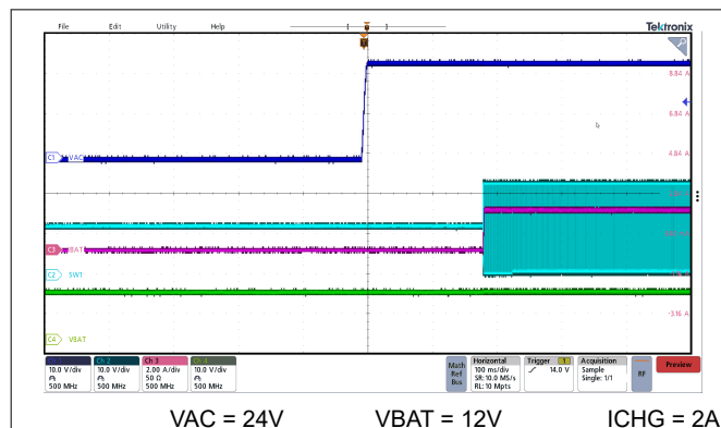
图 8-3. 2A ICHG 下的 VAC 插入上电
