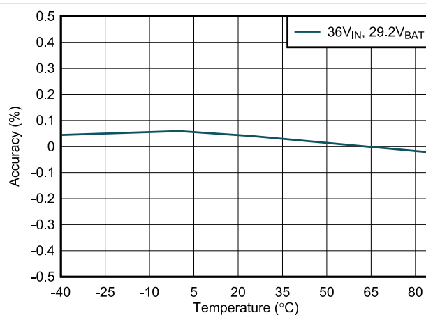
图 6-4. 充电电压精度与温度间的关系
