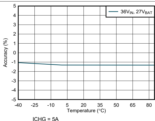
图 6-5. 充电电流精度与温度间的关系
