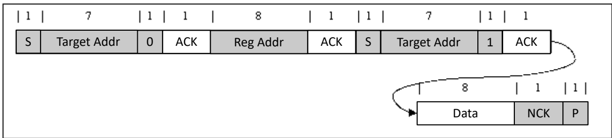
图 7-12. 单次读取
