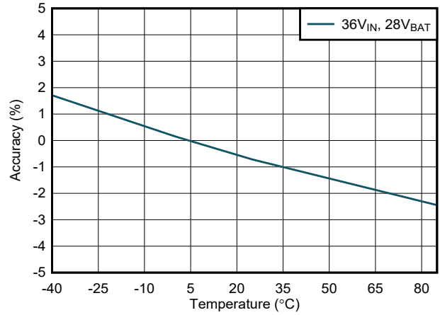
IAC_DPM = 3A 图 6-8. 输入电流 (IAC_DPM) 调节精度与温度间的关系
