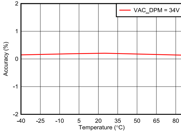
VBAT = 28V 图 6-7. 输入电压 (VAC_DPM) 调节精度与温度间的关系
