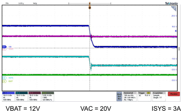
图 8-9. VAC 至 VBAT 电源路径传输
