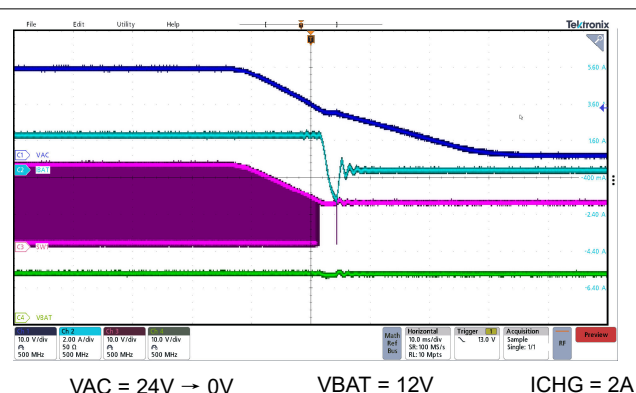
图 8-4. 2A ICHG 下的 VAC 拔下断电
