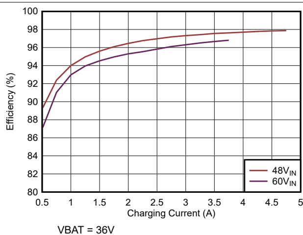
图 6-3. 充电效率与充电电流间的关系 (9 节串联电池配置)
