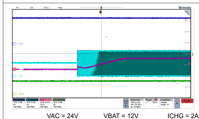
图 8-5. 2A ICHG 下通过 I 2 C 启用充电
