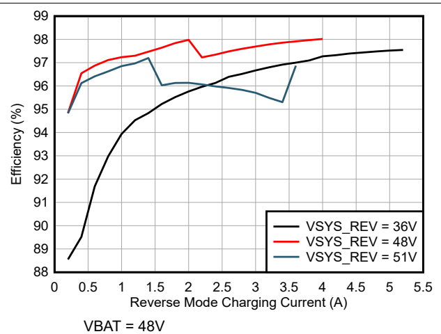
图 6-12. 反向模式效率 (12 节锂离子电池配置)
