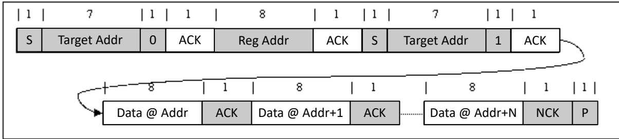
图 7-14. 多重读取
