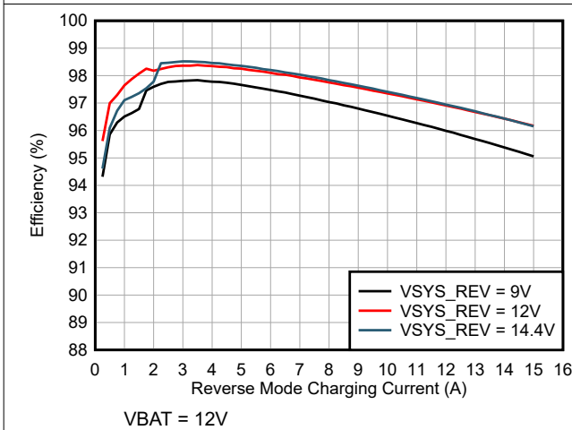
图 6-11. 反向模式效率 (4 节磷酸铁锂电池配置)
