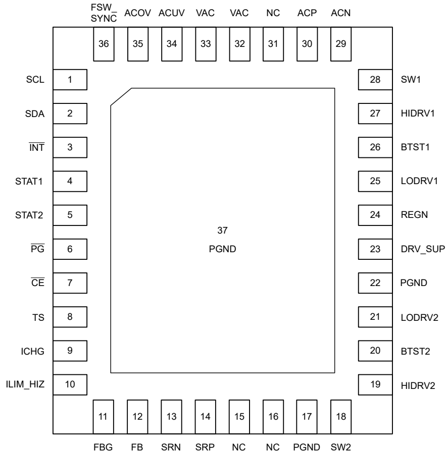
图 5-1. BQ25856-Q1 RRV 封装 36 引脚 VQFN 顶视图
