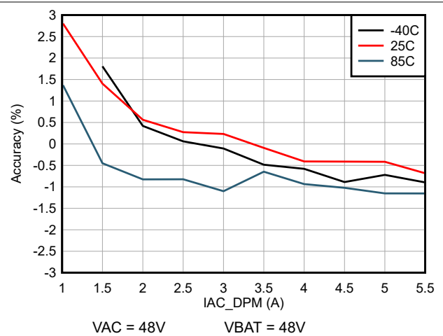
图 6-10. 输入电流 (IAC_DPM) 调节精度 (在不同的温度下)
