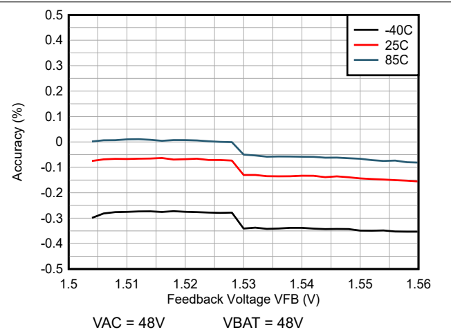
图 6-4. 反馈电压精度 (在不同的温度下)
