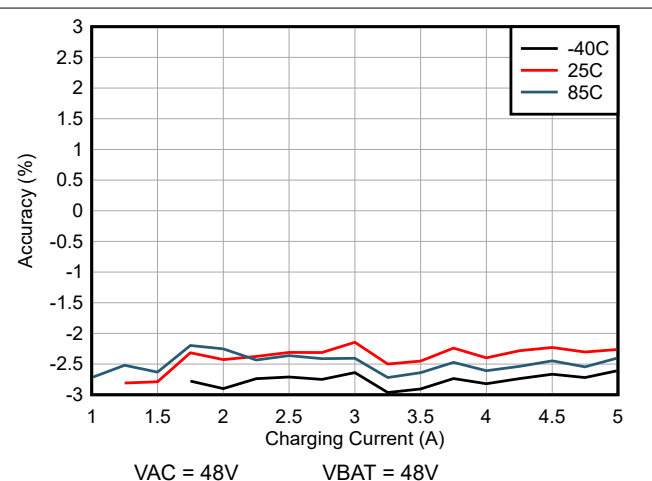
图 6-6. 充电电流精度 (在不同的温度下)
