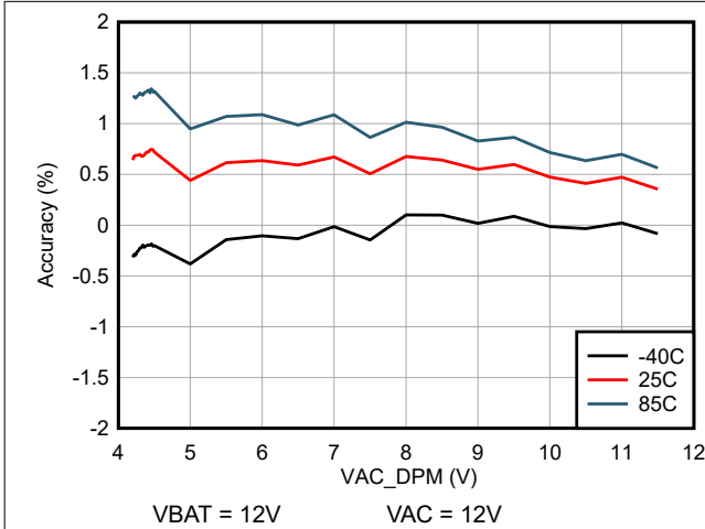
图 6-7. 输入电压 (VAC_DPM) 调节精度 (在不同的温度下)
