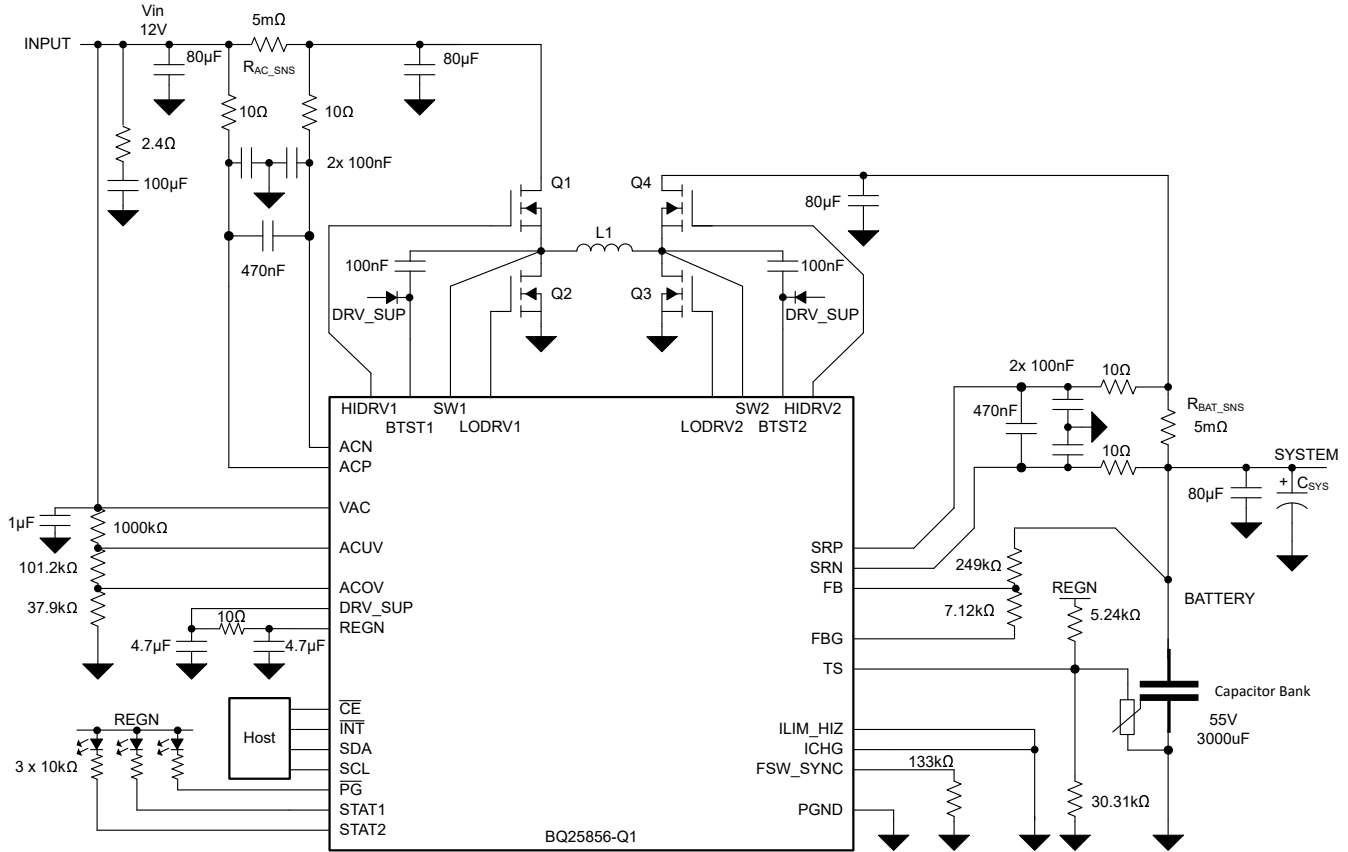
图 8-14. BQ25856-Q1 : 备用电容器或最后关头应用示意图
