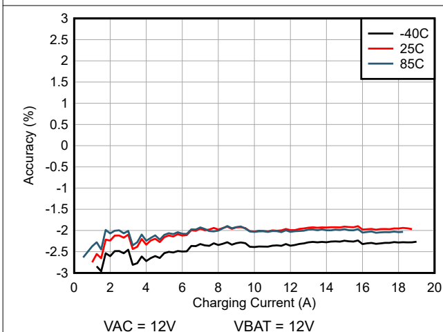
图 6-5. 充电电流精度 (在不同的温度下)
