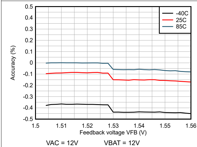
图 6-3. 反馈电压精度 (在不同的温度下)
