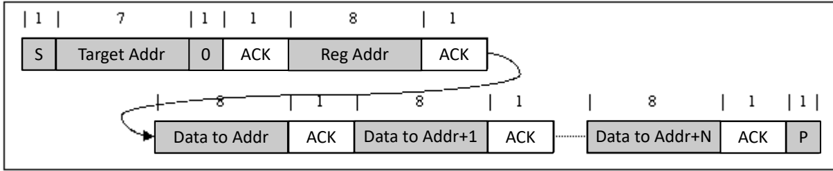
图 7-13. 多重写入
