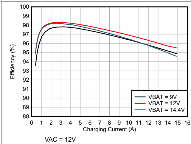
图 6-1. 充电效率与充电电流间的关系 (4 节磷酸铁锂电池配置)
