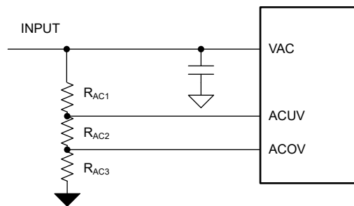
图 8-2. ACUV 和 ACOV 电阻分压器
