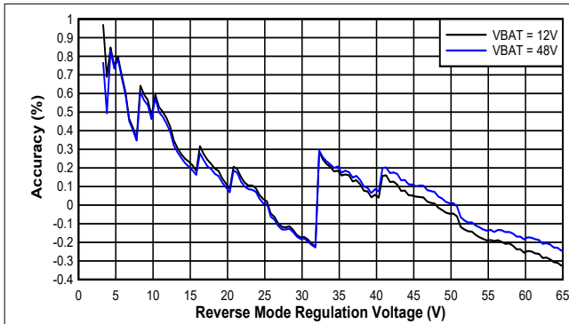
图 6-13. 反向模式输出电压精度与 VAC_REV 设置间的关系
