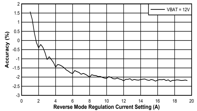
图 6-14. 反向模式输出电流精度与 IAC_REV 设置间的关系
