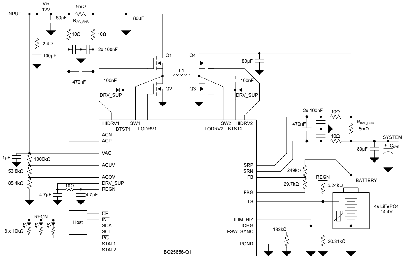
图 8-13. BQ25856-Q1 : 从 12V 输入双向充电，为 4 节磷酸铁锂汽车电池充电
