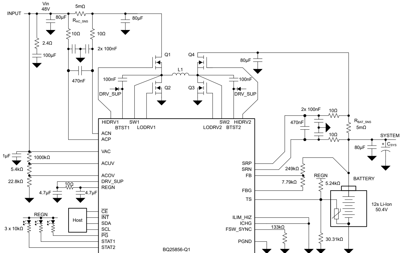
图 8-1. BQ25856-Q1：通过 48V 输入双向充电，为 12 节锂离子汽车电池充电
