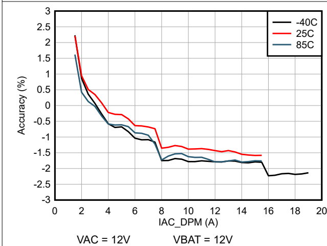
图 6-9. 输入电流 (IAC_DPM) 调节精度 (在不同的温度下)
