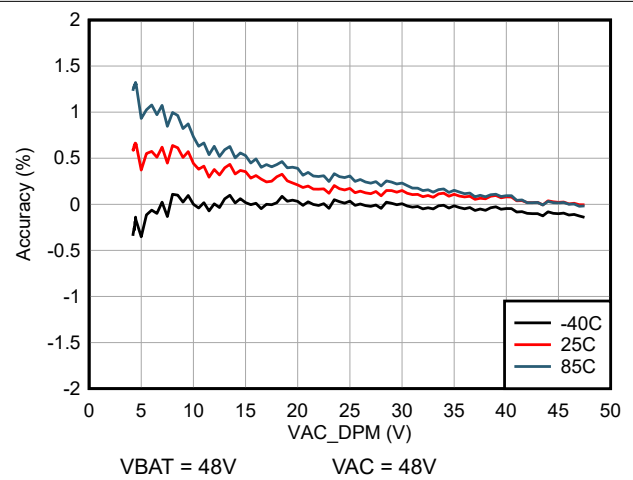
图 6-8. 输入电压 (VAC_DPM) 调节精度 (在不同的温度下)
