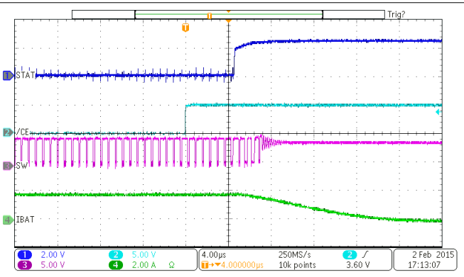
图 10-5. Charge Disable
