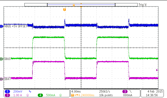
图 9-11. PFM Switching Waveform
