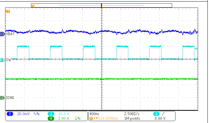
图 48. Charge Enable
