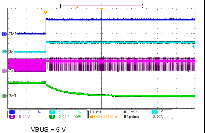
图 44. Charge Disable
