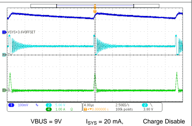
图 44. Charge Disable
