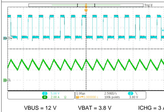
图 43. Charge Enable
