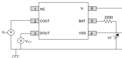
图 7-3. Test Circuit 1
