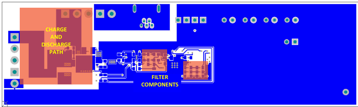
图 11-10. Bottom Layer
