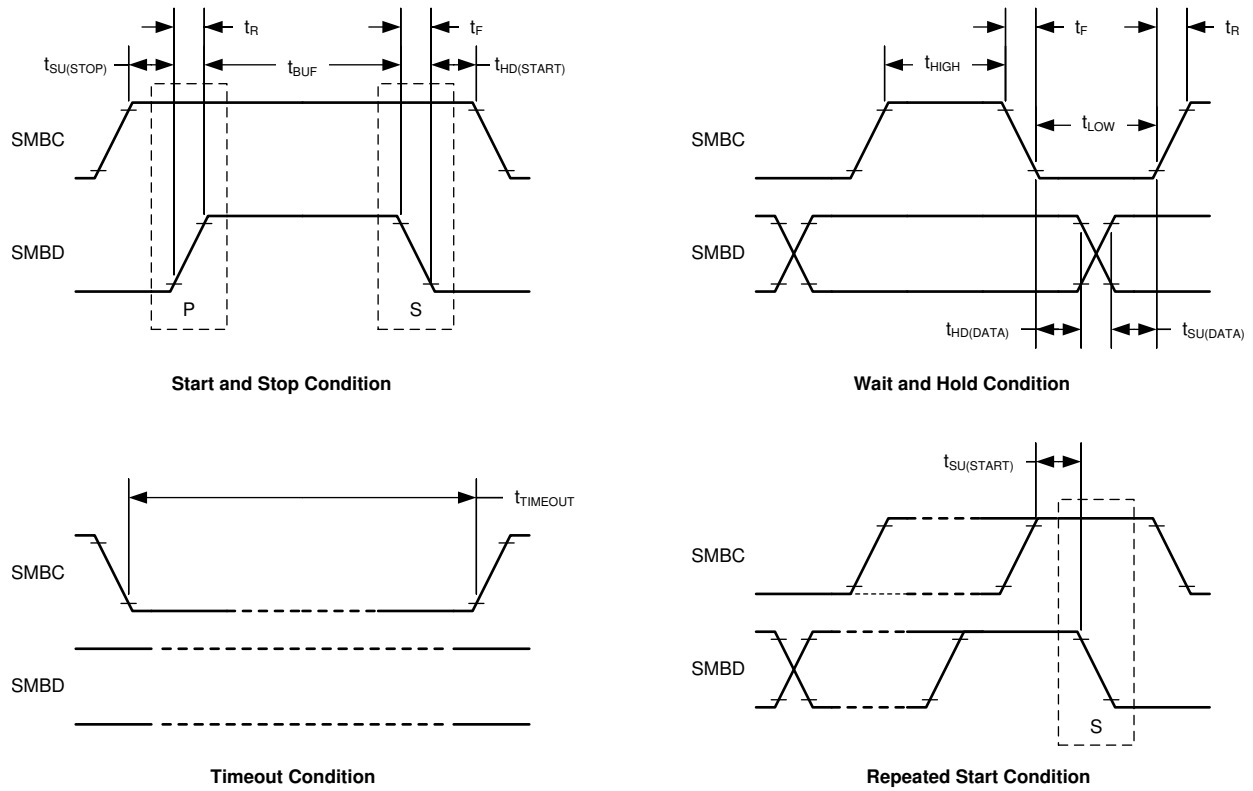
图 7-1. SMBus Timing Diagram
