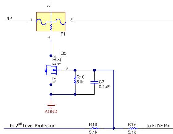
图 9-11. FUSE Circuit
