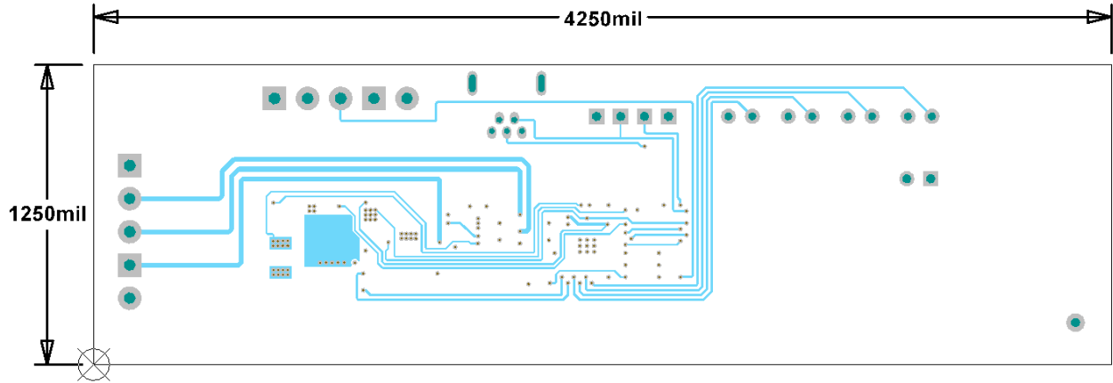
图 11-9. Internal Layer 2
