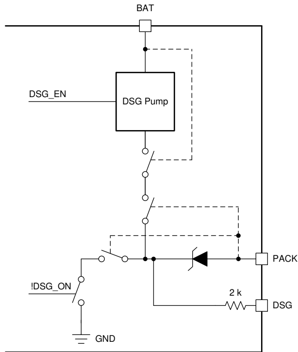
图 5-6. DSG 引脚
