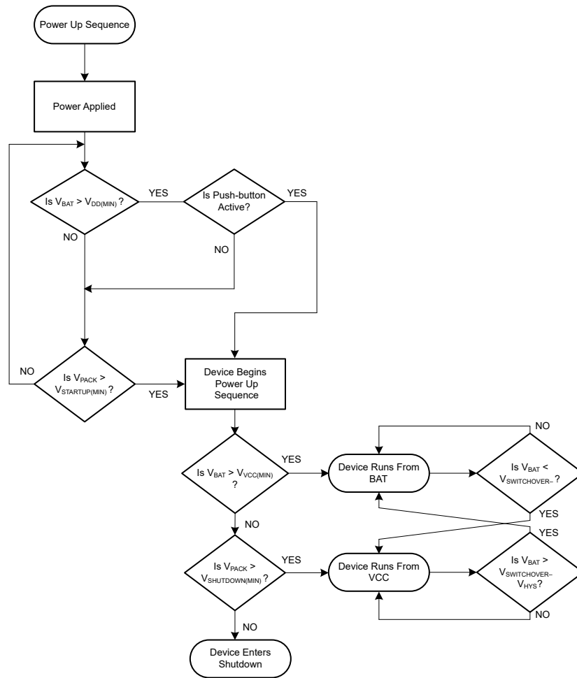
图 7-1. 上电序列
