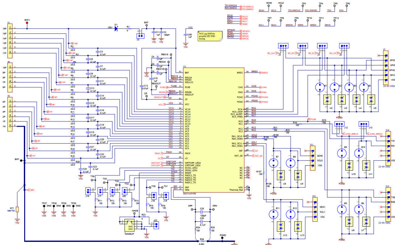
图 8-1. 典型应用
