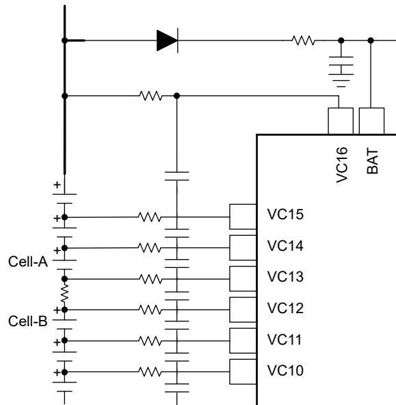
图 7-3. 使用电芯输入引脚进行互连测量
