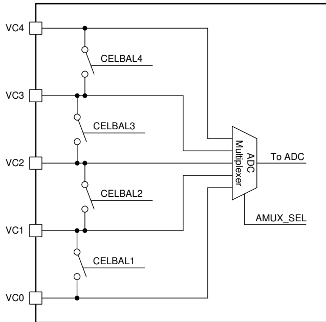
图 5-2. VCx 引脚
