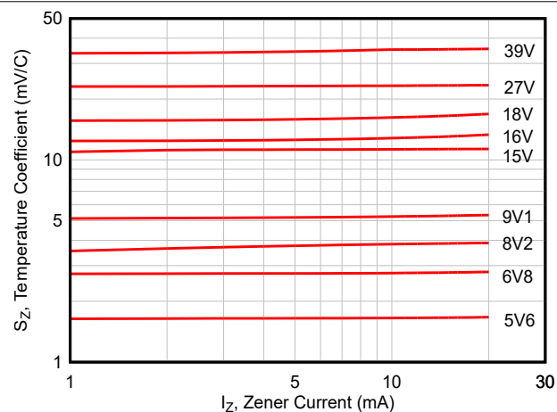
图 6-2. 温度系数
