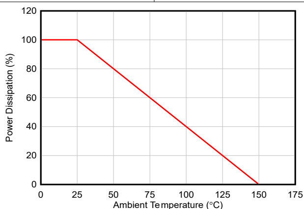
图 5-3. 功率降额曲线
