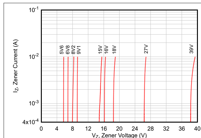
图 5-1. 齐纳电流与齐纳电压间的关系
