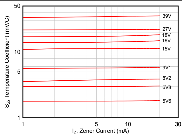
图 5-2. 温度系数
