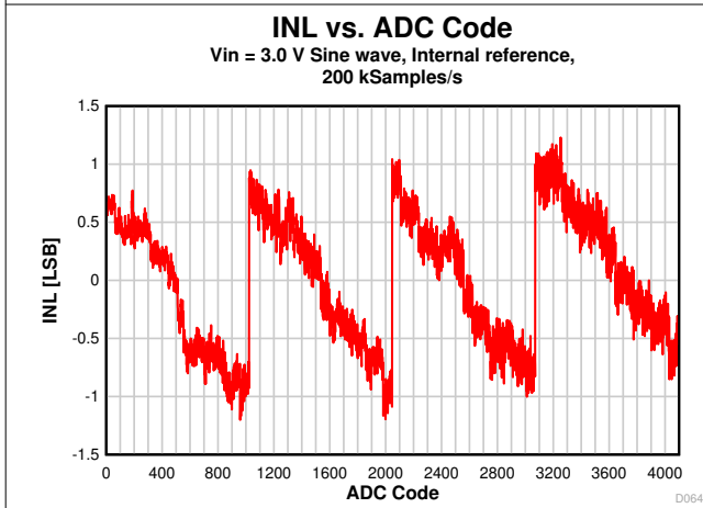
图 8-30. INL vs. ADC Code
