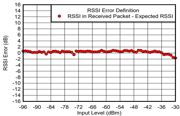
图 7-18. RSSI Error vs. Input Level (dBm)
