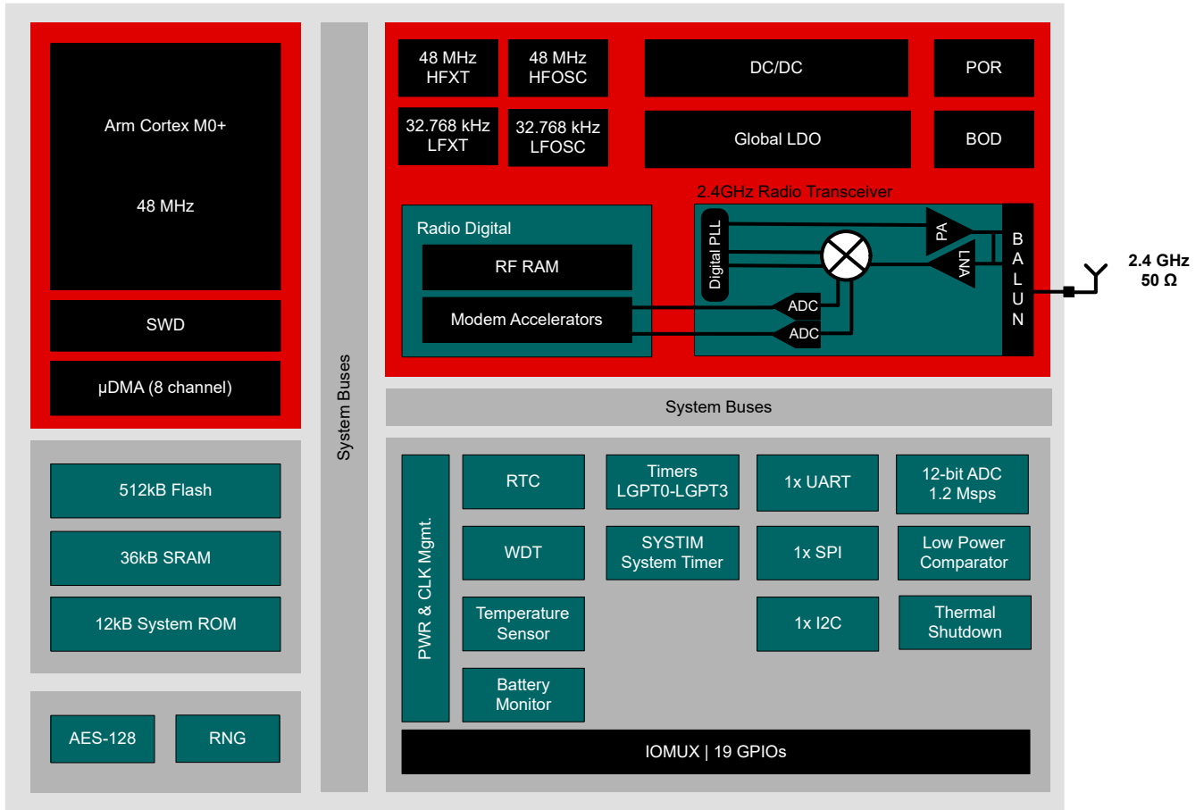
图 4-1. CC2340R5-Q1 方框图
