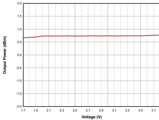
图 7-20. 输出功率与电源电压 (VDD5) 间的关系 ( BLE 1Mbps , 2.44GHz , 0dBm )
