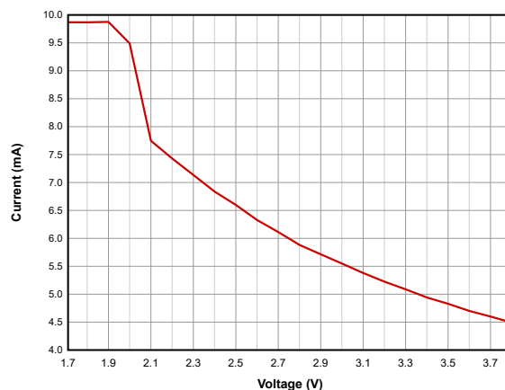
图 7-9. RX 电流与电源电压 (VDD5) 间的关系 ( BLE 1Mbps , 2.44GHz )
