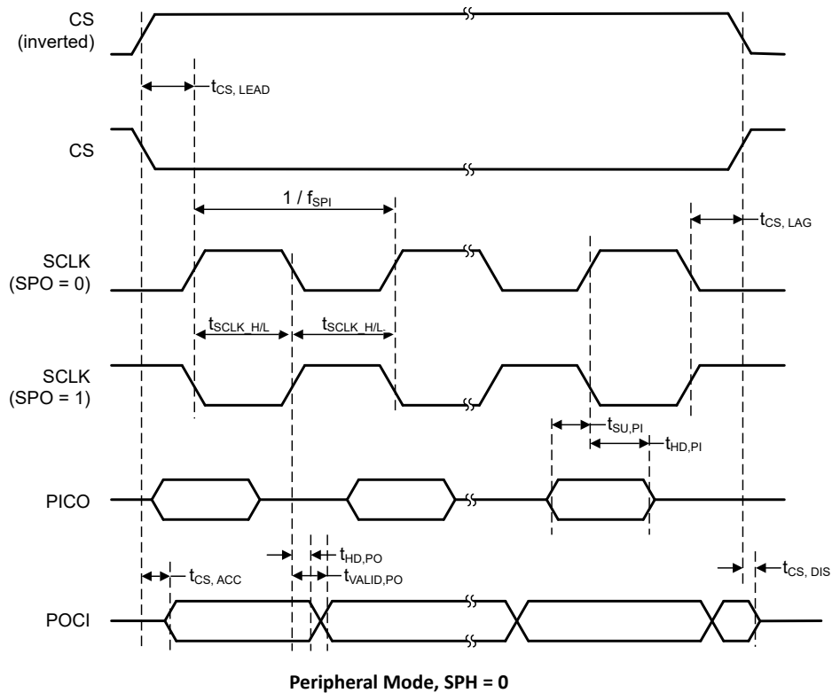
图 7-3. SPI 时序图 - 外设模式，SPH = 0
