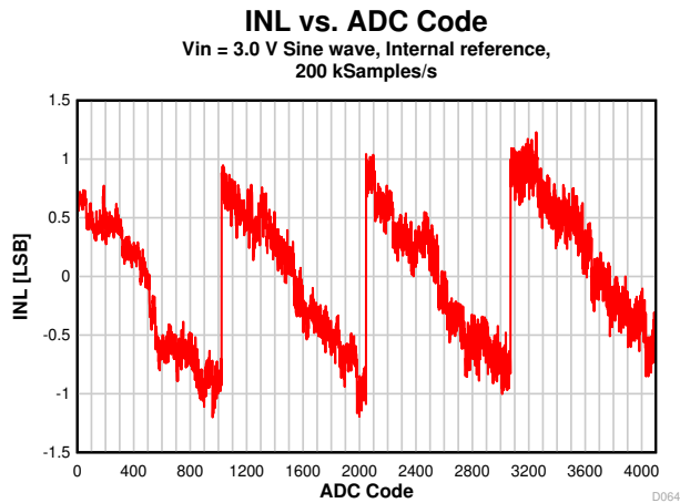
图 8-35. INL vs. ADC Code
