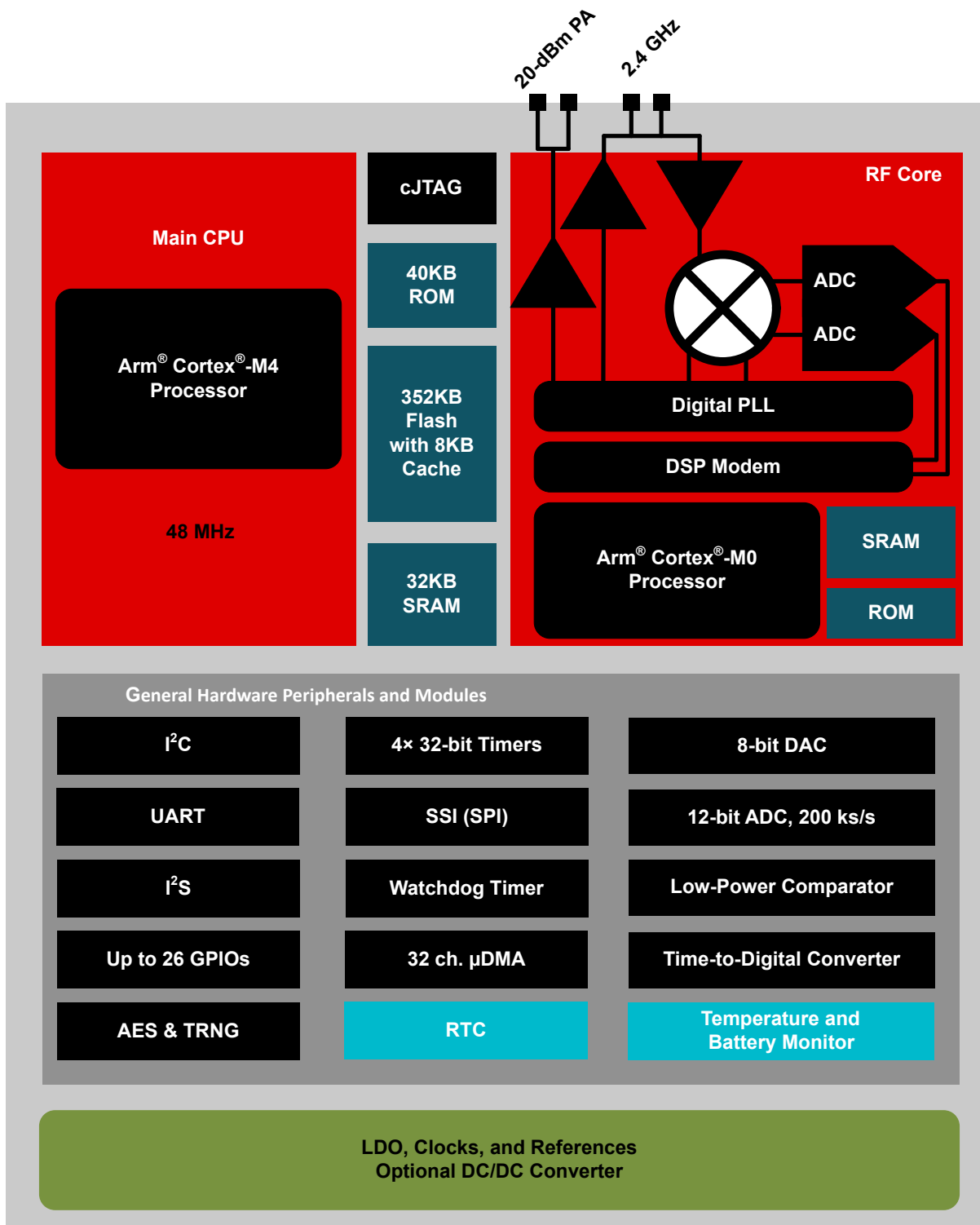
图 4-1. CC2651P3 功能方框图
