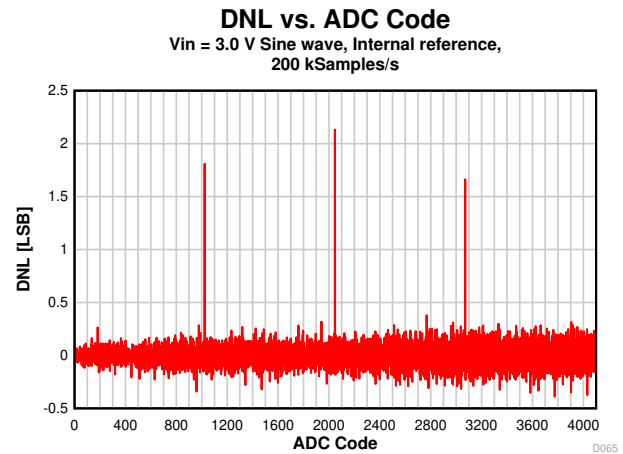
图 8-36. DNL vs. ADC Code
