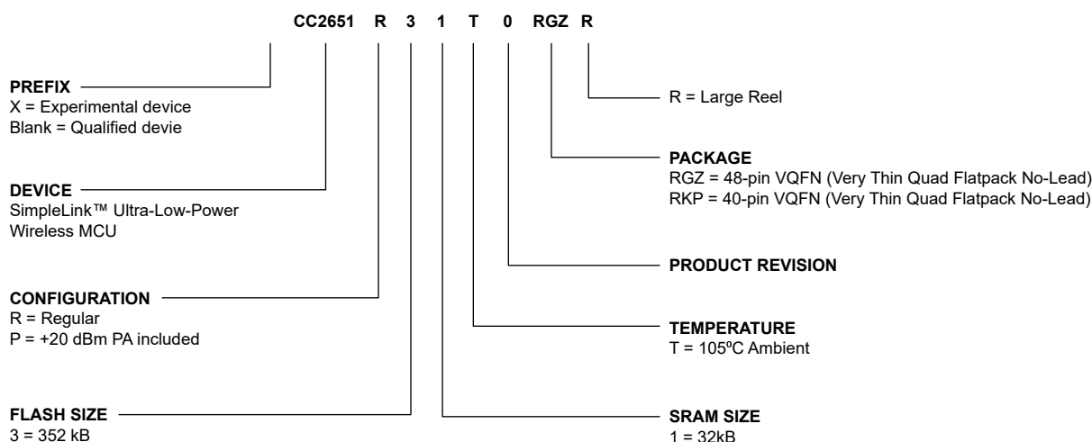
图 11-1. Device Nomenclature
