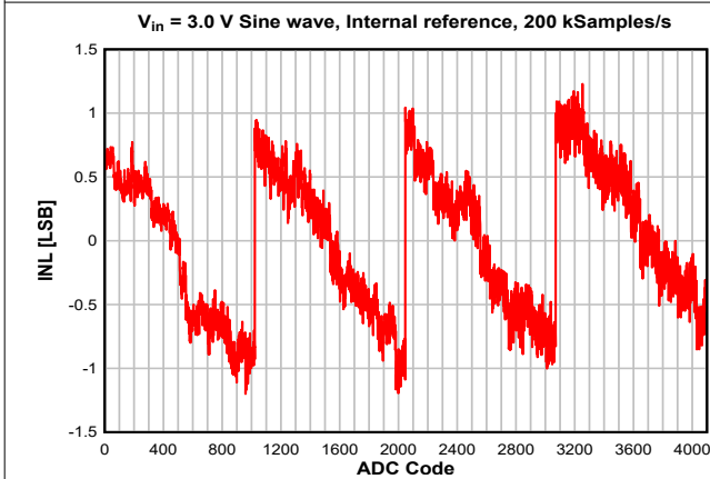
图 7-35. INL vs. ADC Code
