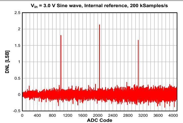
图 7-36. DNL vs. ADC Code
