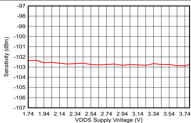
图 7-19. 灵敏度与 VDDDS 间的关系 (IEEE 802.15.4 PHY)
