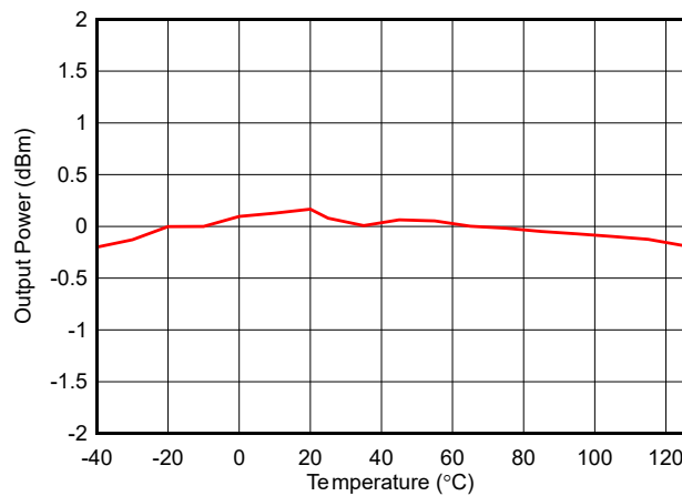
图 7-22. 输出功率与温度间的关系 ( BLE 1Mbps , 2.44GHz , 0dBm )
