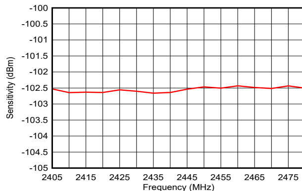
图 7-15. 灵敏度与频率间的关系 (IEEE 802.15.4 PHY)
