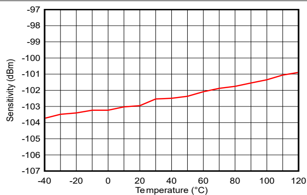
图 7-17. 灵敏度与温度间的关系 (IEEE 802.15.4 PHY)
