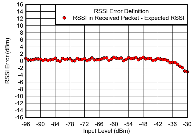
图 7-21. RSSI 误差与输入电平间的关系 (dBm)
