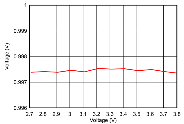
图 7-35. ADC 精度与电源电压间的关系 ( V_{IN} = 1V , 内部基准, 200ksps)
