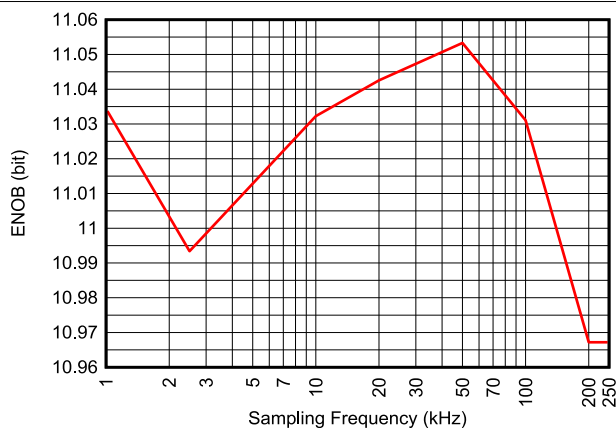
图 7-29. ENOB 与采样频率间的关系 ( V_{in} = 3V 斜坡波, 内部基准, F_{in} = F_s/10 )
