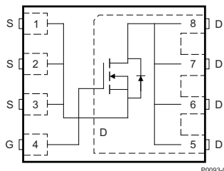
俯视图
