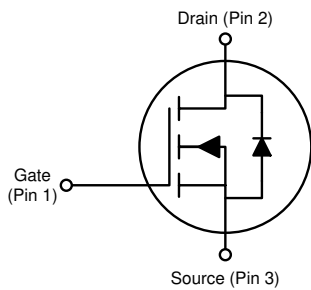
引脚排列
