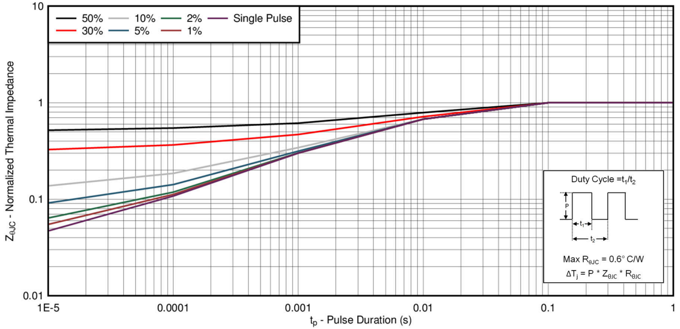
图 4-1. 瞬态热阻抗
