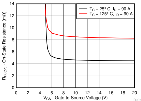
R DS(on) 与 V GS 之间的关系
