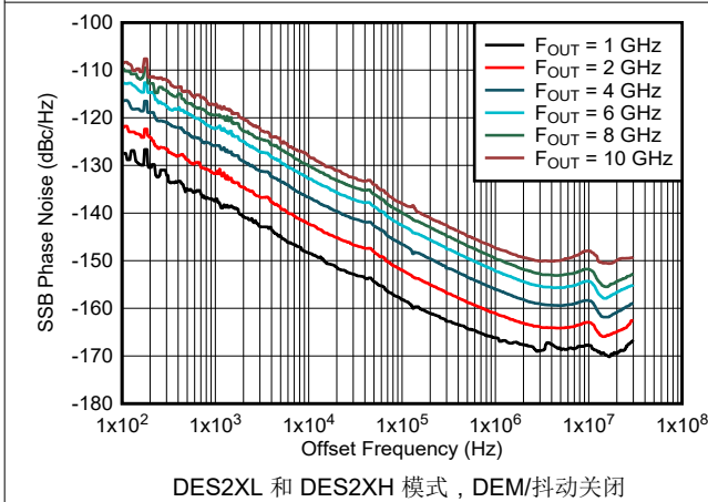
图 6-203. 相位噪声与偏移频率和输出频率间的关系
