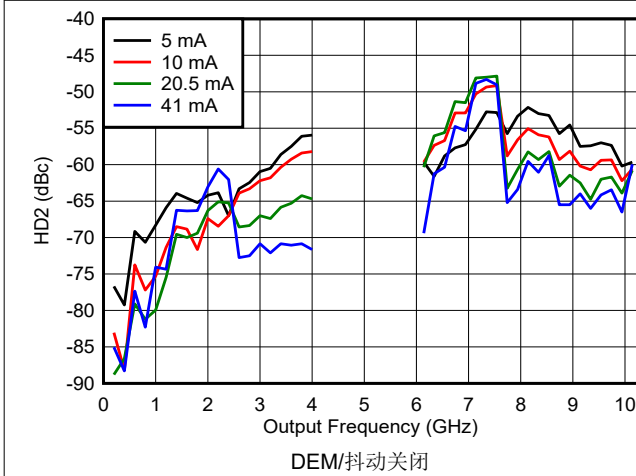
图 6-143. DES2X 模式下 HD2 与频率和输出电流间的关系
