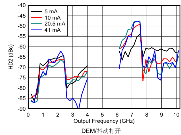
图 6-144. DES2X 模式下 HD2 与频率和输出电流间的关系
