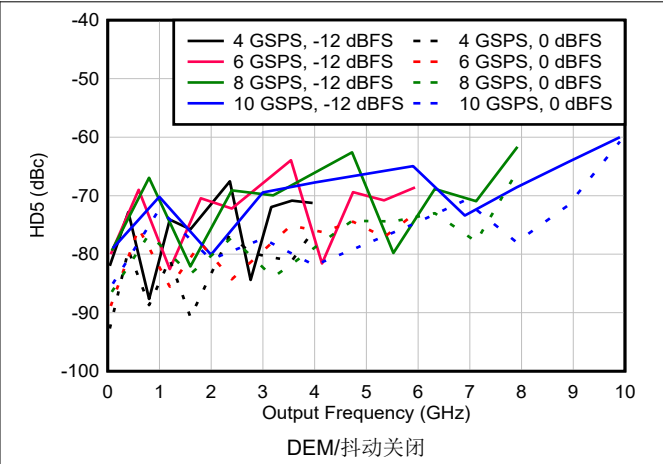
图 6-190. NRZ/RF 模式下 HD5 与频率和采样速率间的关系
