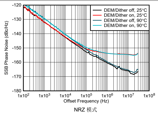
图 6-204. 1GHz 条件下相位噪声与偏移频率间的关系
