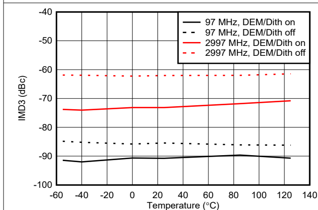
图 6-133. NRZ 模式下 IMD3 与温度间的关系
