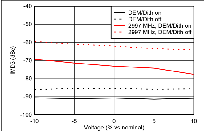
图 6-137. NRZ 模式下 IMD3 与电压间的关系
