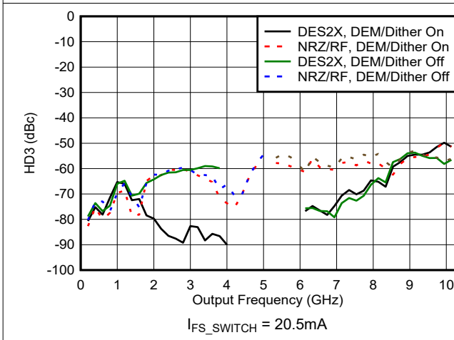
图 6-95. HD3 与频率和模式间的关系
