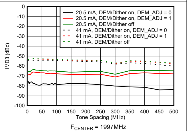
图 6-126. DES2XL 模式下 IMD3 与频率间隔间的关系
