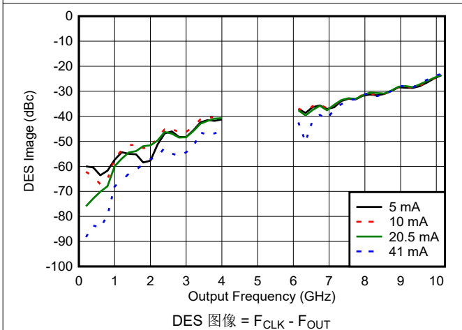
图 6-193. DES2X 模式下 DES 图像与频率和输出电流间的关系
