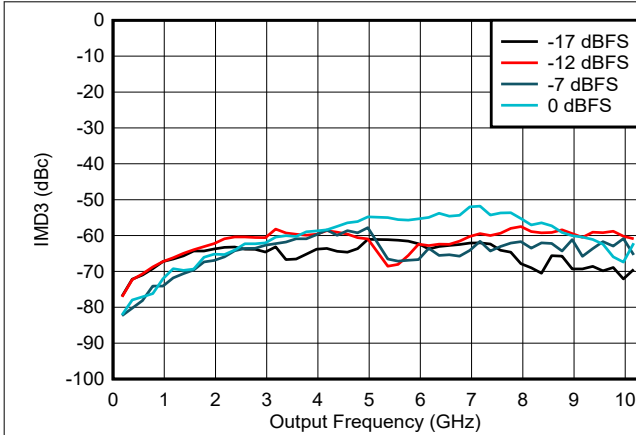
图 6-117. NRZ/RF 模式下 IMD3 与频率和数字振幅间的关系
