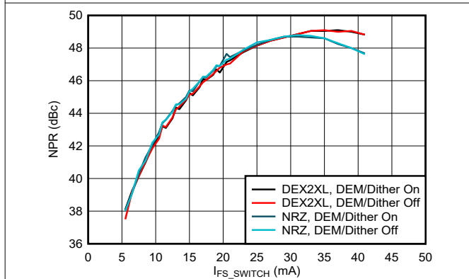
图 6-199. 电源抑制比与输出电流间的关系：第一奈奎斯特区域
