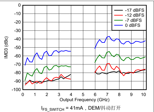
图 6-124. DES2X 模式下 IMD3 与频率和数字振幅间的关系
