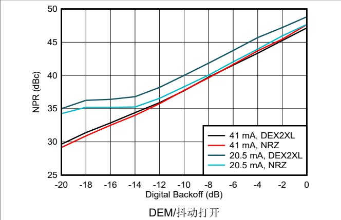
图 6-196. 噪声功率比与数字退避：第一奈奎斯特区域
