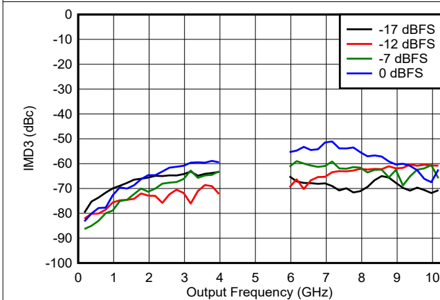
图 6-119. NRZ/RF 模式下 IMD3 与频率和数字振幅间的关系
