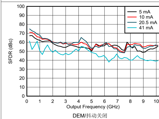
图 6-97. NRZ/RF 模式下 SFDR 与频率和输出电流间的关系
