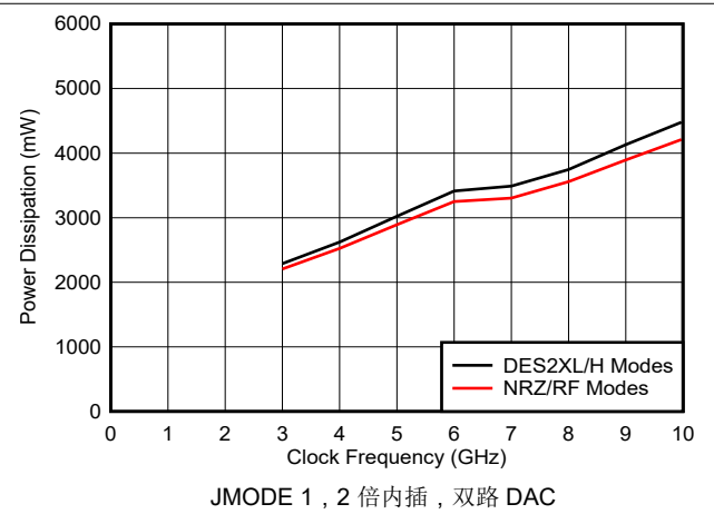
图 6-214. 功率损耗与时钟频率以及 DAC 模式间的关系
