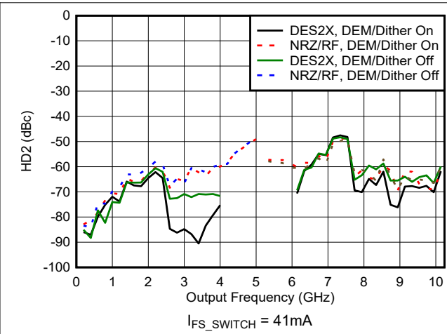
图 6-94. HD2 与频率和模式间的关系
