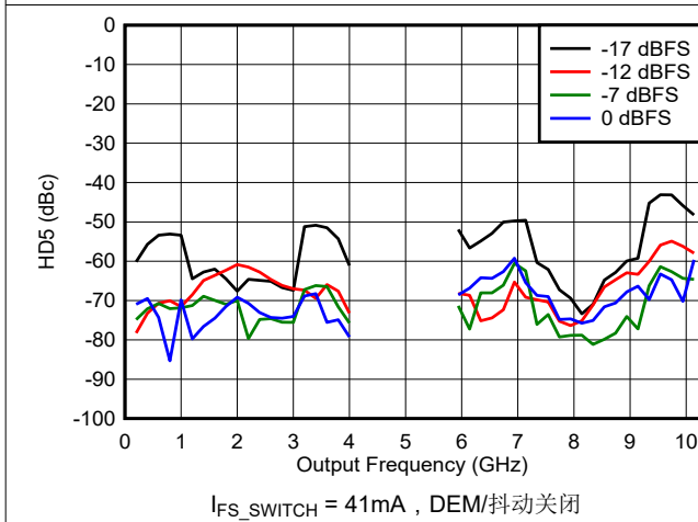
图 6-187. DES2X 模式下 HD5 与频率和数字振幅间的关系
