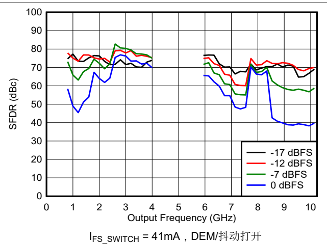
图 6-108. DES2X 模式下 SFDR 与频率和数字振幅间的关系
