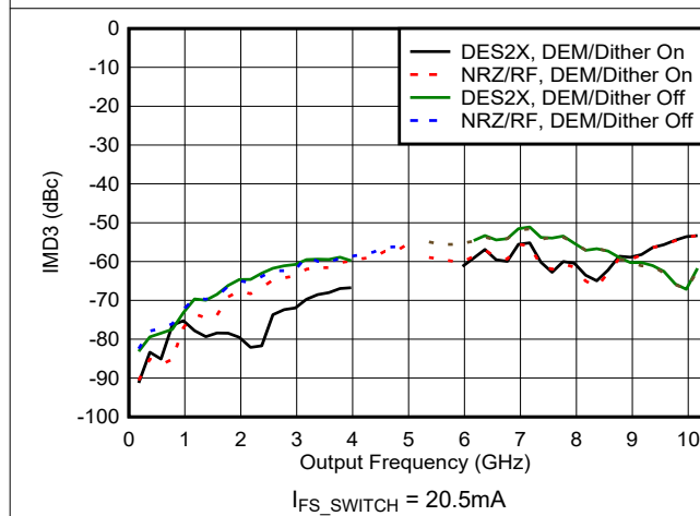
图 6-91. IMD3 与频率和模式间的关系
