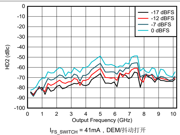
图 6-148. NRZ/RF 模式下 HD2 与频率和数字振幅间的关系
