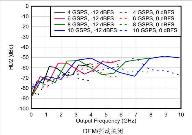
图 6-156. DES2X 模式下 HD2 与频率和采样速率间的关系
