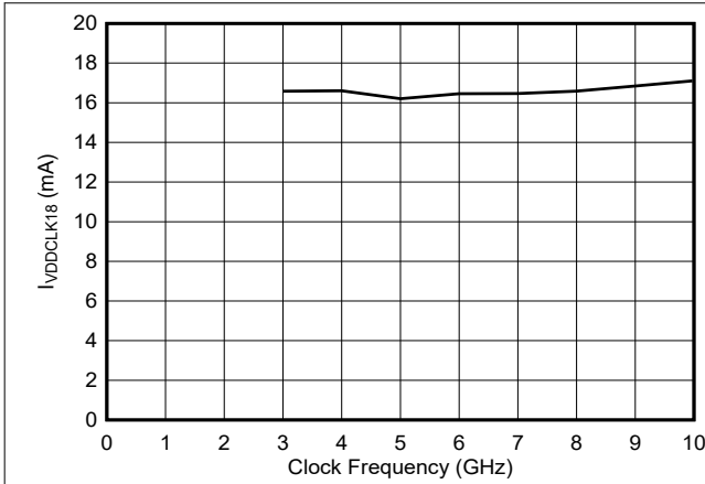
图 6-217. VDDCLK18 电流与时钟频率间的关系
