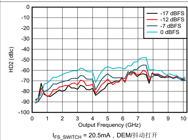
图 6-146. NRZ/RF 模式下 HD2 与频率和数字振幅间的关系
