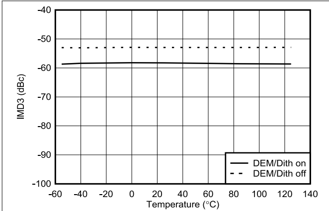
图 6-135. 7247MHz RF 模式下 IMD3 与温度间的关系
