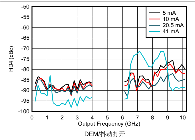
图 6-176. DES2X 模式下 HD4 与频率和输出电流间的关系
