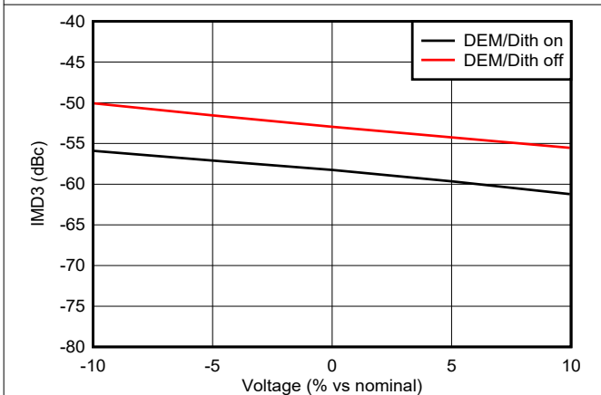
图 6-139. 7247MHz RF 模式下 IMD3 与电压间的关系
