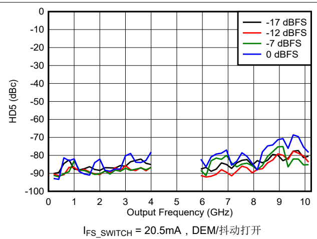
图 6-186. DES2X 模式下 HD5 与频率和数字振幅间的关系
