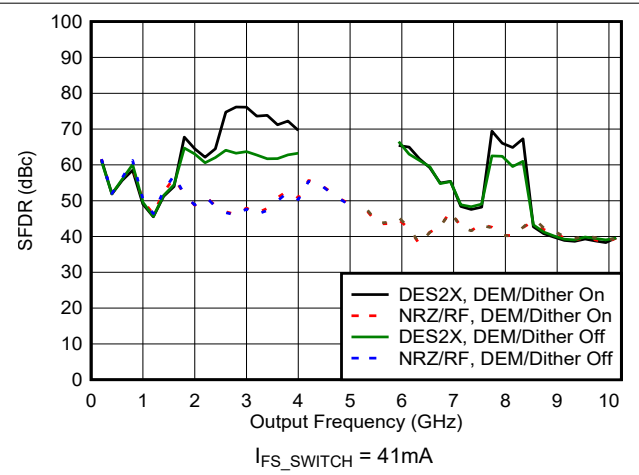
图 6-90. SFDR 与频率和模式间的关系
