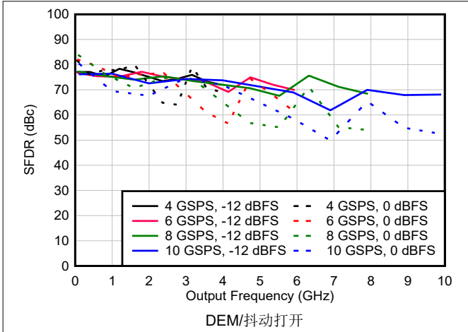
图 6-111. DES2X 模式下 SFDR 与频率和采样速率间的关系
