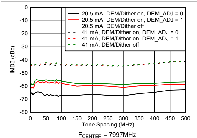
图 6-127. RF 模式下 IMD3 与频率间隔间的关系
