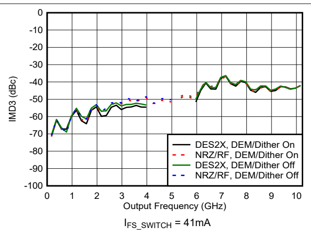
图 6-92. IMD3 与频率和模式间的关系
