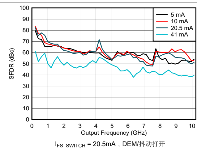
图 6-98. NRZ/RF 模式下 SFDR 与频率和输出电流间的关系
