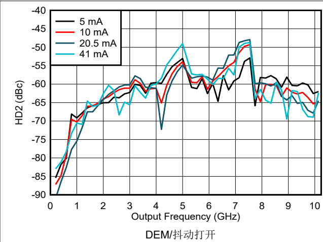
图 6-142. NRZ/RF 模式下 HD2 与频率和输出电流间的关系
