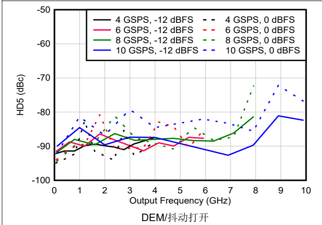
图 6-191. DES2X 模式下 HD5 与频率和采样速率间的关系
