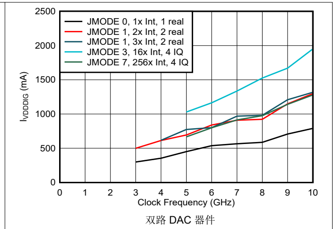
图 6-224. VDDDIG 电流与时钟频率和数字模式间的关系
