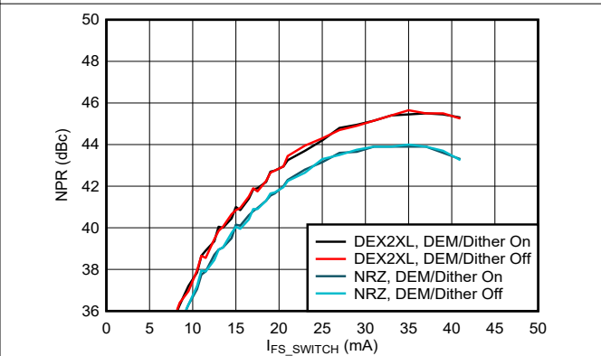
图 6-200. 电源抑制比与输出电流间的关系：第二个奈奎斯特区域
