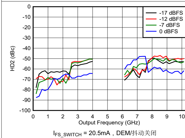
图 6-149. DES2X 模式下 HD2 与频率和数字振幅间的关系
