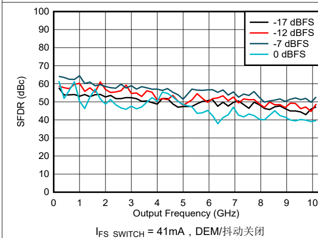
图 6-103. NRZ/RF 模式下 SFDR 与频率和数字振幅间的关系
