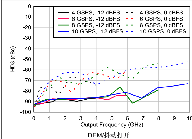
图 6-169. NRZ/RF 模式下 HD3 与频率和采样速率间的关系
