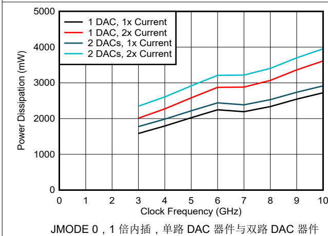
图 6-215. 功率损耗与时钟频率以及 DAC 模式间的关系
