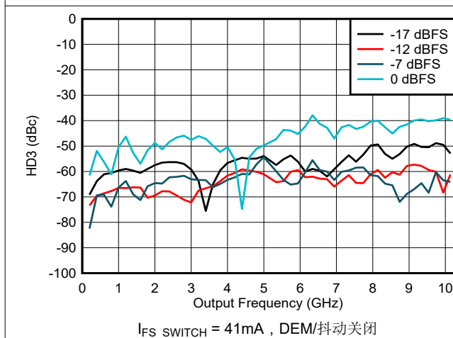
图 6-163. NRZ/RF 模式下 HD3 与频率和数字振幅间的关系
