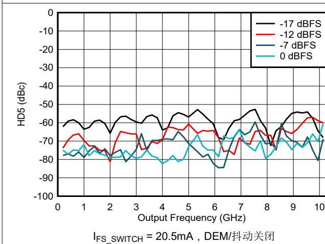
图 6-181. NRZ/RF 模式下 HD5 与频率和数字振幅间的关系
