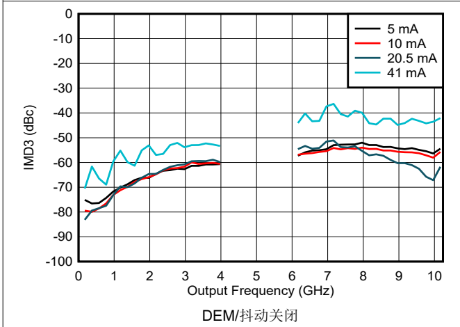
图 6-115. DES2X 模式下 IMD3 与频率和输出电流间的关系
