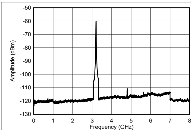
图 8-18. 0GHz 至 8GHz 频率下的 NLFM 线性调频脉冲输出频谱
