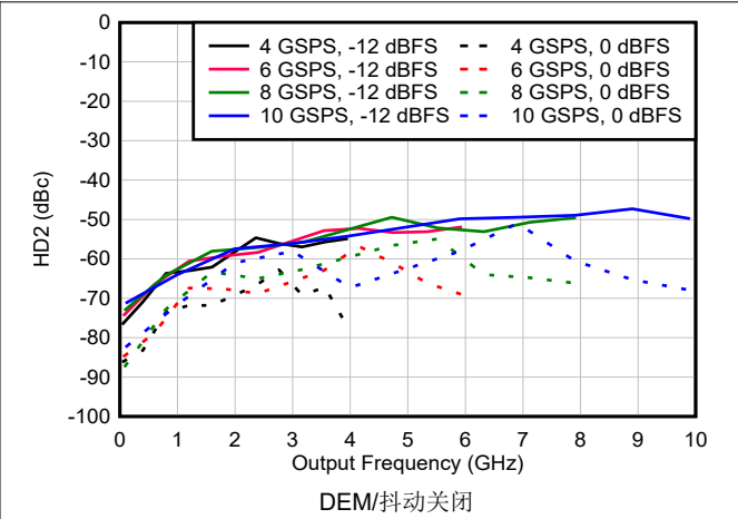
图 6-154. NRZ/RF 模式下 HD2 与频率和采样速率间的关系
