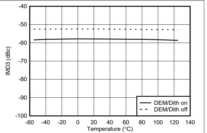
图 6-136. 7247MHz DES2XH 模式下 IMD3 与温度间的关系
