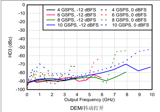
图 6-171. DES2X 模式下 HD3 与频率和采样速率间的关系
