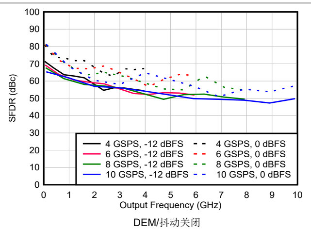
图 6-110. NRZ/RF 模式下 SFDR 与频率和采样速率间的关系
