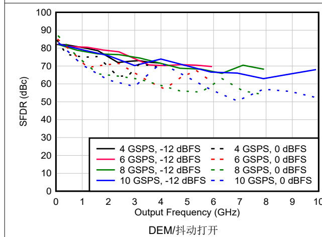
图 6-109. NRZ/RF 模式下 SFDR 与频率和采样速率间的关系
