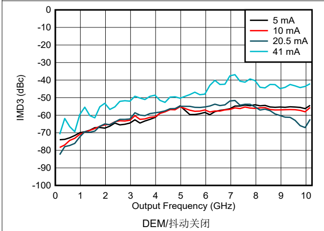
图 6-113. NRZ/RF 模式下 IMD3 与频率和输出电流间的关系
