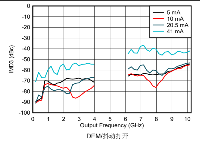
图 6-116. DES2X 模式下 IMD3 与频率和输出电流间的关系
