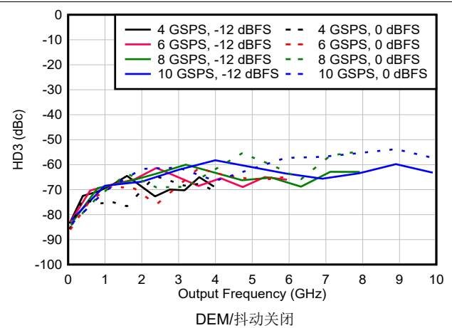
图 6-170. NRZ/RF 模式下 HD3 与频率和采样速率间的关系
