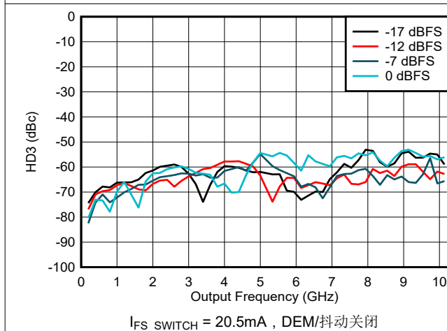
图 6-161. NRZ/RF 模式下 HD3 与频率和数字振幅间的关系
