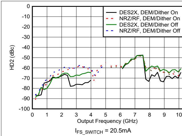
图 6-93. HD2 与频率和模式间的关系
