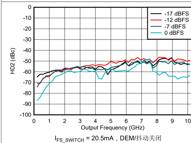
图 6-145. NRZ/RF 模式下 HD2 与频率和数字振幅间的关系
