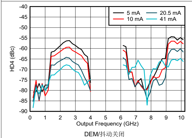
图 6-175. DES2X 模式下 HD4 与频率和输出电流间的关系
