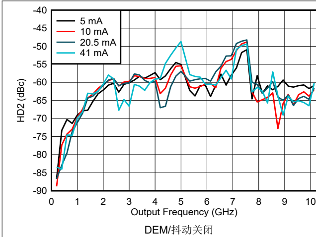
图 6-141. NRZ/RF 模式下 HD2 与频率和输出电流间的关系
