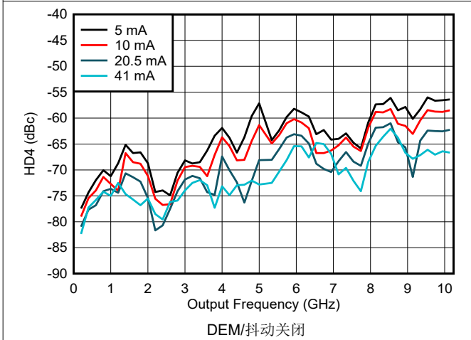
图 6-173. NRZ/RF 模式下 HD4 与频率和输出电流间的关系
