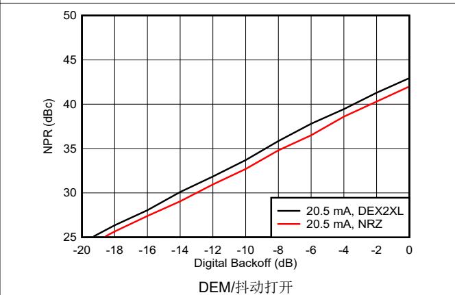
图 6-198. 噪声功率比与数字退避：第二个奈奎斯特区域
