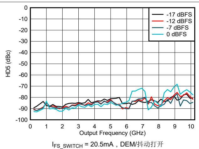
图 6-182. NRZ/RF 模式下 HD5 与频率和数字振幅间的关系
