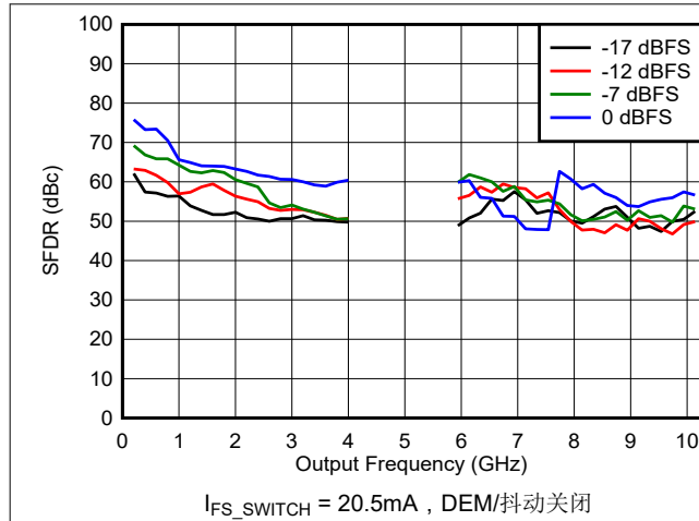
图 6-105. DES2X 模式下 SFDR 与频率和数字振幅间的关系
