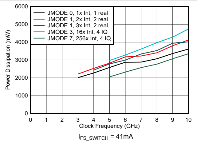
图 6-212. 功率损耗与时钟频率和数字模式间的关系
