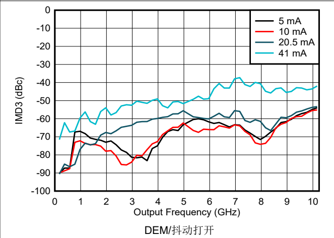
图 6-114. NRZ/RF 模式下 IMD3 与频率和输出电流间的关系
