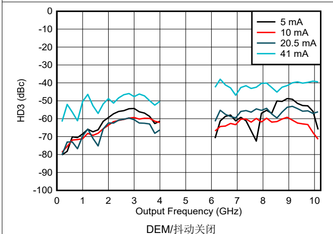
图 6-157. NRZ/RF 模式下 HD3 与频率和输出电流间的关系
