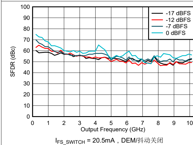
图 6-101. NRZ/RF 模式下 SFDR 与频率和数字振幅间的关系
