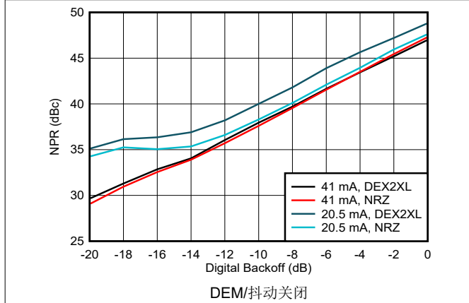
图 6-195. 噪声功率比与数字退避：第一奈奎斯特区域
