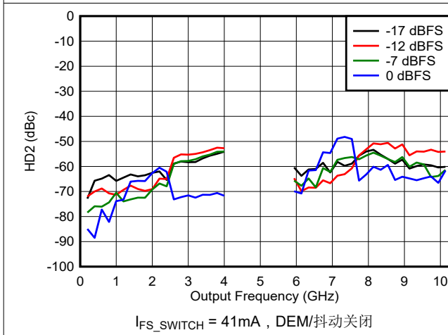
图 6-151. DES2X 模式下 HD2 与频率和数字振幅间的关系
