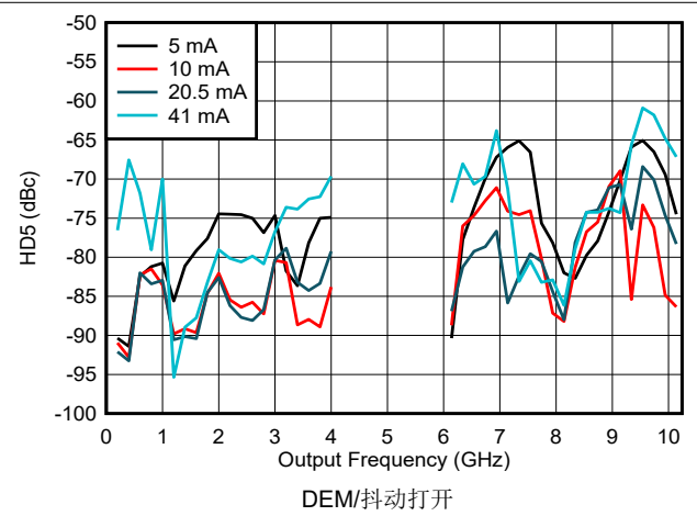
图 6-180. DES2X 模式下 HD5 与频率和输出电流间的关系
