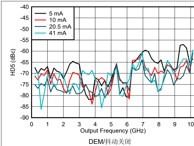
图 6-177. NRZ/RF 模式下 HD5 与频率和输出电流间的关系
