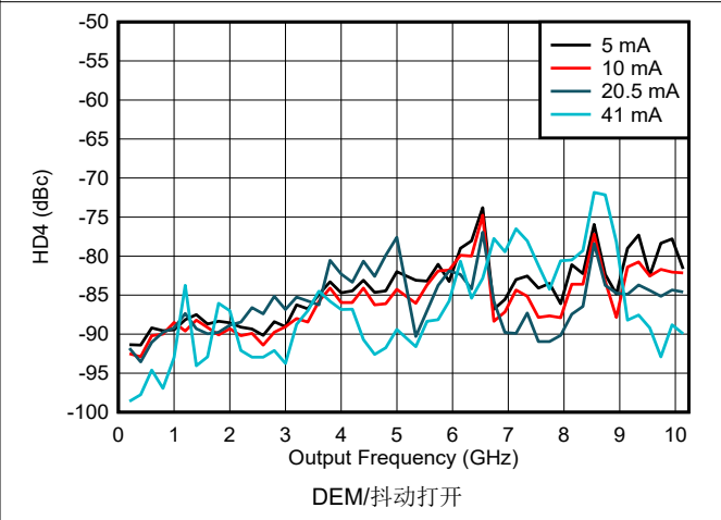
图 6-174. NRZ/RF 模式下 HD4 与频率和输出电流间的关系
