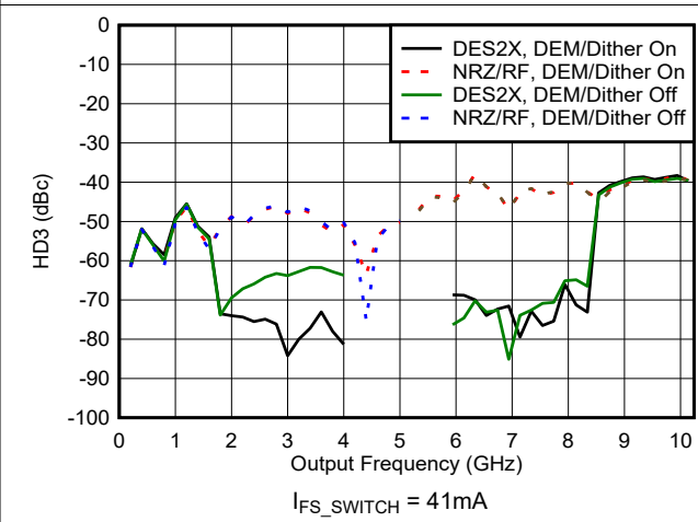
图 6-96. HD3 与频率和模式间的关系
