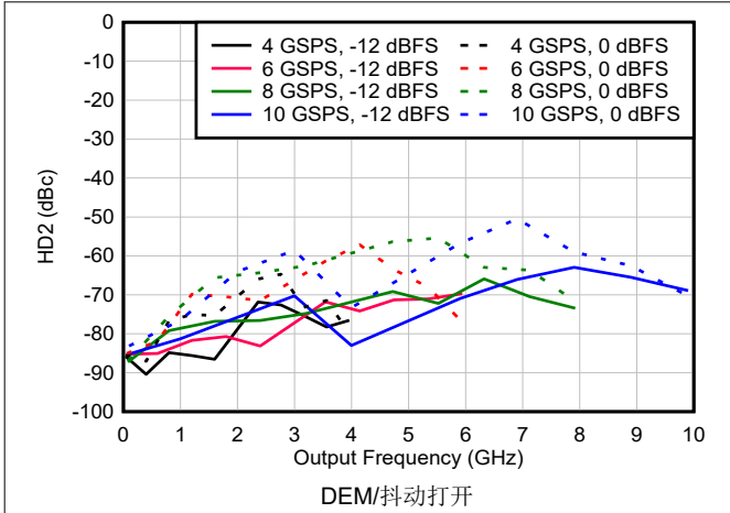
图 6-153. NRZ/RF 模式下 HD2 与频率和采样速率间的关系
