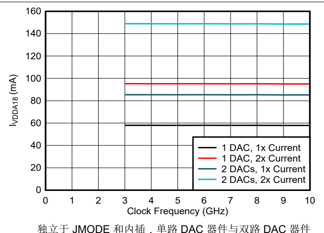
图 6-216. VDDA18 电流与时钟频率和 DAC 模式间的关系
