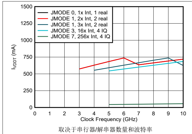
图 6-223. VDDT 电流与时钟频率和模式间的关系
