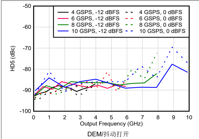
图 6-189. NRZ/RF 模式下 HD5 与频率和采样速率间的关系
