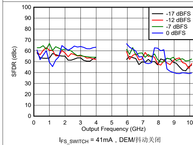
图 6-107. DES2X 模式下 SFDR 与频率和数字振幅间的关系
