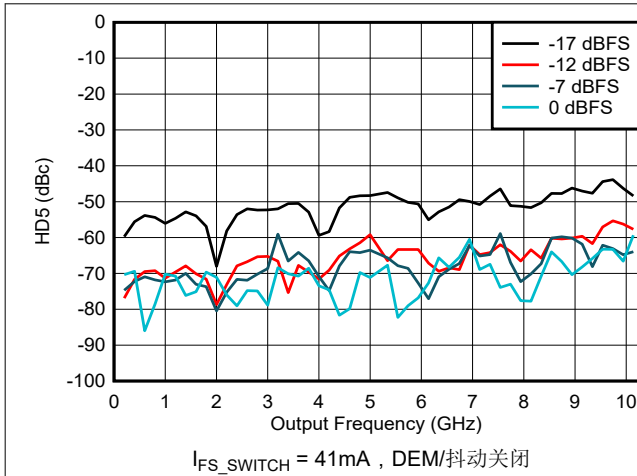
图 6-183. NRZ/RF 模式下 HD5 与频率和数字振幅间的关系
