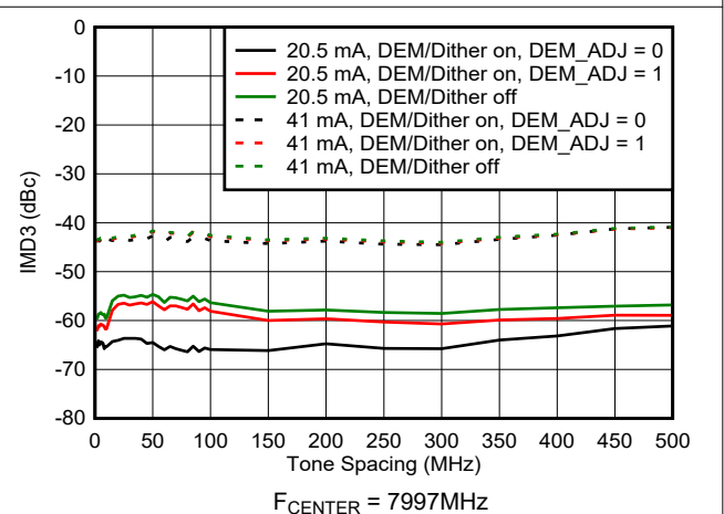
图 6-128. DES2XH 模式下 IMD3 与频率间隔间的关系
