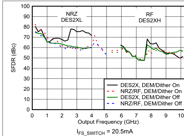
图 6-89. SFDR 与频率和模式间的关系
