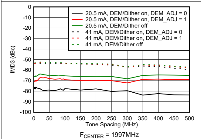
图 6-125. NRZ 模式下 IMD3 与频率间隔间的关系
