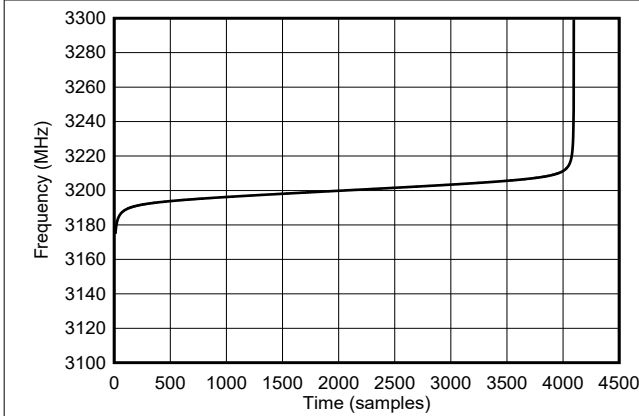
图 8-14. NLFM 频率斜升
