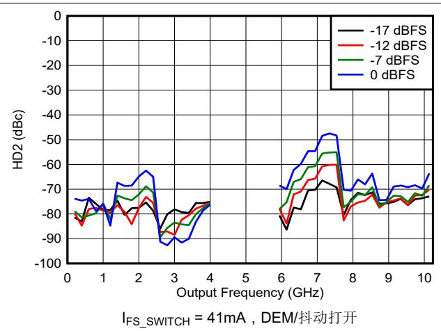
图 6-152. DES2X 模式下 HD2 与频率和数字振幅间的关系
