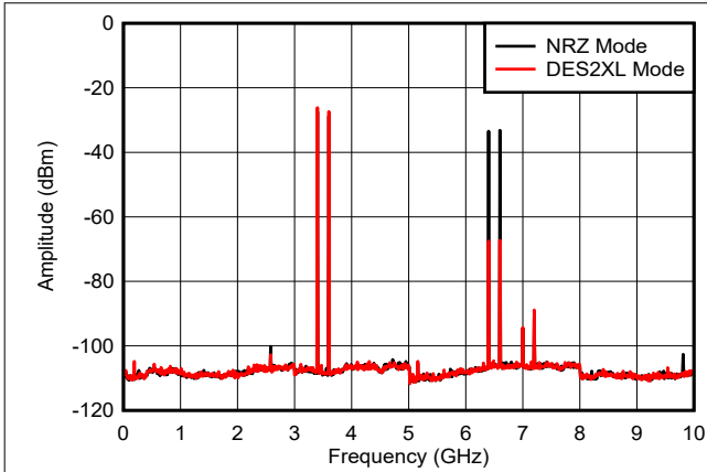
图 6-51. 双音， f_{\text{OUT}} = 3497\text{ MHz} ，-12dBFS
