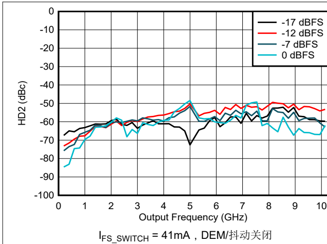
图 6-147. NRZ/RF 模式下 HD2 与频率和数字振幅间的关系
