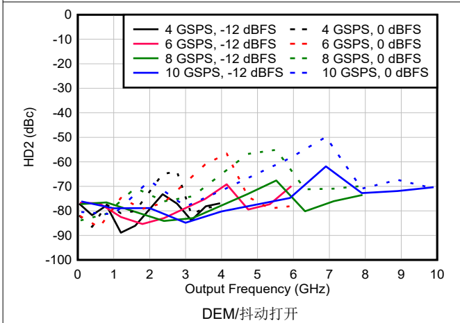
图 6-155. DES2X 模式下 HD2 与频率和采样速率间的关系
