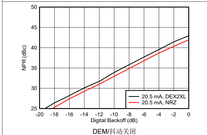
图 6-197. 噪声功率比与数字退避：第二个奈奎斯特区域
