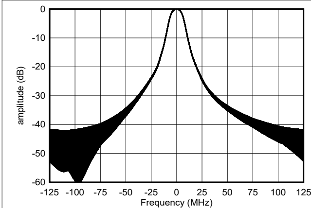
图 8-16. NLFM 线性调频脉冲的数字频谱
