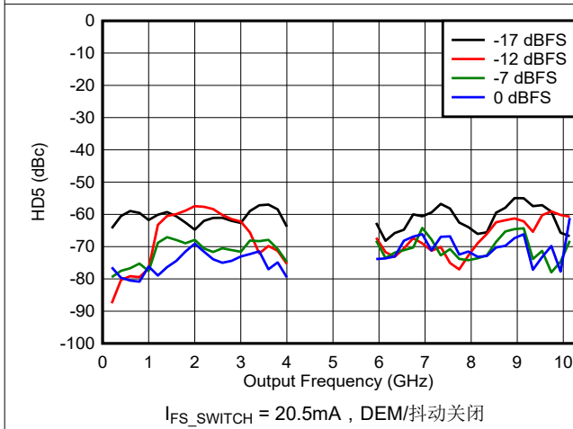
图 6-185. DES2X 模式下 HD5 与频率和数字振幅间的关系
