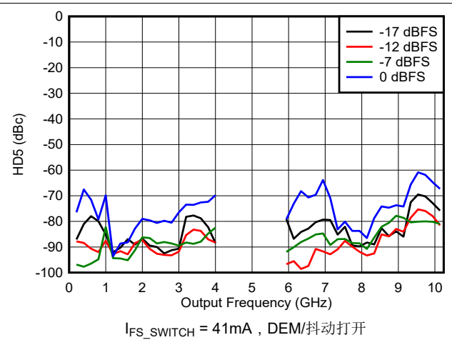
图 6-188. DES2X 模式下 HD5 与频率和数字振幅间的关系
