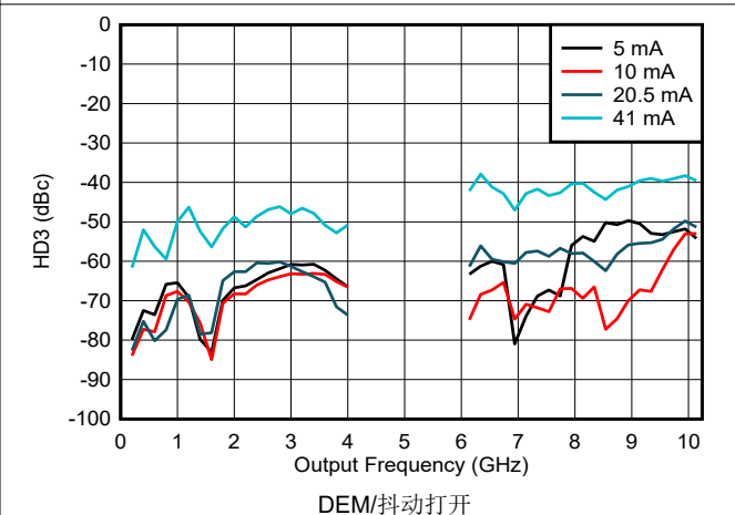
图 6-158. NRZ/RF 模式下 HD3 与频率和输出电流间的关系
