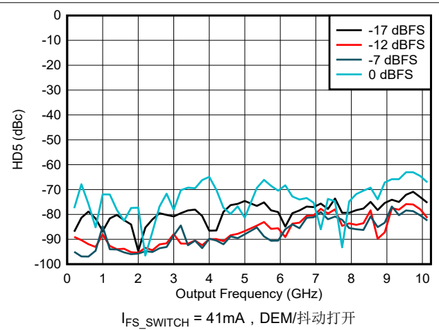
图 6-184. NRZ/RF 模式下 HD5 与频率和数字振幅间的关系
