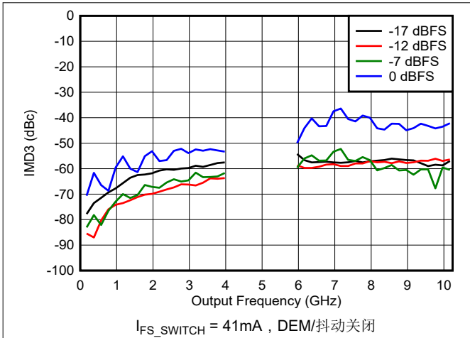
图 6-123. DES2X 模式下 IMD3 与频率和数字振幅间的关系
