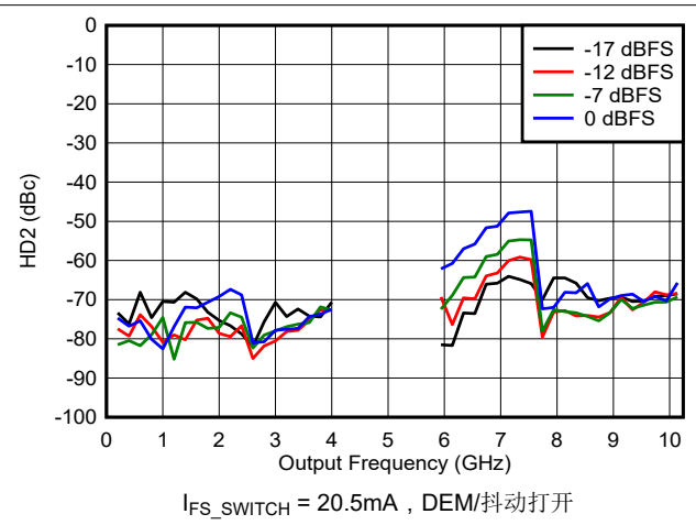
图 6-150. DES2X 模式下 HD2 与频率和数字振幅间的关系
