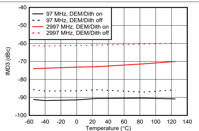
图 6-134. DES2XL 模式下 IMD3 与温度间的关系
