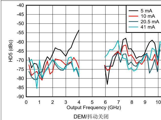
图 6-179. DES2X 模式下 HD5 与频率和输出电流间的关系
