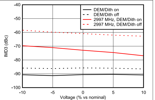
图 6-138. DES2XL 模式下 IMD3 与电压间的关系
