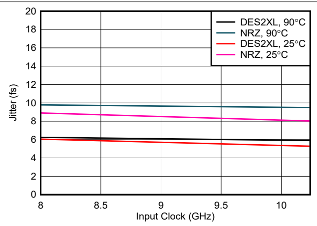
图 6-206. 抖动与输入时钟间的关系
