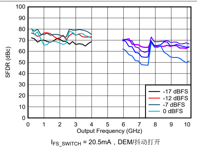
图 6-106. DES2X 模式下 SFDR 与频率和数字振幅间的关系
