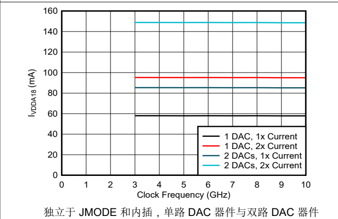
图 6-94. VDDA18 电流与时钟频率和 DAC 模式间的关系
