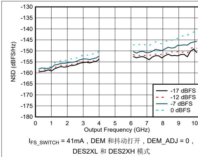
图 6-74. NSD 与输出频率和数字振幅间的关系
