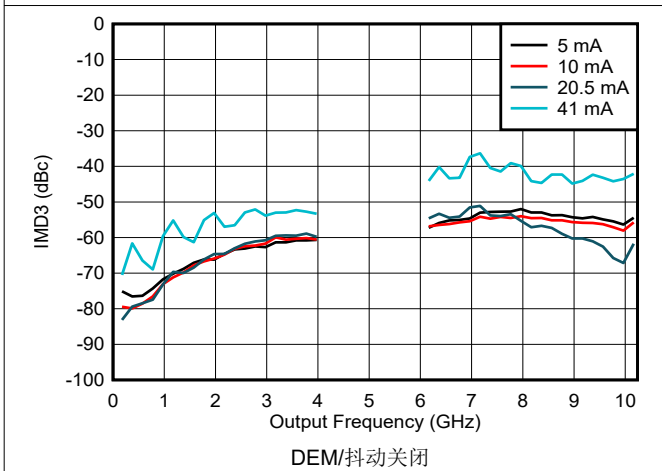
图 6-130. DES2X 模式下 IMD3 与频率和输出电流间的关系
