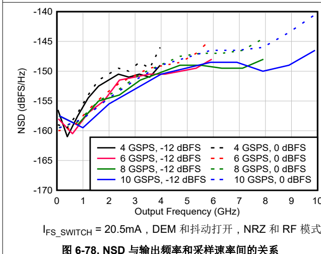
图 6-78. NSD 与输出频率和采样速率间的关系
