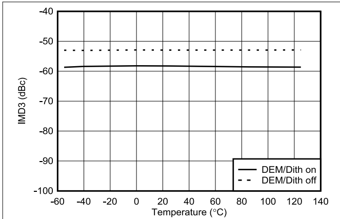
图 6-150. 7247MHz RF 模式下 IMD3 与温度间的关系
