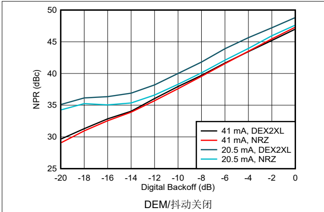
图 6-210. 噪声功率比与数字退避间的关系：第一奈奎斯特区域
