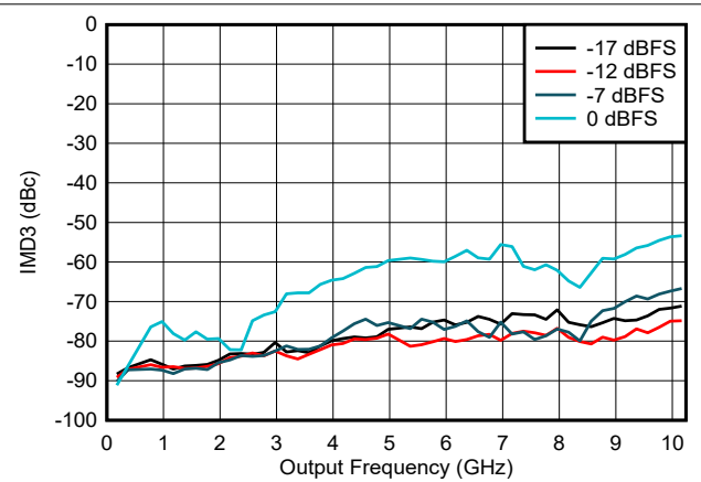
图 6-133. NRZ/RF 模式下 IMD3 与频率和数字振幅间的关系
