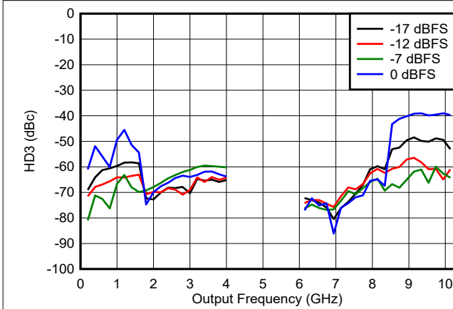
图 6-180. DES2X 模式下 HD3 与频率和数字振幅间的关系
