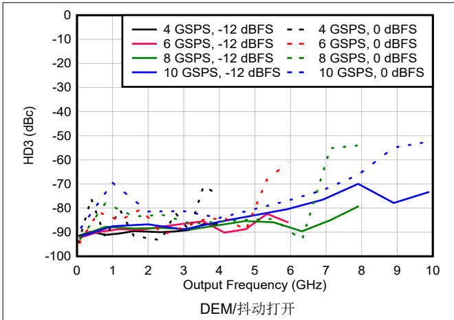
图 6-186. DES2X 模式下 HD3 与频率和采样速率间的关系
