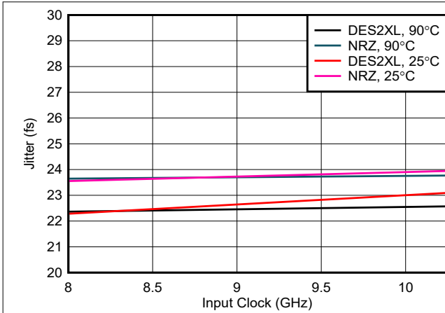
图 6-222. 抖动与输入时钟间的关系
