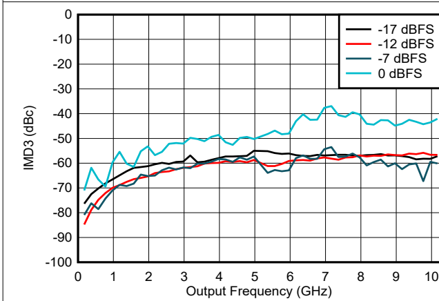
图 6-132. NRZ/RF 模式下 IMD3 与频率和数字振幅间的关系
