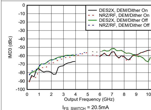
图 6-106. IMD3 与频率和模式间的关系
