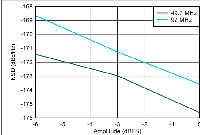
I_{\text{FS\_SWITCH}} = 41\text{mA} , DES2XL, DEM/抖动关闭 图 6-60. 低频条件下 NSD 与数字振幅间的关系
