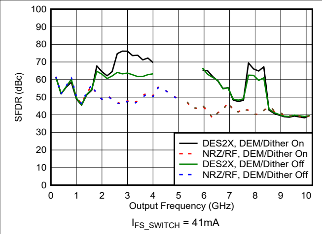
图 6-105. SFDR 与频率和模式间的关系
