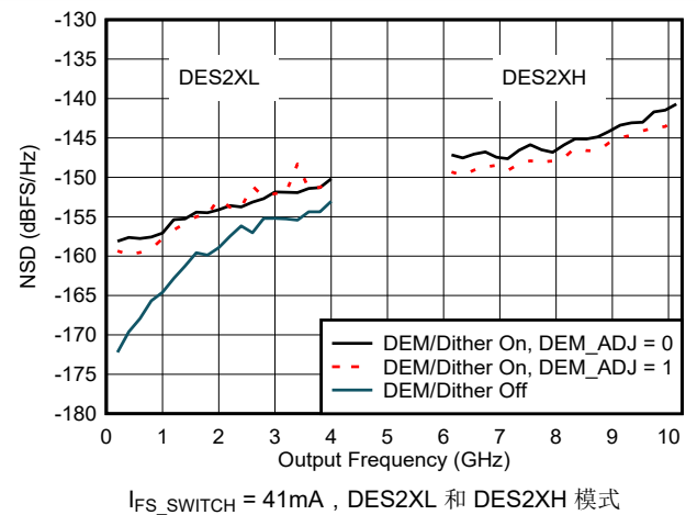
I_{\text{FS\_SWITCH}} = 41\text{mA} , DES2XL 和 DES2XH 模式 图 6-59. NSD 与输出频率和 DEM/抖动模式间的关系
