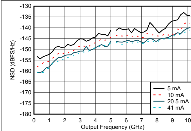
图 6-62. NSD 与输出频率和输出电流间的关系
