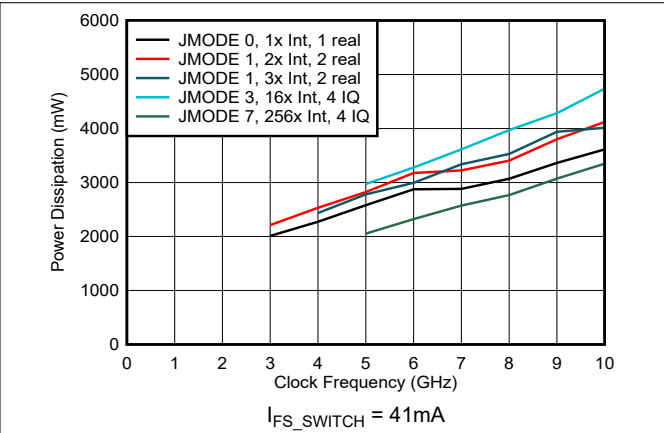
图 6-90. 功率损耗与时钟频率和数字模式间的关系
