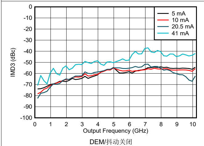
图 6-128. NRZ/RF 模式下 IMD3 与频率和输出电流间的关系
