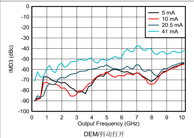
图 6-129. NRZ/RF 模式下 IMD3 与频率和输出电流间的关系
