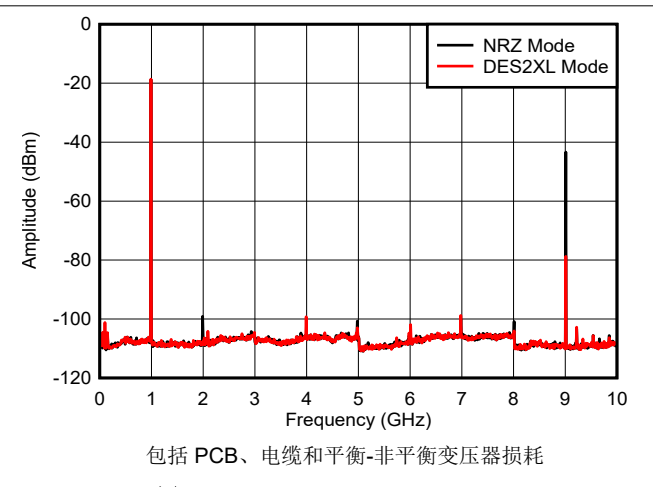
图 6-24. f_{\text{OUT}} = 997\text{MHz} ，-12dBFS
