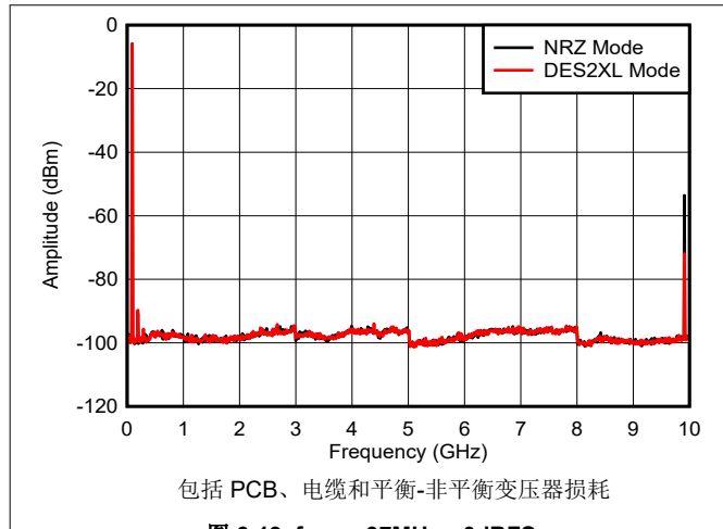
图 6-19. f_{\text{OUT}} = 97\text{MHz} ，0dBFS
