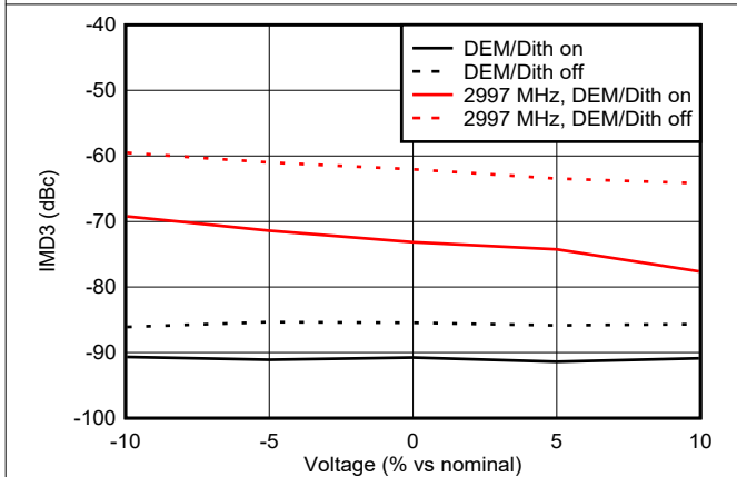
图 6-152. NRZ 模式下 IMD3 与电压间的关系
