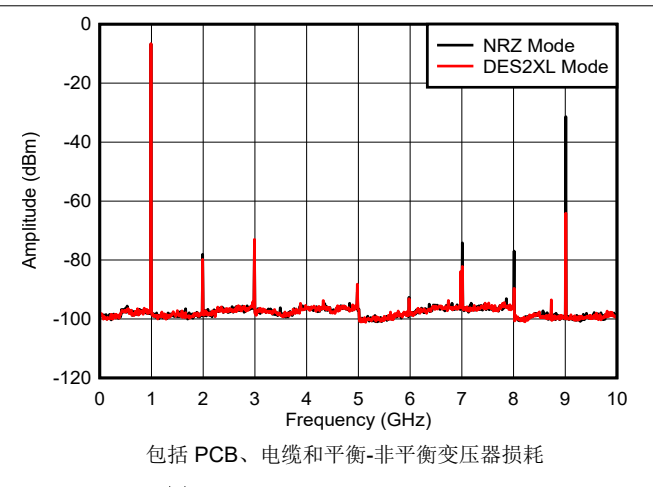
图 6-22. f_{\text{OUT}} = 997\text{MHz} ，0dBFS
