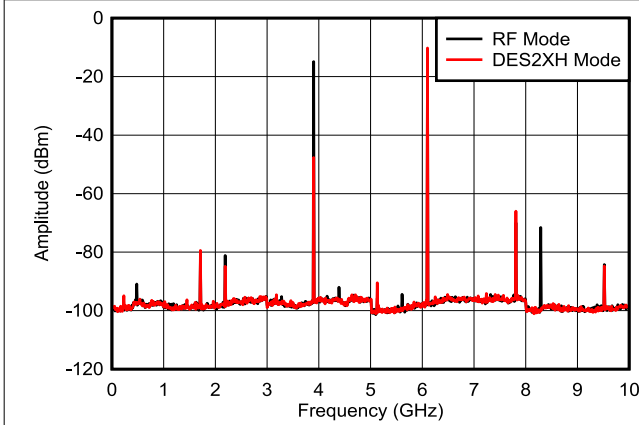
图 6-31. f_{\text{OUT}} = 6097\text{MHz} ，0dBFS
