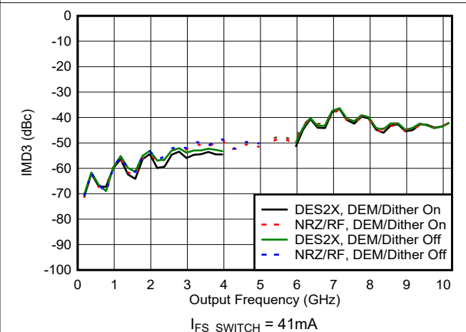
图 6-107. IMD3 与频率和模式间的关系
