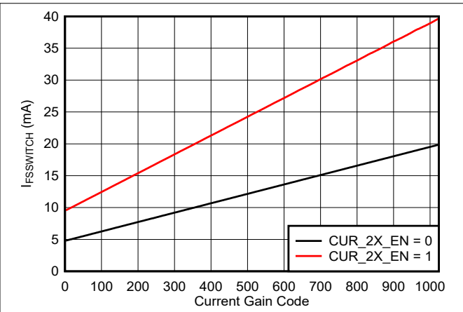
图 6-15. I_{\text{FS\_SWITCH}} 与增益代码间的关系
