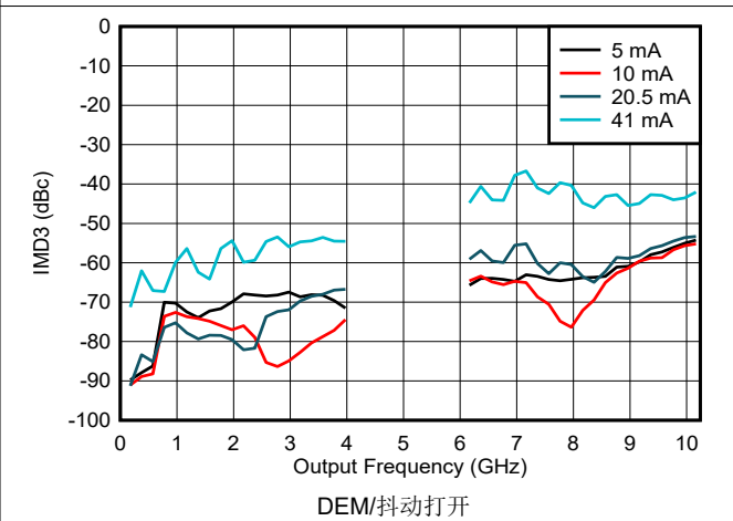
图 6-131. DES2X 模式下 IMD3 与频率和输出电流间的关系
