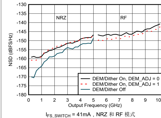
I_{\text{FS\_SWITCH}} = 41\text{mA} , NRZ 和 RF 模式 图 6-58. NSD 与输出频率和 DEM/抖动模式间的关系
