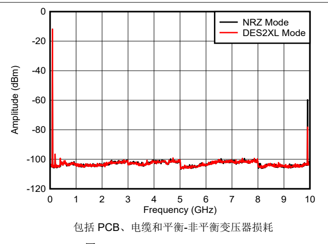
图 6-20. f_{\text{OUT}} = 97\text{MHz} ，-6dBFS
