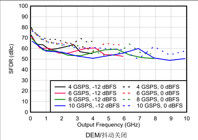
图 6-127. DES2X 模式下 SFDR 与频率和采样速率间的关系
