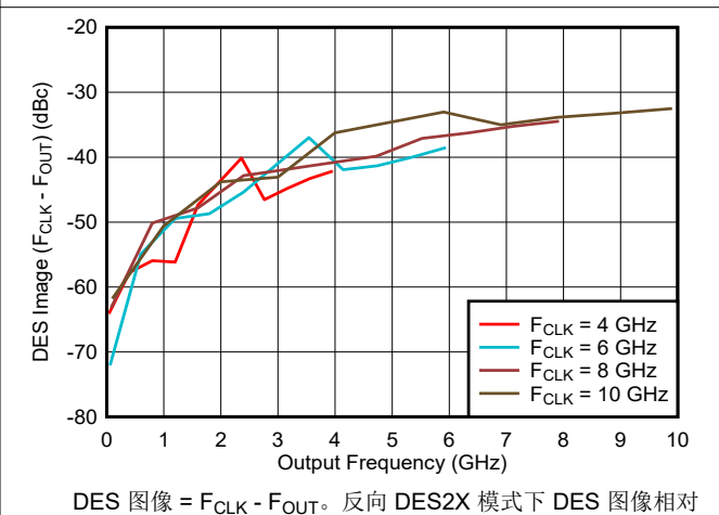
图 6-209. DES2X 模式下 DES 图像与频率和采样速率间的关系
