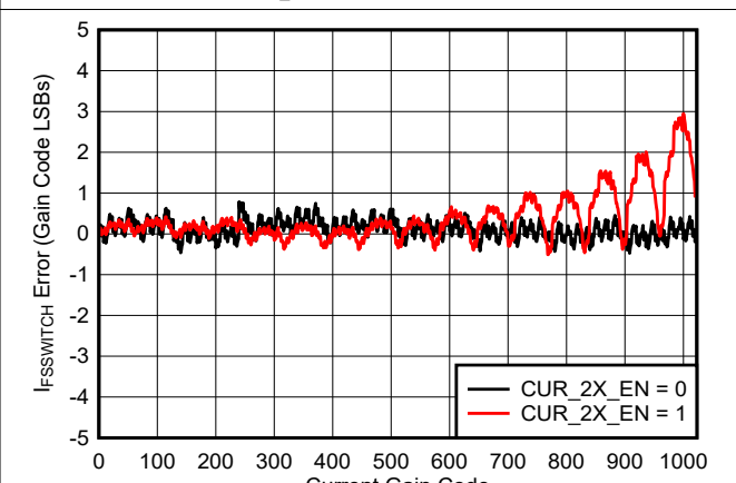
图 6-15. I_{\text{FS\_SWITCH}} 与增益代码间的关系
