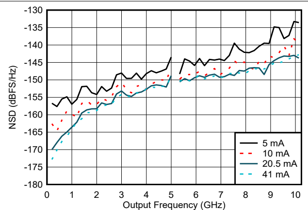
DEM 和抖动关闭, NRZ 和 RF 模式 图 6-61. NSD 与输出频率和输出电流间的关系
