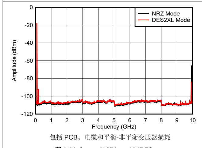
图 6-21. f_{\text{OUT}} = 97\text{MHz} ，-12dBFS
