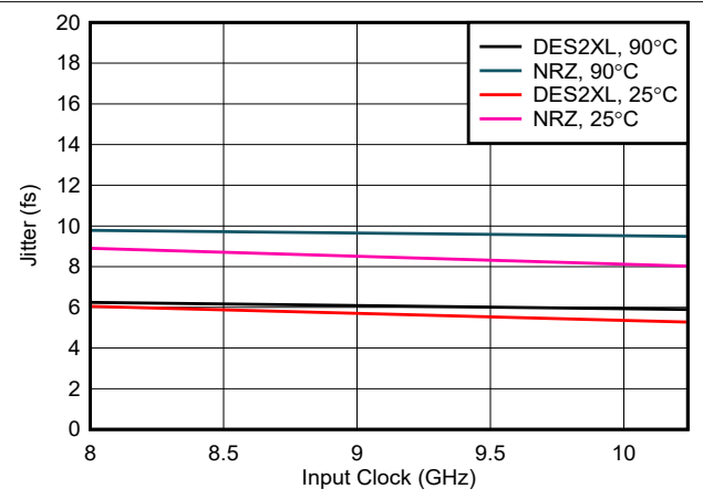
图 6-221. 抖动与输入时钟间的关系
