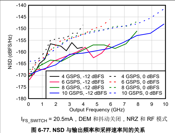
图 6-77. NSD 与输出频率和采样速率间的关系
