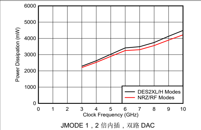
图 6-92. 功率损耗与时钟频率和 DAC 模式间的关系
