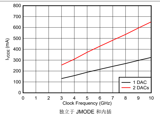
图 6-51. VDDDE 电流与时钟频率间的关系
