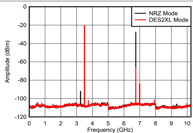
图 6-17. f_{\text{OUT}} = 3497\text{MHz} ， 0\text{dBFS}
