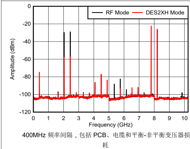
图 6-42. 双音， f_{\text{OUT}} = 7997\text{MHz} ， -6\text{dBFS}
