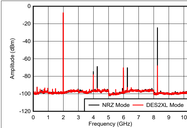
图 6-14. f_{\text{OUT}} = 1997\text{MHz} ，0dBFS
