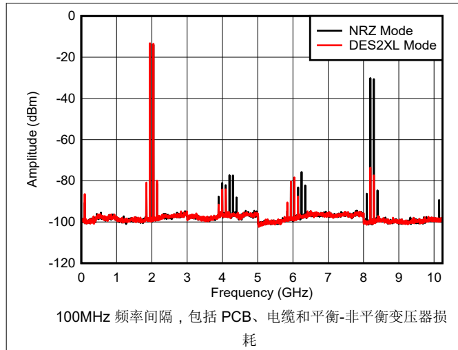
图 6-32. 双音， f_{\text{OUT}} = 1997\text{MHz} ，0dBFS
