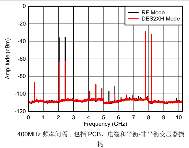
图 6-43. 双音， f_{\text{OUT}} = 7997\text{MHz} ， -12\text{dBFS}
