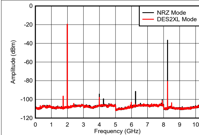
图 6-14. f_{\text{OUT}} = 1997\text{MHz} ， 0\text{dBFS}
