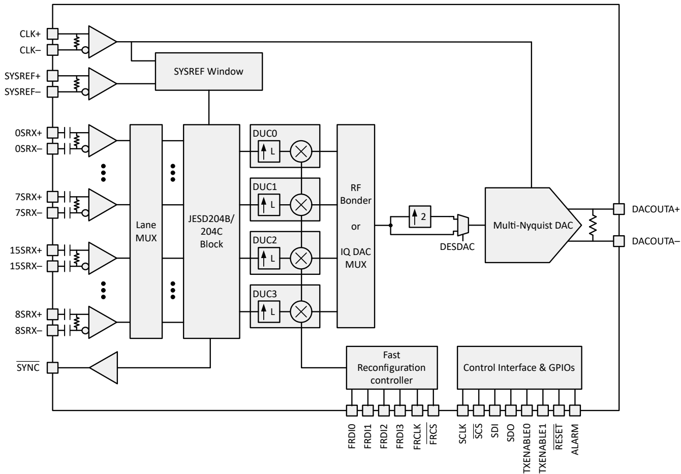
图 7-2. 单通道器件
