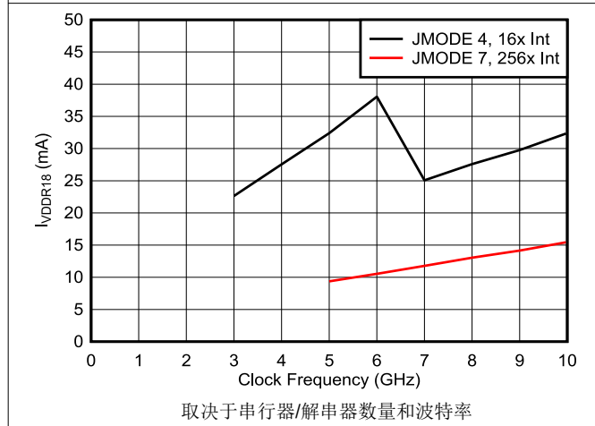
图 6-52. VDDR18 电流与时钟频率和接口模式间的关系
