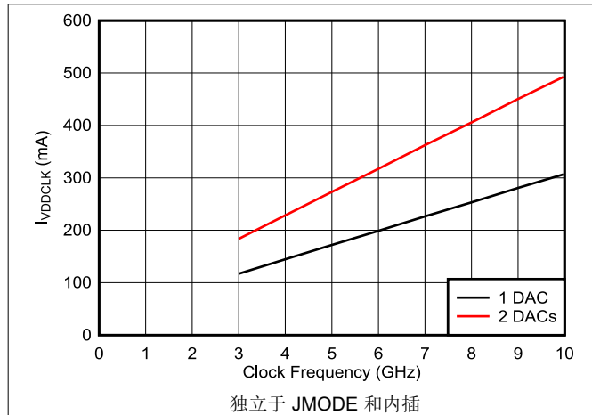
图 6-50. VDDCLK 电流与时钟频率间的关系
