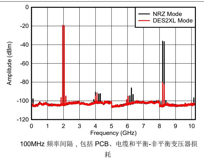
图 6-33. 双音， f_{\text{OUT}} = 1997\text{MHz} ，-6dBFS
