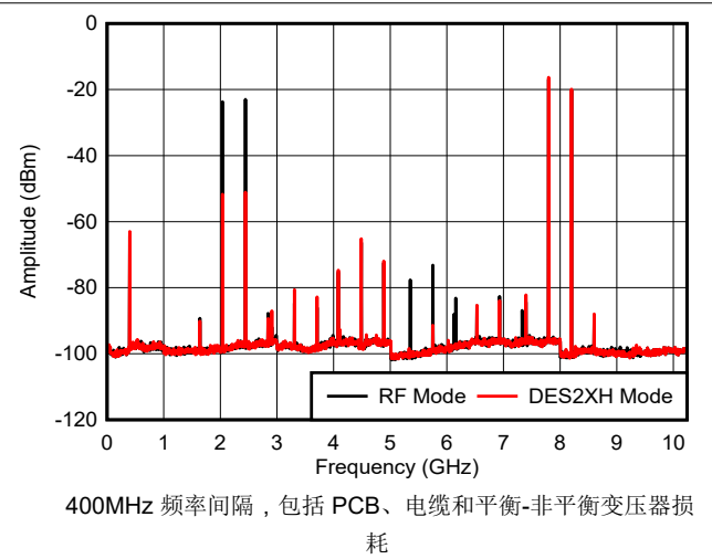
图 6-41. 双音， f_{\text{OUT}} = 7997\text{MHz} ， 0\text{dBFS}
