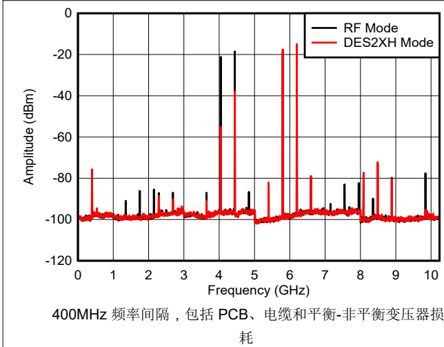
图 6-38. 双音， f_{\text{OUT}} = 5997\text{MHz} ， 0\text{dBFS}
