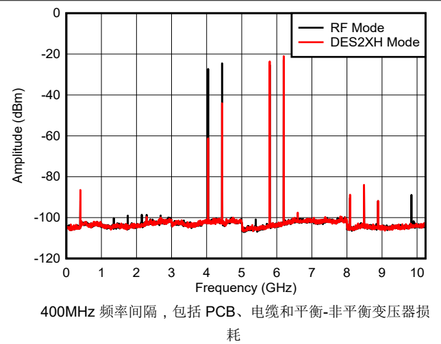
图 6-39. 双音， f_{\text{OUT}} = 5997\text{MHz} ， -6\text{dBFS}
