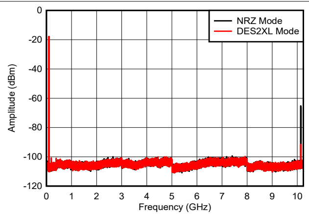
图 6-27. 双音， f_{\text{OUT}} = 97\text{MHz} ，-6dBFS
