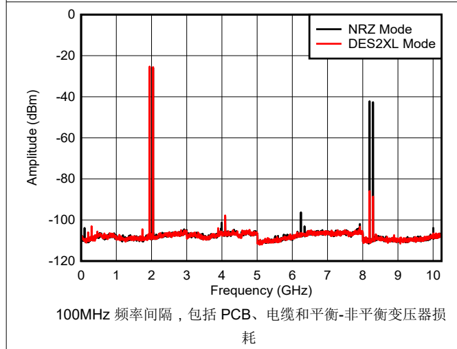
图 6-34. 双音， f_{\text{OUT}} = 1997\text{MHz} ，-12dBFS
