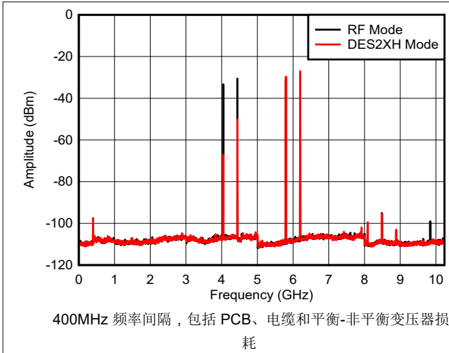
图 6-40. 双音， f_{\text{OUT}} = 5997\text{MHz} ， -12\text{dBFS}
