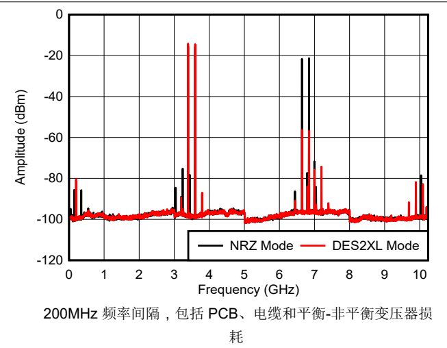
图 6-35. 双音， f_{\text{OUT}} = 3497\text{MHz} ，0dBFS
