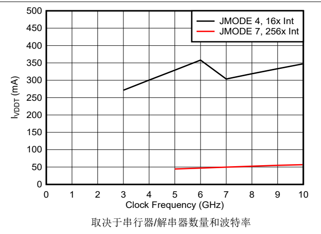
图 6-53. VDDT 电流与时钟频率和接口模式间的关系
