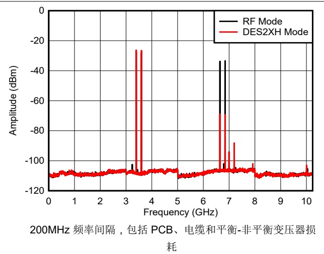
图 6-37. 双音， f_{\text{OUT}} = 3497\text{MHz} ， -12\text{dBFS}
