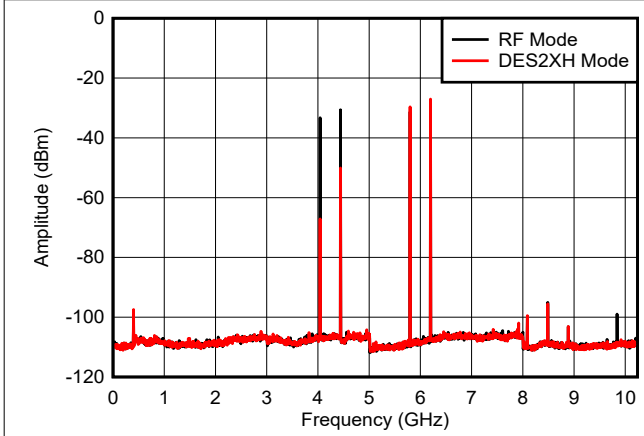
400MHz 频率间隔，包括 PCB、电缆和平衡-非平衡变压器损耗
