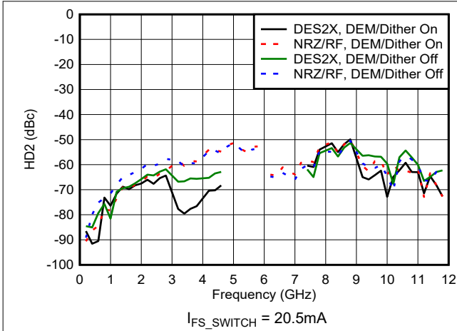
图 6-86. HD2 与频率和模式间的关系
