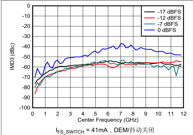
图 6-112. NRZ/RF 模式下 IMD3 与频率和数字振幅间的关系
