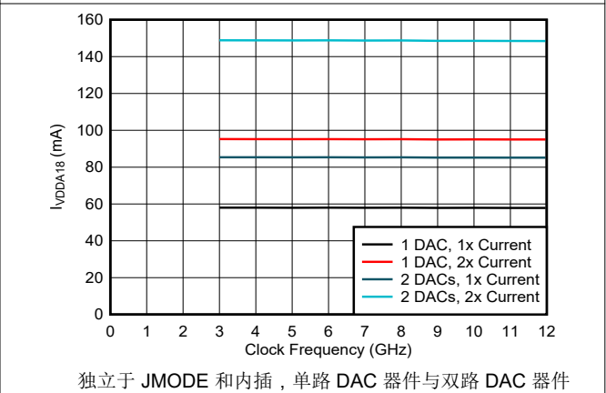
图 6-208. V_{DDA18} 电流与时钟频率和 DAC 模式间的关系
