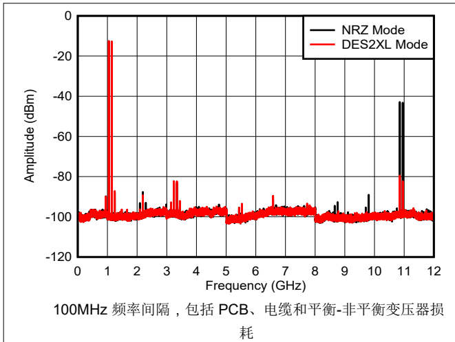
图 6-43. 双音， f_{\text{OUT}} = 1097\text{MHz} ，0dBFS
