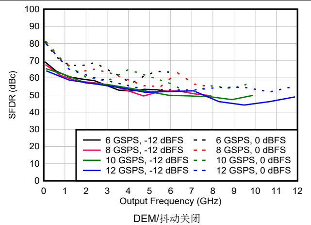
图 6-103. NRZ/RF 模式下 SFDR 与频率和采样速率间的关系
