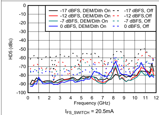
图 6-178. NRZ/RF 模式下 HD5 与频率和数字振幅间的关系
