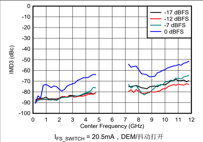
图 6-115. DES2X 模式下 IMD3 与频率和数字振幅间的关系
