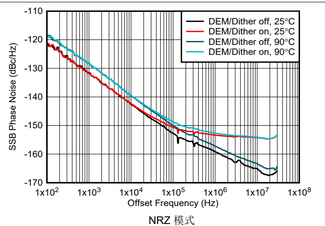
图 6-196. 1GHz 条件下相位噪声与偏移频率间的关系
