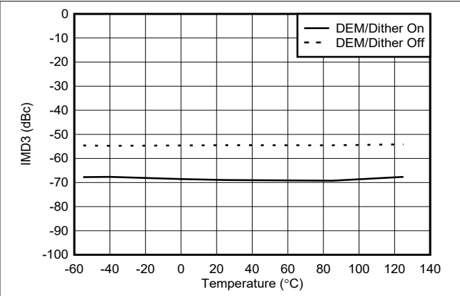
图 6-129. 9002MHz DES2XH 模式下 IMD3 与温度间的关系
