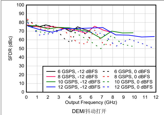
图 6-104. DES2X 模式下 SFDR 与频率和采样速率间的关系
