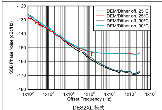
图 6-197. 1GHz 条件下相位噪声与偏移频率间的关系
