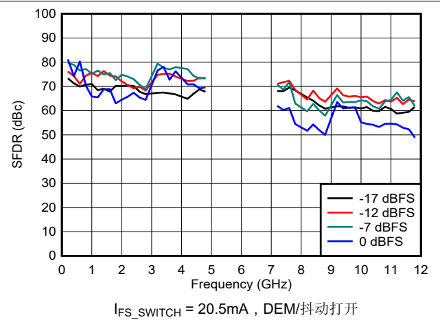
图 6-99. DES2X 模式下 SFDR 与频率和数字振幅间的关系
