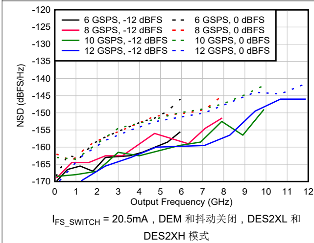
图 6-74. NSD 与输出频率和采样速率间的关系
