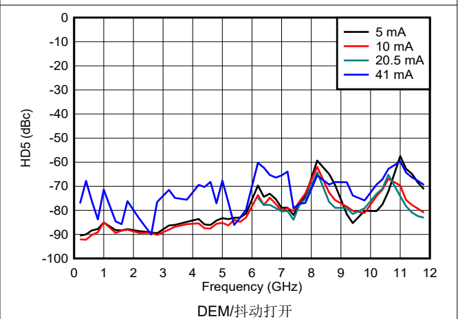
图 6-175. NRZ/RF 模式下 HD5 与频率和输出电流间的关系
