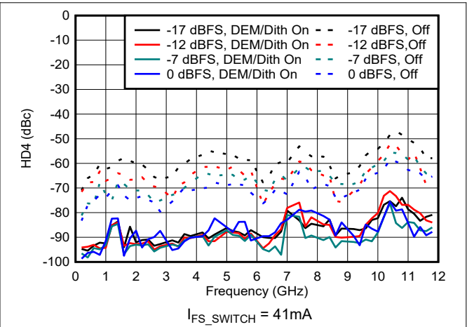
图 6-171. NRZ/RF 模式下 HD4 与频率和数字振幅间的关系
