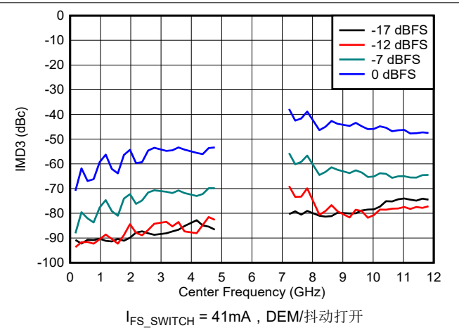
图 6-117. DES2X 模式下 IMD3 与频率和数字振幅间的关系
