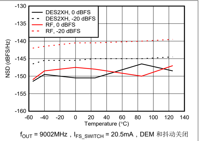
图 6-77. NSD 与温度间的关系
