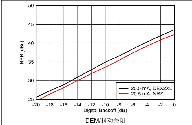
图 6-189. 噪声功率比与数字退避：第二个奈奎斯特区域
