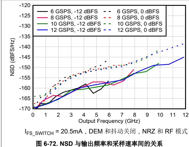
图 6-72. NSD 与输出频率和采样速率间的关系
