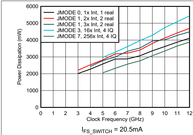
图 6-203. 功率损耗与时钟频率和数字模式间的关系
