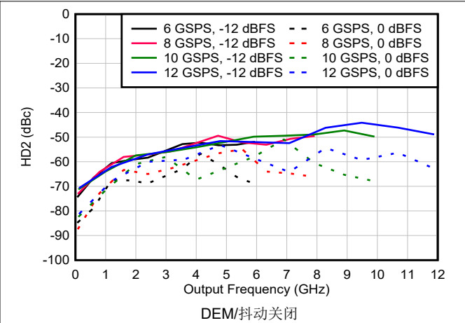
图 6-147. NRZ/RF 模式下 HD2 与频率和采样速率间的关系
