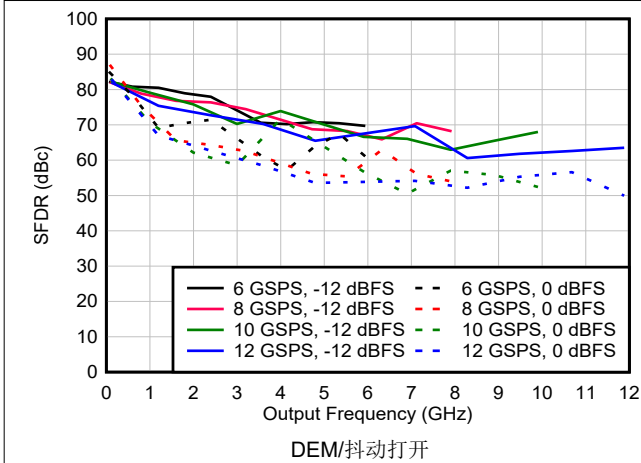
图 6-102. NRZ/RF 模式下 SFDR 与频率和采样速率间的关系
