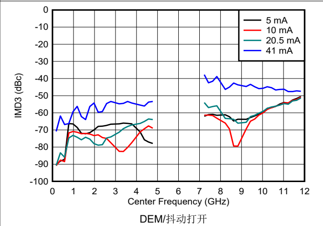
图 6-109. DES2X 模式下 IMD3 与频率和输出电流间的关系
