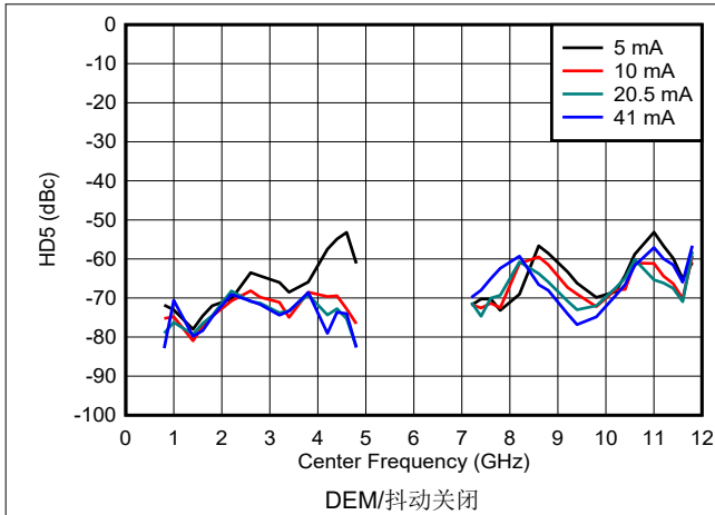
图 6-176. DES2X 模式下 HD5 与频率和输出电流间的关系
