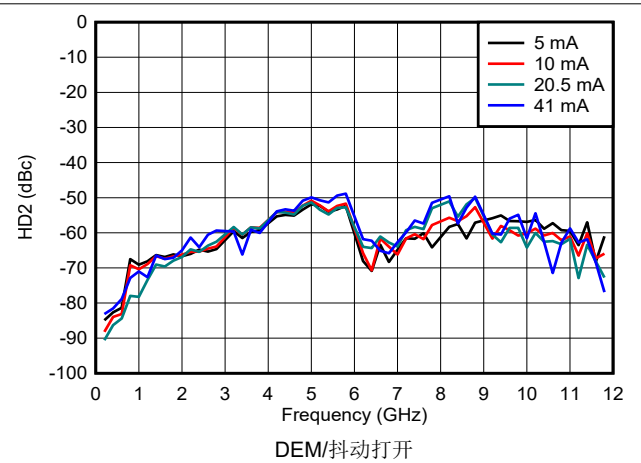
图 6-135. NRZ/RF 模式下 HD2 与频率和输出电流间的关系
