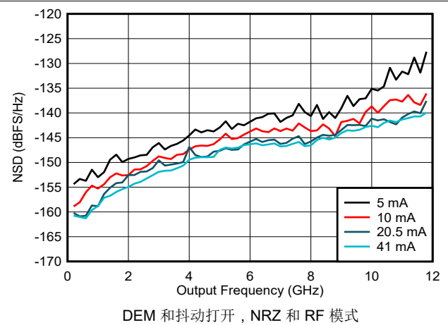
图 6-61. NSD 与输出频率和输出电流间的关系
