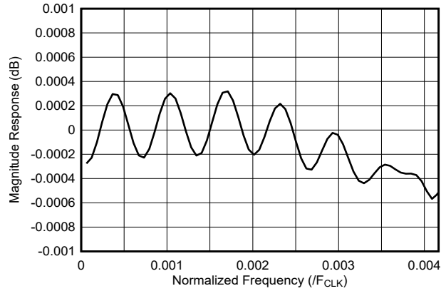
图 7-37. 96 倍内插滤波器通带响应
