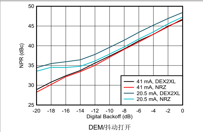
图 6-188. 噪声功率比与数字退避：第一奈奎斯特区域
