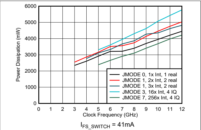
图 6-204. 功率损耗与时钟频率和数字模式间的关系
