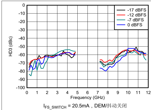
图 6-158. DES2X 模式下 HD3 与频率和数字振幅间的关系
