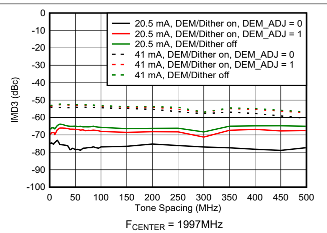
图 6-119. DES2XL 模式下 IMD3 与频率间隔间的关系
