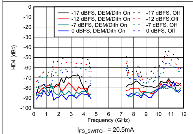
图 6-172. NRZ/RF 模式下 HD4 与频率和数字振幅间的关系
