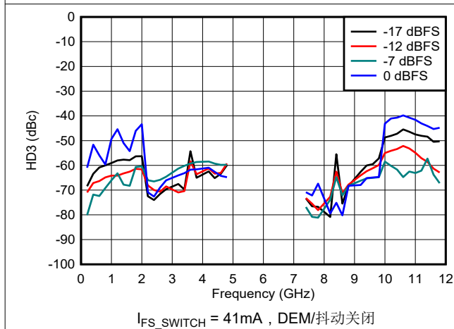
图 6-160. DES2X 模式下 HD3 与频率和数字振幅间的关系
