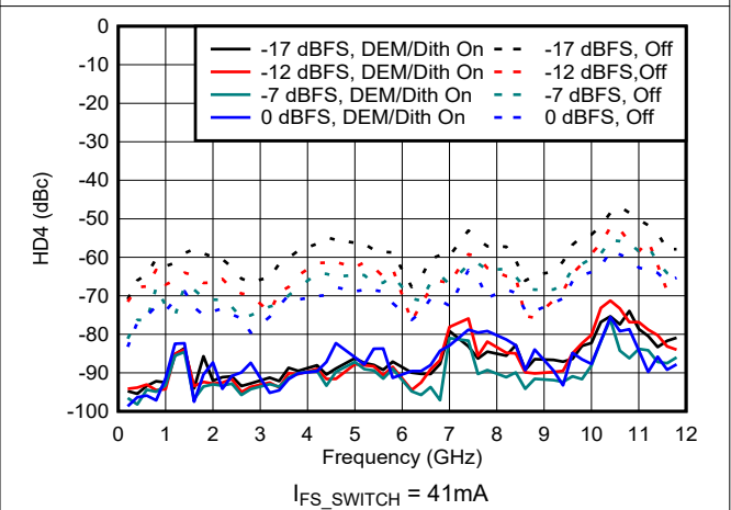
图 6-173. NRZ/RF 模式下 HD4 与频率和数字振幅间的关系
