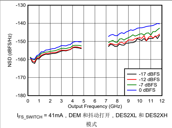
图 6-71. NSD 与输出频率和数字振幅间的关系
