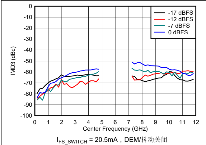
图 6-114. DES2X 模式下 IMD3 与频率和数字振幅间的关系
