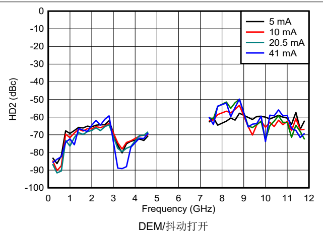
图 6-137. DES2X 模式下 HD2 与频率和输出电流间的关系
