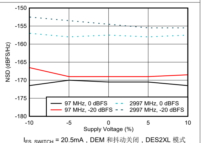
图 6-81. NSD 与电源电压间的关系
