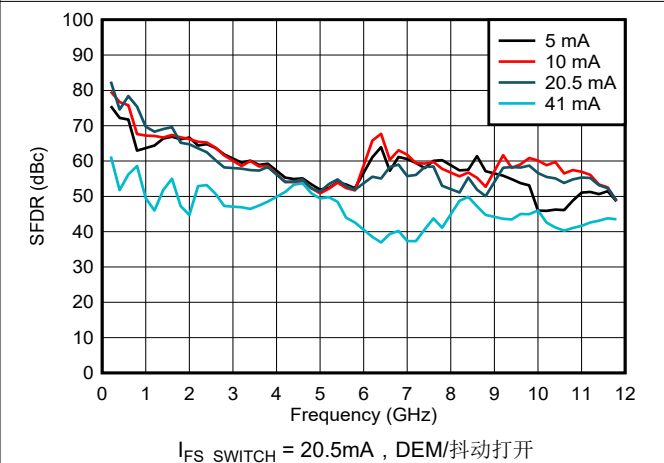
图 6-91. NRZ/RF 模式下 SFDR 与频率和输出电流间的关系
