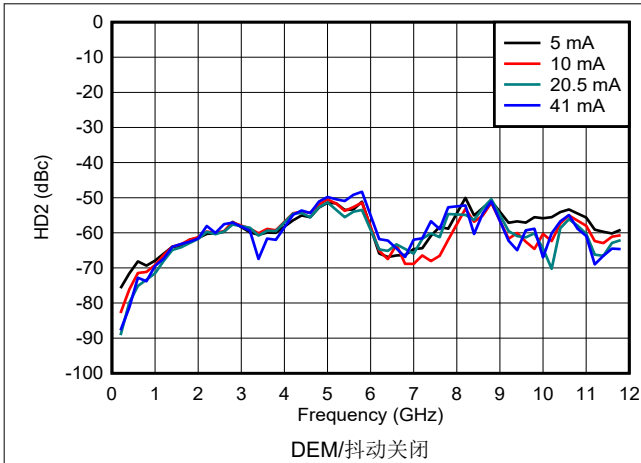
图 6-134. NRZ/RF 模式下 HD2 与频率和输出电流间的关系
