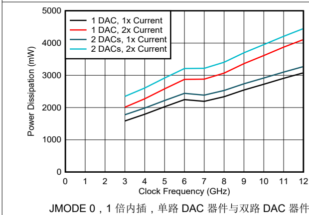
图 6-207. 功率损耗与时钟频率以及 DAC 模式间的关系
