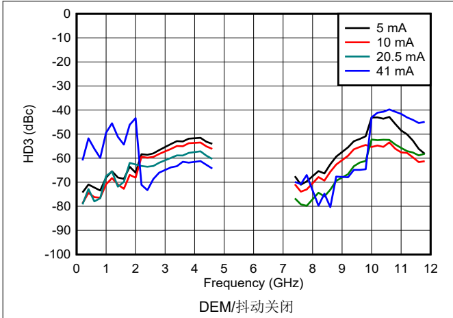
图 6-152. DES2X 模式下 HD3 与频率和输出电流间的关系
