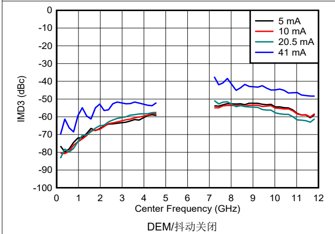
图 6-108. DES2X 模式下 IMD3 与频率和输出电流间的关系
