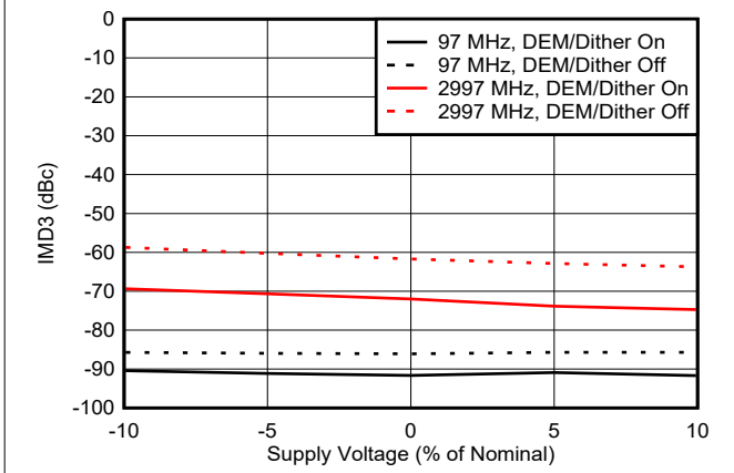
图 6-130. NRZ 模式下 IMD3 与电压间的关系
