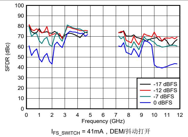
图 6-101. DES2X 模式下 SFDR 与频率和数字振幅间的关系
