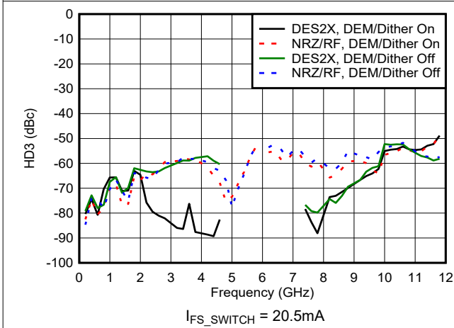
图 6-88. HD3 与频率和模式间的关系
