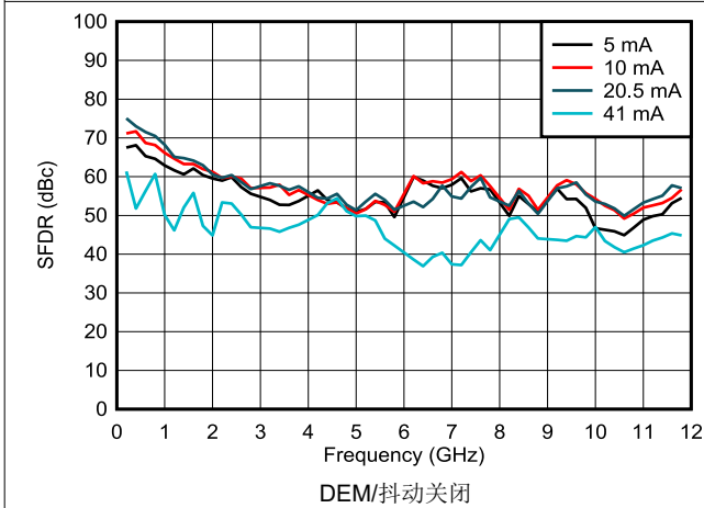
图 6-90. NRZ/RF 模式下 SFDR 与频率和输出电流间的关系
