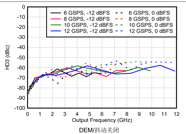
图 6-163. NRZ/RF 模式下 HD3 与频率和采样速率间的关系
