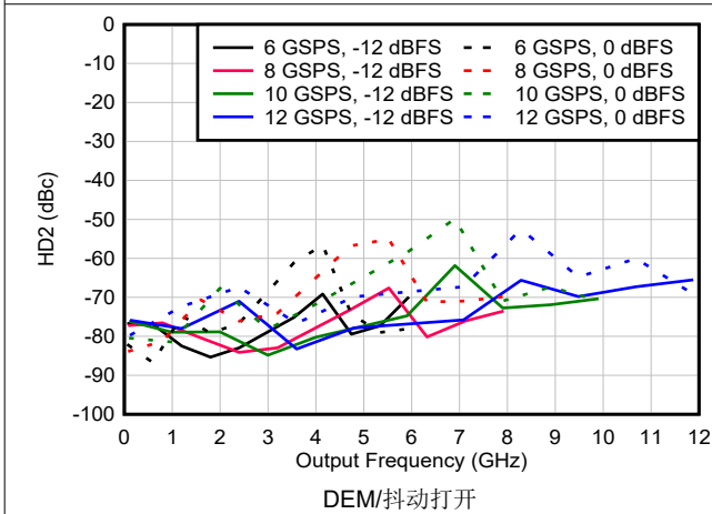
图 6-148. DES2X 模式下 HD2 与频率和采样速率间的关系
