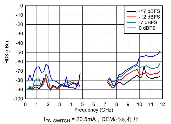
图 6-159. DES2X 模式下 HD3 与频率和数字振幅间的关系
