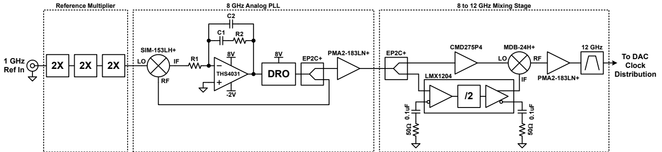
图 8-11. 12GHz 时钟合成器
