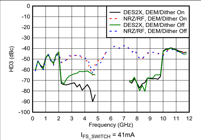
图 6-89. HD3 与频率和模式间的关系
