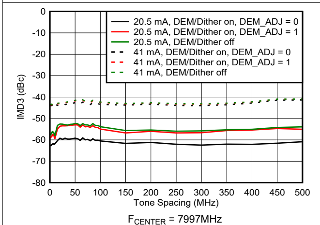
图 6-120. RF 模式下 IMD3 与频率间隔间的关系
