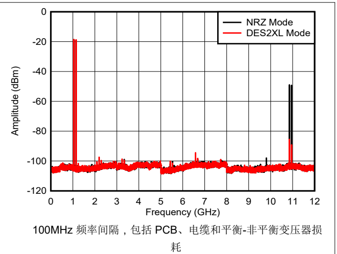
图 6-44. 双音， f_{\text{OUT}} = 1097\text{MHz} ，-6dBFS
