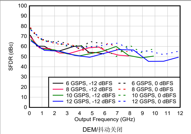
图 6-105. DES2X 模式下 SFDR 与频率和采样速率间的关系
