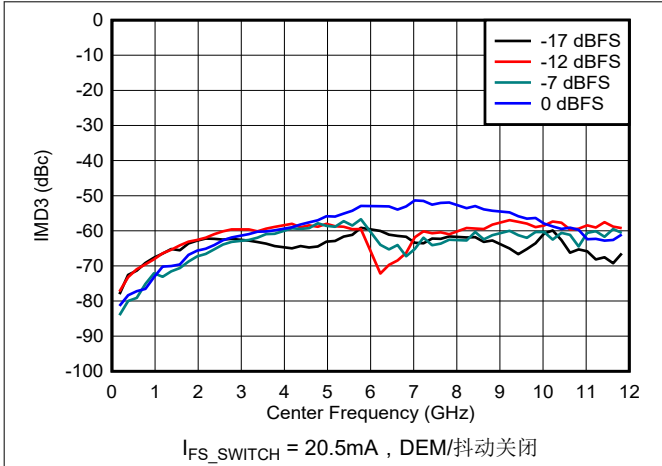
图 6-110. NRZ/RF 模式下 IMD3 与频率和数字振幅间的关系
