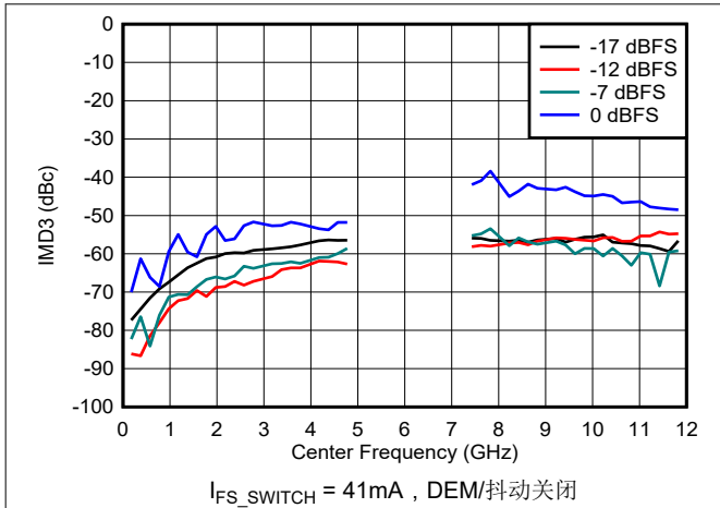
图 6-116. DES2X 模式下 IMD3 与频率和数字振幅间的关系
