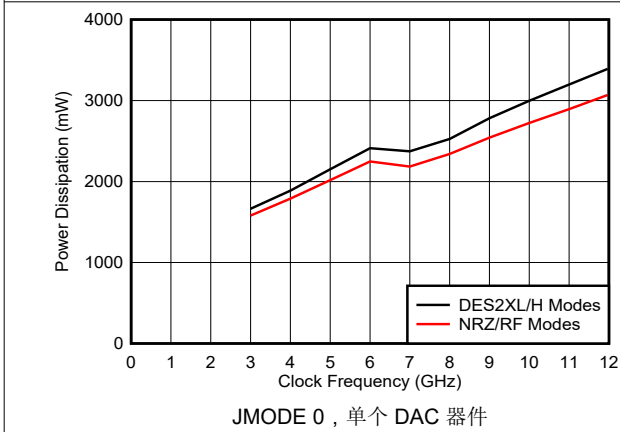
图 6-205. 功率损耗与时钟频率以及 DAC 模式间的关系
