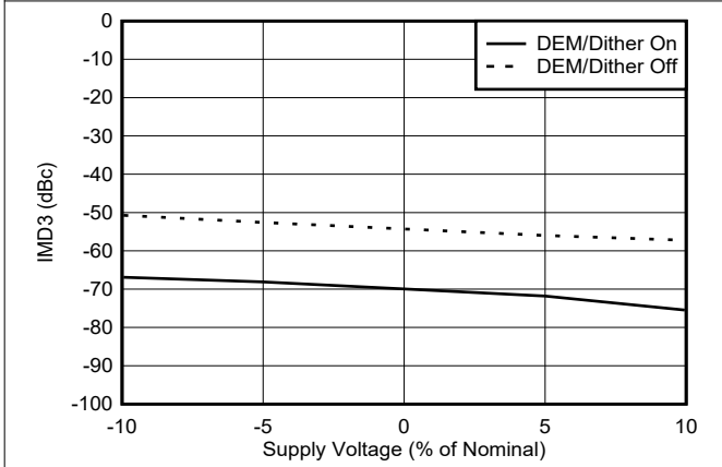
图 6-132. 9002MHz RF 模式下 IMD3 与电压间的关系
