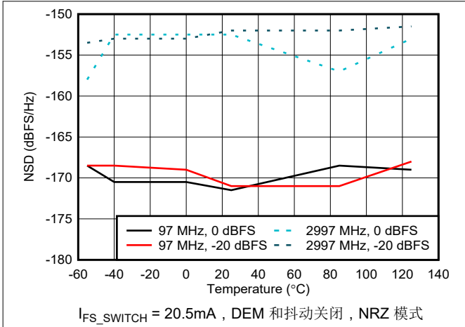
图 6-76. NSD 与温度间的关系
