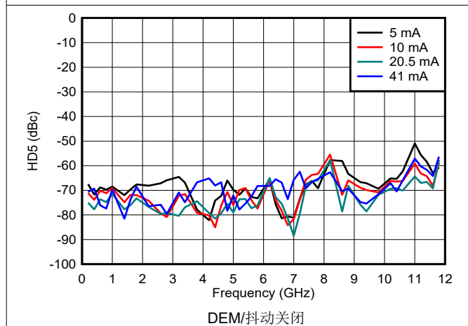
图 6-174. NRZ/RF 模式下 HD5 与频率和输出电流间的关系
