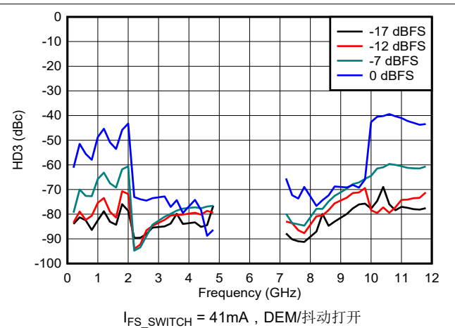
图 6-161. DES2X 模式下 HD3 与频率和数字振幅间的关系
