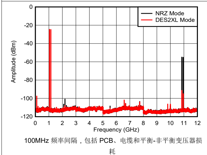
图 6-45. 双音， f_{\text{OUT}} = 1097\text{MHz} ，-12dBFS
