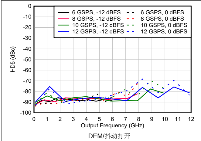
图 6-182. NRZ/RF 模式下 HD5 与频率和采样速率间的关系
