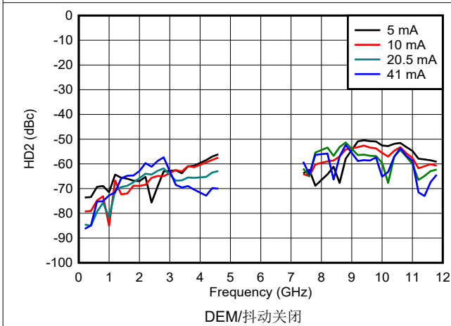
图 6-136. DES2X 模式下 HD2 与频率和输出电流间的关系
