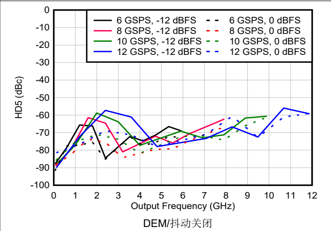
图 6-185. DES2X 模式下 HD5 与频率和采样速率间的关系
