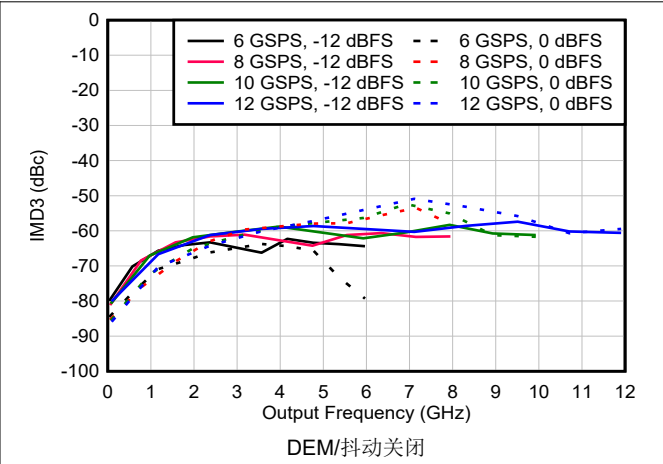
图 6-123. NRZ/RF 模式下 IMD3 与频率和采样速率间的关系
