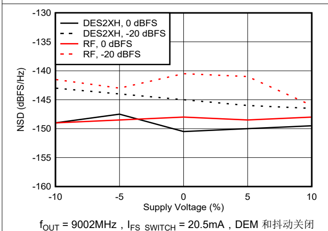
图 6-80. NSD 与电源电压间的关系
