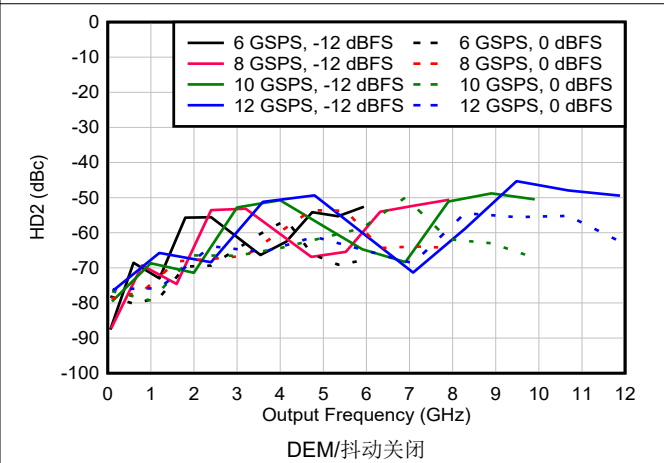
图 6-149. DES2X 模式下 HD2 与频率和采样速率间的关系
