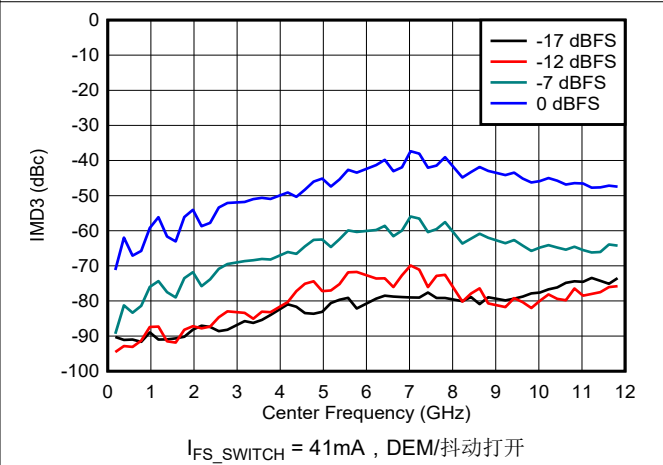
图 6-113. NRZ/RF 模式下 IMD3 与频率和数字振幅间的关系
