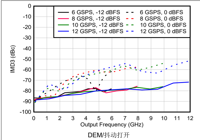
图 6-122. NRZ/RF 模式下 IMD3 与频率和采样速率间的关系
