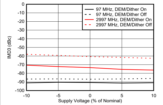
图 6-131. DES2XL 模式下 IMD3 与电压间的关系
