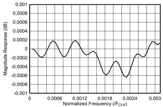
图 7-39. 128 倍内插滤波器通带响应
