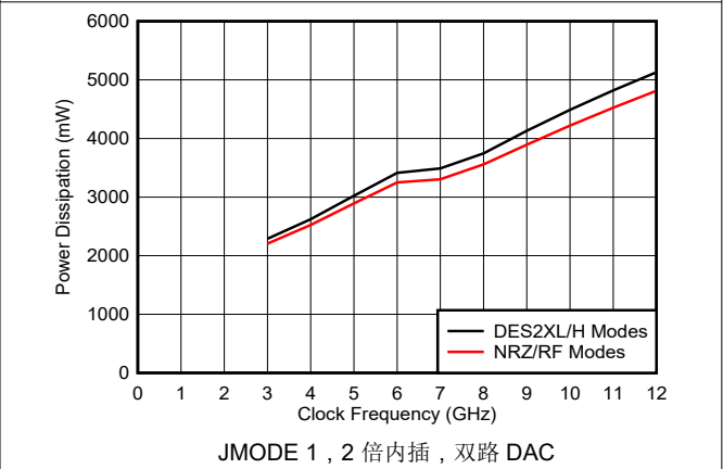
图 6-206. 功率损耗与时钟频率以及 DAC 模式间的关系
