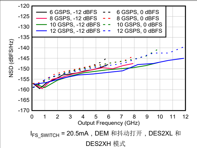
图 6-75. NSD 与输出频率和采样速率间的关系
