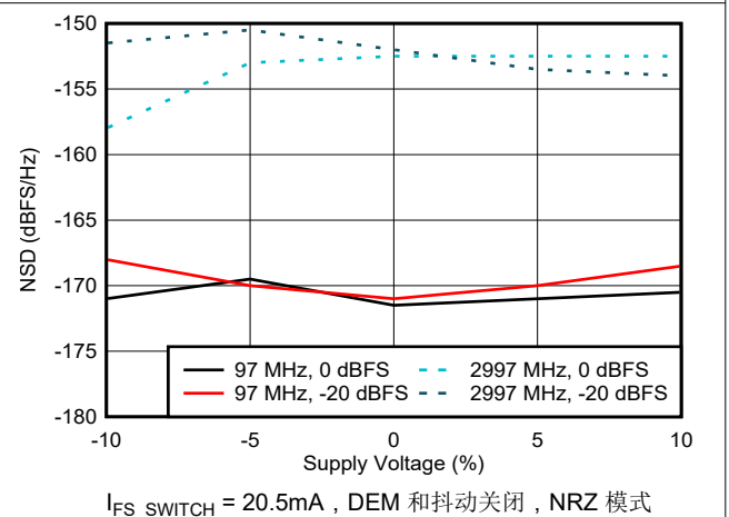
图 6-79. NSD 与电源电压间的关系
