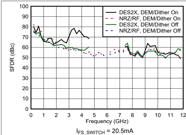
图 6-82. SFDR 与频率和模式间的关系
