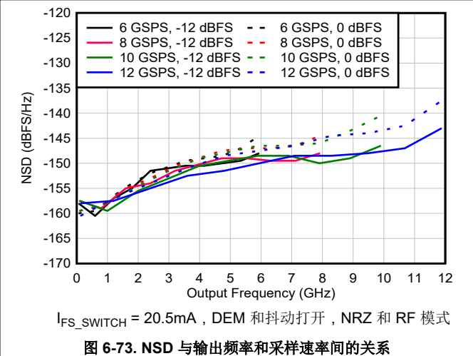
图 6-73. NSD 与输出频率和采样速率间的关系
