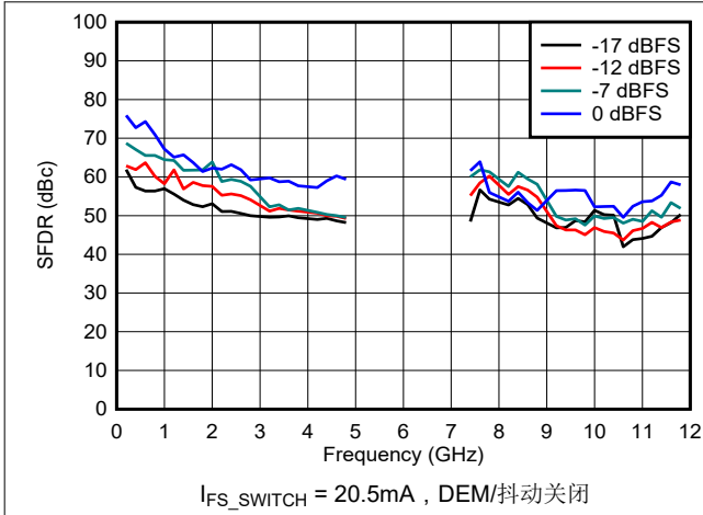
图 6-98. DES2X 模式下 SFDR 与频率和数字振幅间的关系
