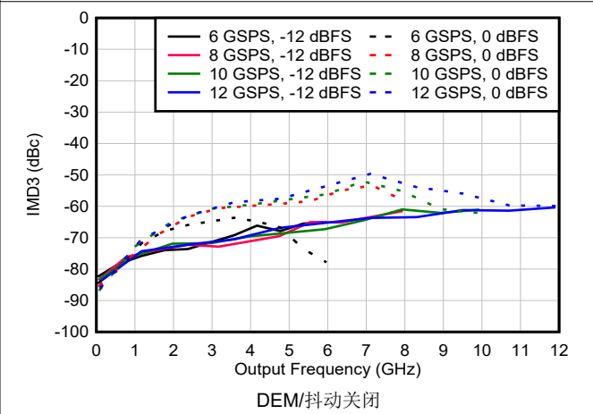
图 6-125. DES2X 模式下 IMD3 与频率和采样速率间的关系
