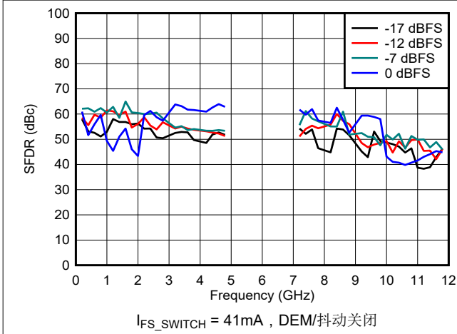
图 6-100. DES2X 模式下 SFDR 与频率和数字振幅间的关系
