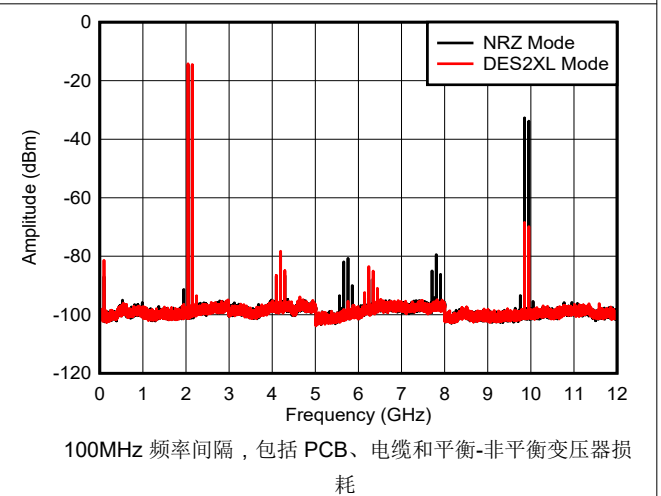
图 6-46. 双音， f_{\text{OUT}} = 2097\text{MHz} ，0dBFS
