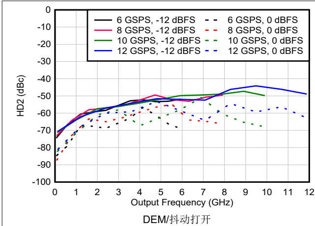
图 6-146. NRZ/RF 模式下 HD2 与频率和采样速率间的关系
