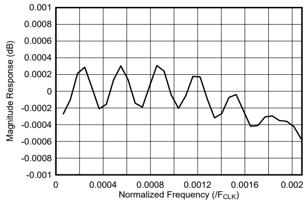
图 7-41. 192 倍内插滤波器通带响应
