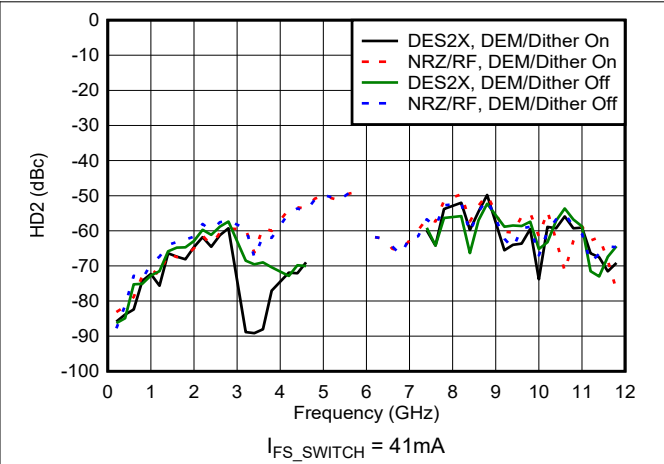
图 6-87. HD2 与频率和模式间的关系
