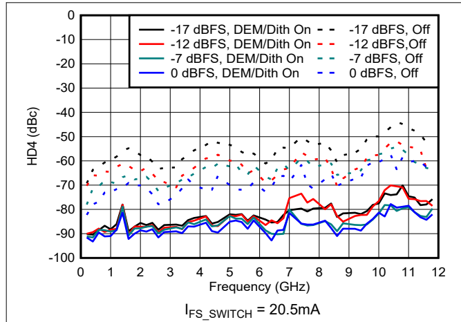
图 6-170. NRZ/RF 模式下 HD4 与频率和数字振幅间的关系
