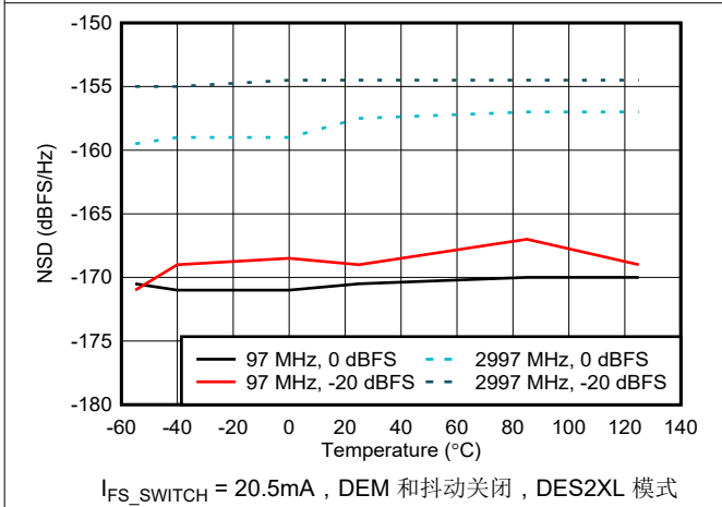
图 6-78. NSD 与温度间的关系
