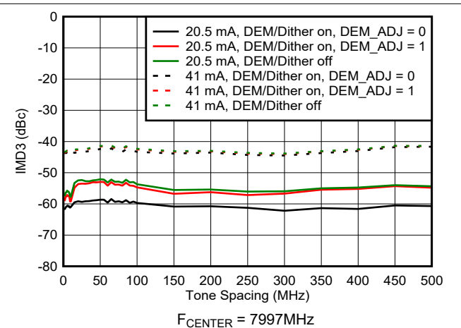
图 6-121. DES2XH 模式下 IMD3 与频率间隔间的关系
