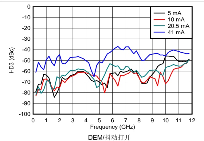
图 6-151. NRZ/RF 模式下 HD3 与频率和输出电流间的关系
