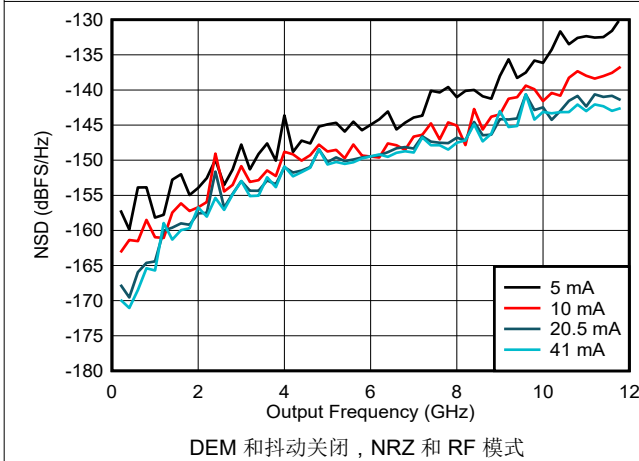
图 6-60. NSD 与输出频率和输出电流间的关系
