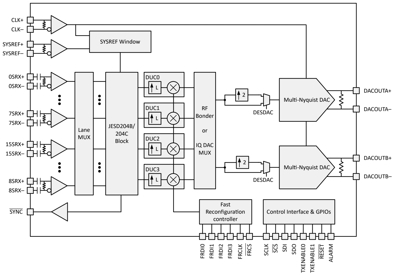
图 7-1. 双通道器件
