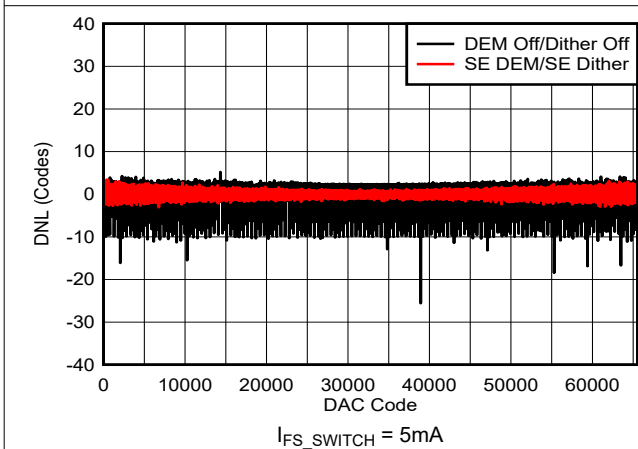
图 6-12. DNL 与 DAC 代码间的关系：5mA
