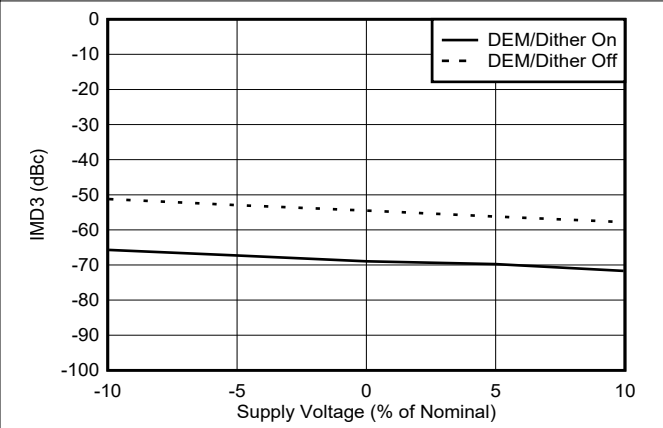
图 6-133. 9002MHz DES2XH 模式下 IMD3 与电压间的关系
