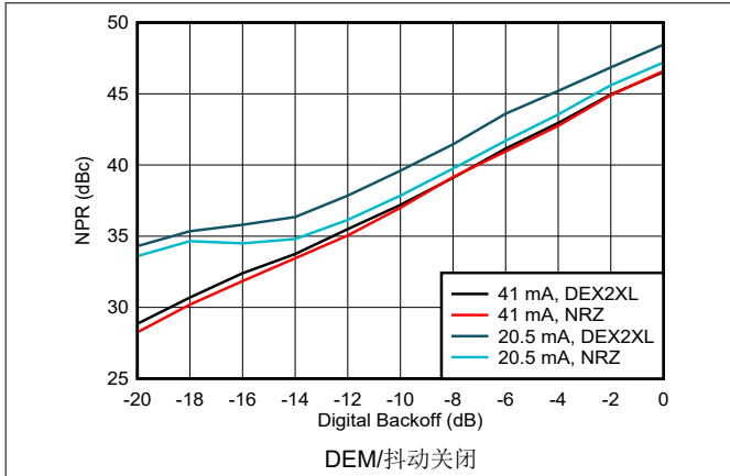
图 6-187. 噪声功率比与数字退避：第一奈奎斯特区域
