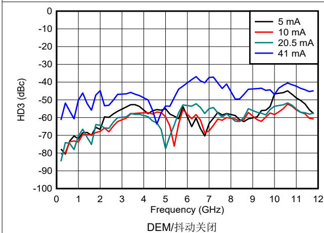
图 6-150. NRZ/RF 模式下 HD3 与频率和输出电流间的关系
