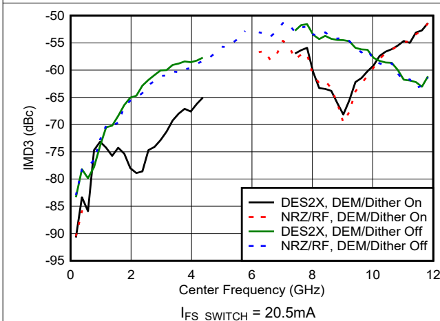
图 6-84. IMD3 与频率和模式间的关系
