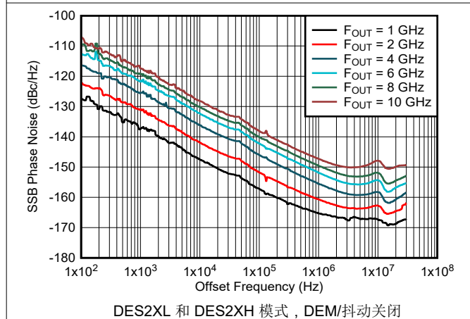
图 6-195. 相位噪声与偏移频率和输出频率间的关系
