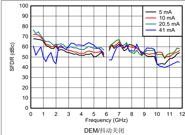
图 6-92. DES2X 模式下 SFDR 与频率和输出电流间的关系
