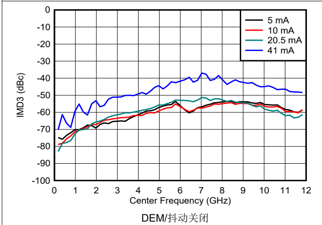
图 6-106. NRZ/RF 模式下 IMD3 与频率和输出电流间的关系
