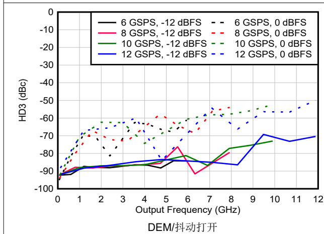
图 6-162. NRZ/RF 模式下 HD3 与频率和采样速率间的关系
