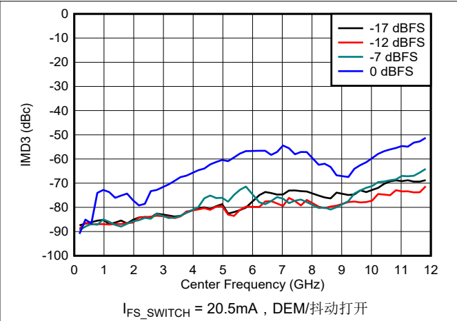
图 6-111. NRZ/RF 模式下 IMD3 与频率和数字振幅间的关系
