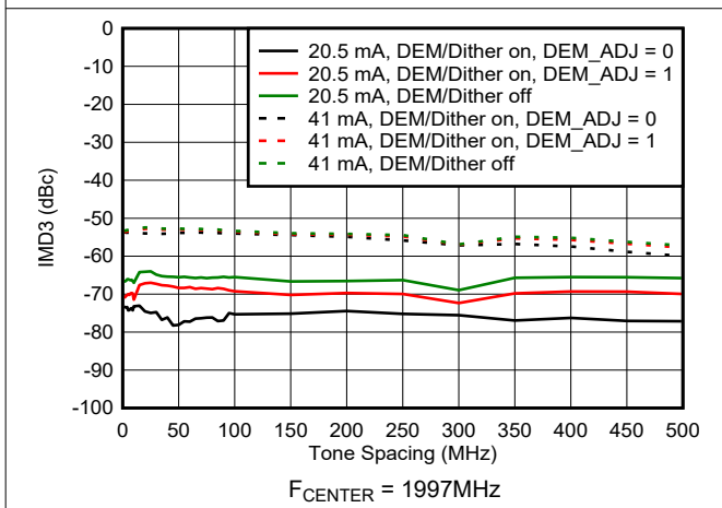
图 6-118. NRZ 模式下 IMD3 与频率间隔间的关系
