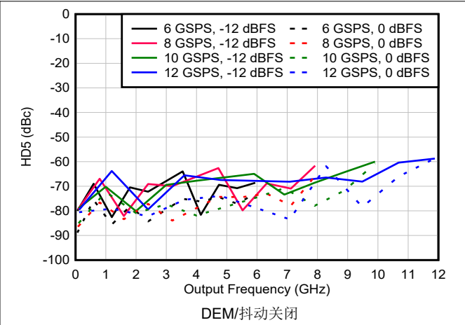
图 6-183. NRZ/RF 模式下 HD5 与频率和采样速率间的关系
