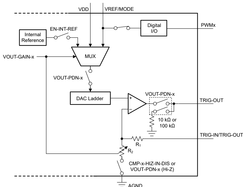
图 7-2. 电压基准选择与断电逻辑
