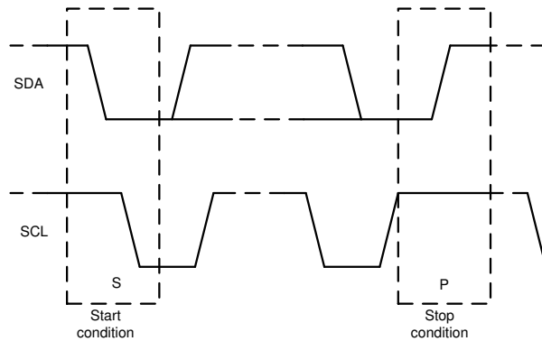
图 7-16. 启动和停止条件
