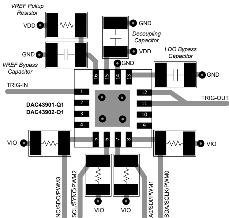
图 8-4. 布局示例
