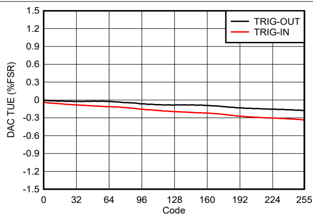
图 6-4. DAC TUE 与数字输入代码间的关系
