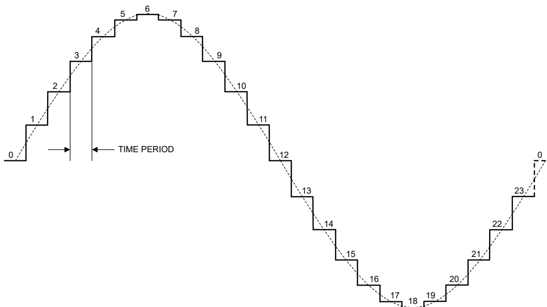
图 7-14. 正弦波生成
