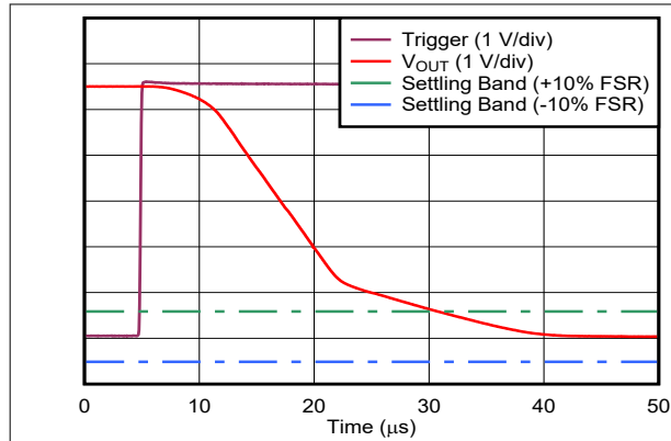
图 6-22. 电压输出建立时间 - 下降沿
