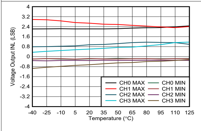
图 6-6. 电压输出 INL 与温度间的关系
