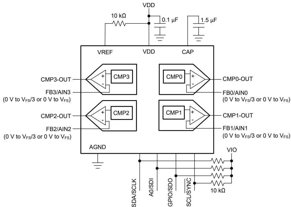
图 7-3. 比较器接口
