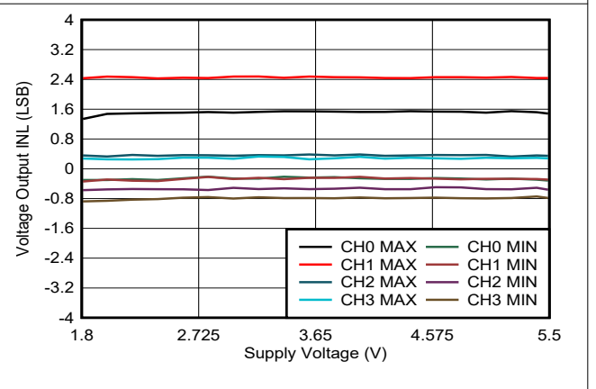
图 6-7. 电压输出 INL 与电源电压间的关系
