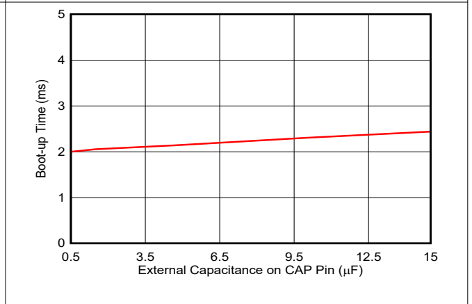
图 6-57. 启动时间与 CAP 引脚上电容间的关系
