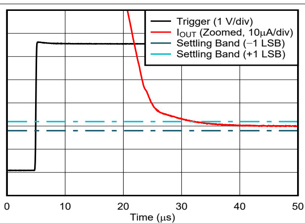
图 6-44. 电流输出建立时间 (下降沿)
