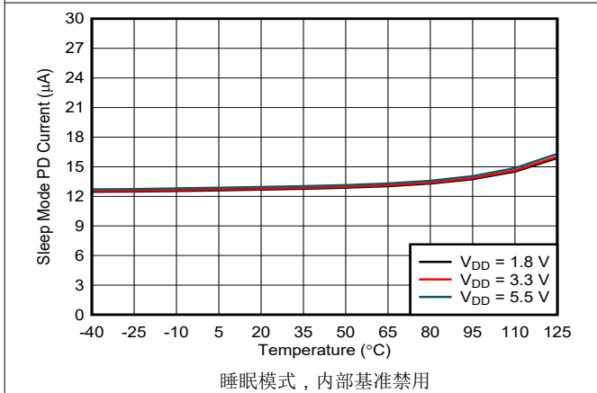
图 6-56. 断电电流与温度间的关系
