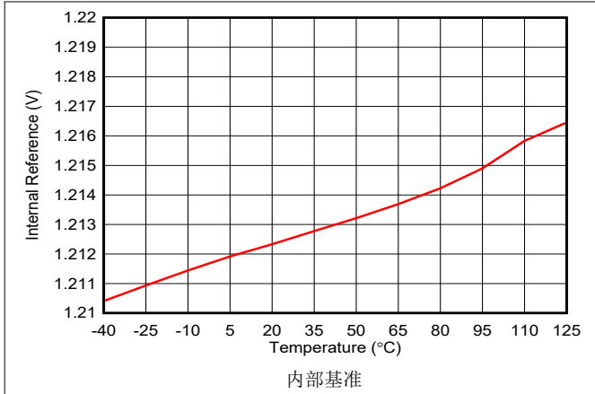
图 6-54. 内部基准与温度间的关系
