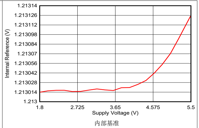
图 6-55. 内部基准与电源电压间的关系
