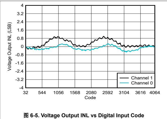
图 6-5. Voltage Output INL vs Digital Input Code
