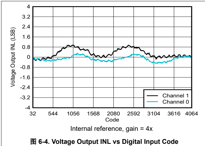
图 6-4. Voltage Output INL vs Digital Input Code
