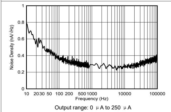
图 6-52. Current Output Noise Density
