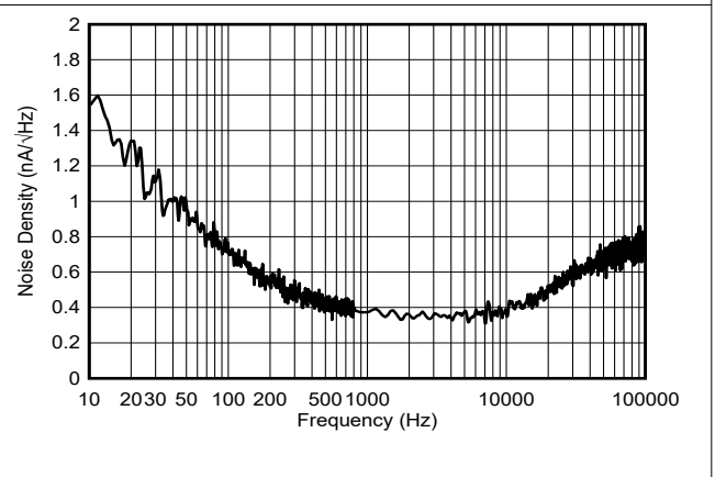
图 6-53. Current Output Noise Density
